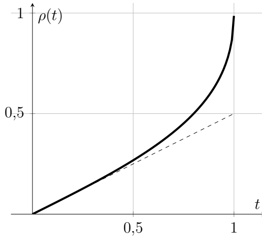
Figura 5.1: Gráfica de la función \rho
