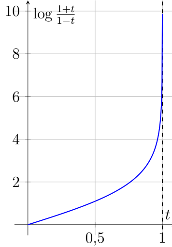
Figura 3.2: Gráfica de f(t) = \log \frac{1+t}{1-t} en [0, 1) .
