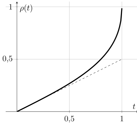
Figura 5.1: Gráfica de la función \rho
