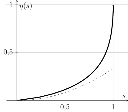
Figura 5.3: Gráfica de la función \eta
