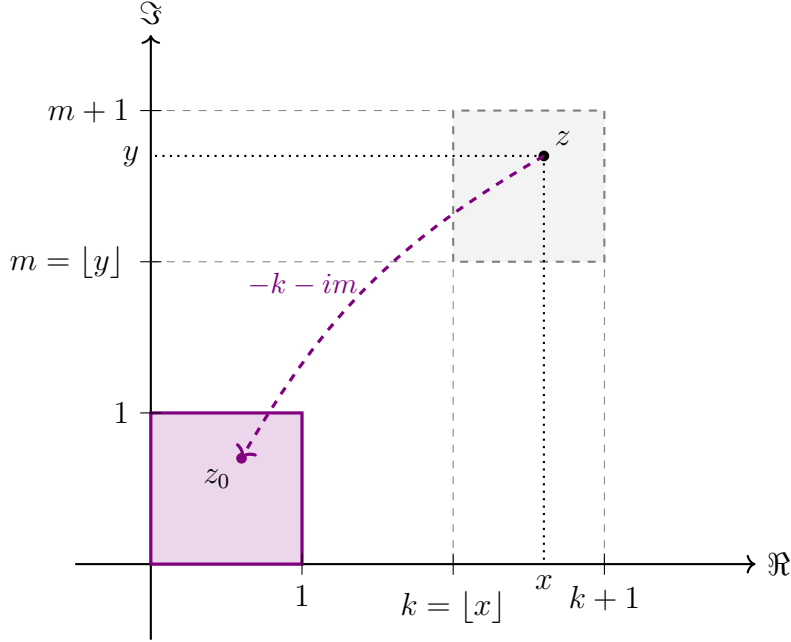
Figura H.2: Reducción de un punto z = x + iy al dominio fundamental K .
