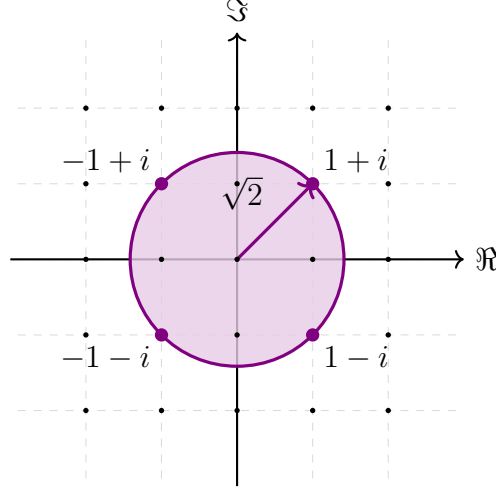
Figura H.1: Retícula de puntos E y el disco máximo de centro el origen libre de ellos.
