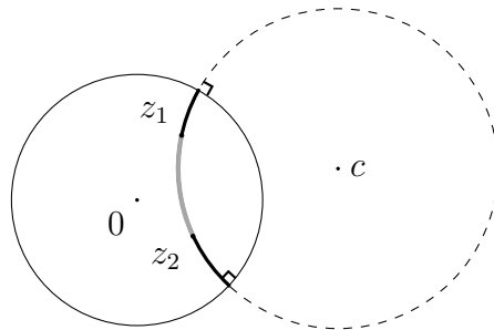
Figura 3.3: Recta hiperbólica que pasa por z_1 y z_2 .
