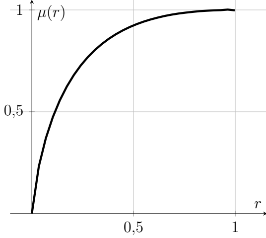
Figura 5.2: Gráfica de la función \mu
