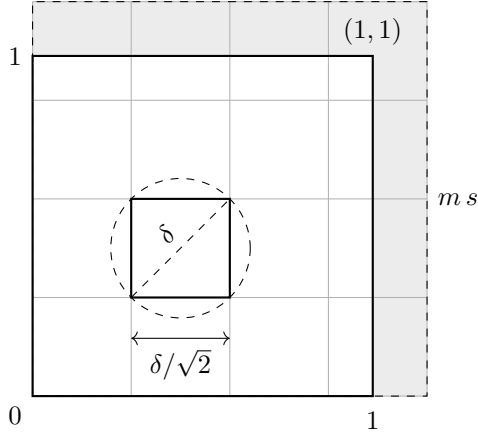
Figura H.1: Cubrimiento del cuadrado unidad Q_{(1,1)} \subset \mathbb{R}^2 (blanco) mediante una rejilla de m \times m subcuadrados de lado s = \delta/\sqrt{2} (y, por tanto, diámetro s\sqrt{2} \leq \delta ), con m = \lceil \sqrt{2}/\delta \rceil .
