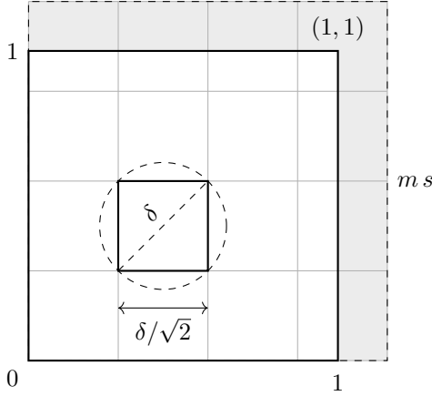
Figura H.2: Cubrimiento del cuadrado unidad Q_{(1,1)} \subset \mathbb{R}^2 (blanco) mediante una rejilla de m \times m subcuadrados de lado s = \delta/\sqrt{2} (y, por tanto, diámetro s\sqrt{2} \leq \delta ), con m = \lceil \sqrt{2}/\delta \rceil .
