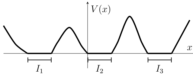
Figura H.1: Potencial que se anula en los intervalos I_1, I_2, I_3 .
