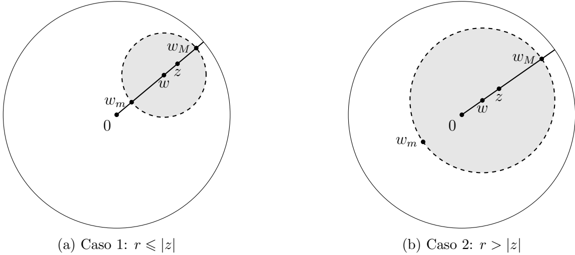
Figure 2.1: Borde de \mathbb{D} , segmento radial en dirección z/|z| , y B_\rho(z, r) = \tau_z(D(0, r)) con centro w y radio s ; se señalan w_m y w_M .
