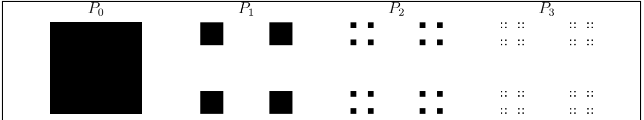
Figura 1.5: Primeros cuatro órdenes en la construcción del polvo de Cantor.
