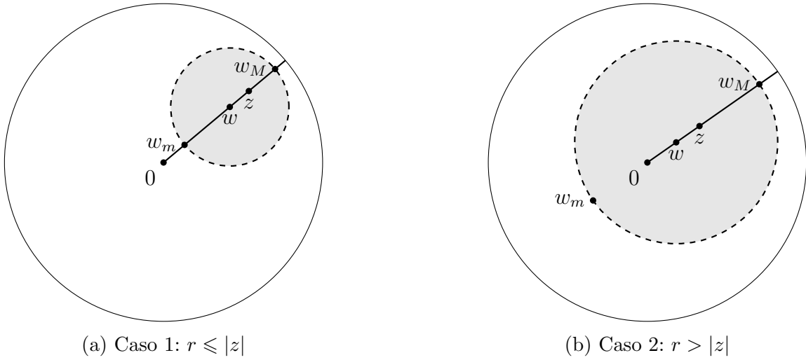
Figura 2.1: Borde de \mathbb{D} , segmento radial en dirección z/|z| , y B_\rho(z, r) = \tau_z(D(0, r)) con centro w y radio s ; se señalan w_m y w_M .
