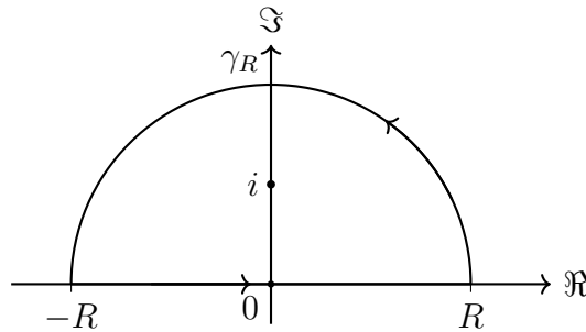
Figure 8.1: Camino \gamma_R en el semiplano superior y polo en i .
