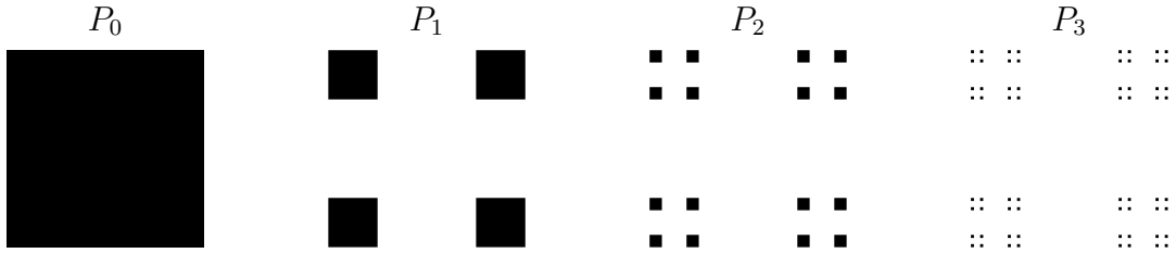
Figura 1.5: Primeros cuatro órdenes en la construcción del polvo de Cantor.
