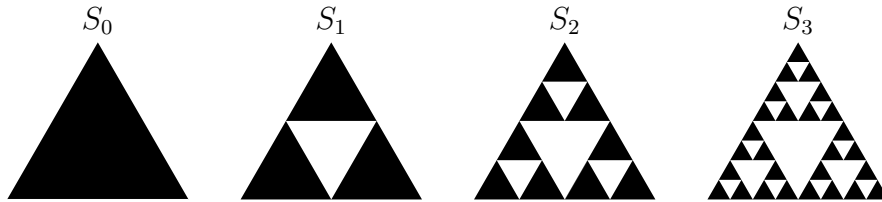
Figura 1.3: Primeros cuatro órdenes en la construcción del triángulo de Sierpinski.
