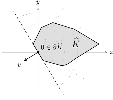
(a) Cuerpo convexo trasladado \hat{K} con su recta soporte L y red polar.
