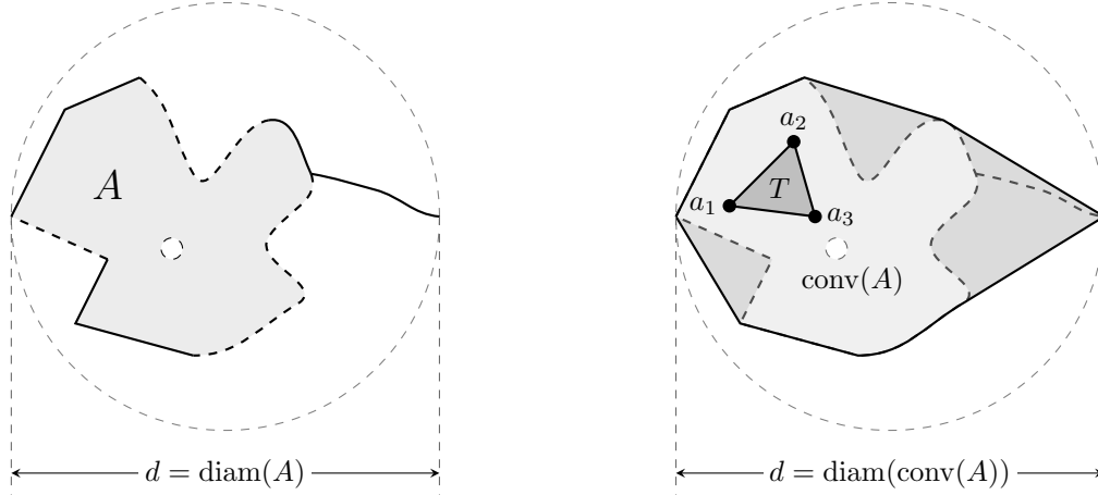
(a) Conjunto medible A \subset \mathbb{R}^2 con diámetro d = \text{diam}(A) marcado.
