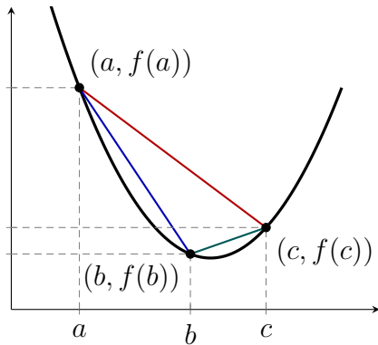
Figura 2.1: Representación gráfica de la proposición 2.2.14. La función f es convexa, y las pendientes de las secantes cumplen la desigualdad de la proposición.
