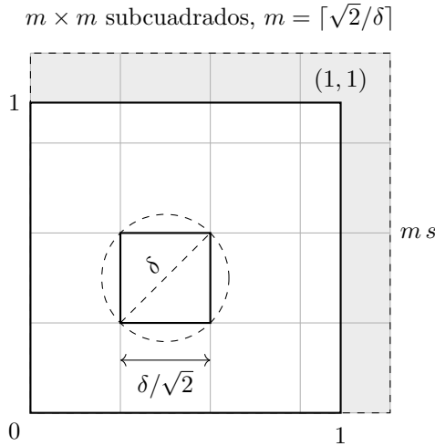
Figura E.1: Cubrimiento del cuadrado unidad Q_{(1,1)} \subset \mathbb{R}^2 (blanco) mediante una rejilla de m \times m subcuadrados de lado s = \delta/\sqrt{2} (y, por tanto, diámetro s\sqrt{2} \leq \delta ), con m = \lceil \sqrt{2}/\delta \rceil .
