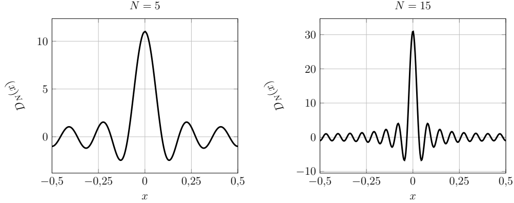
Figura 4.1: Gráficas del núcleo de Dirichlet para diferentes valores de N .
