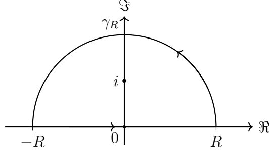
Figura 1.1: Camino \gamma_R en el semiplano superior y polo en i .
