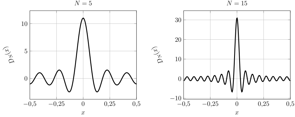
Figura 4.1: Gráficas del núcleo de Dirichlet para diferentes valores de N .
