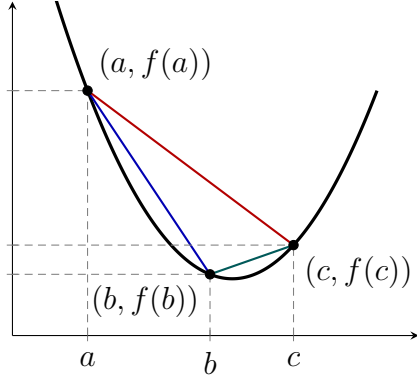
Figura 1.1: Representación gráfica de la proposición 1.6.2. La función f es convexa, y las pendientes de las secantes cumplen la desigualdad de la proposición.
