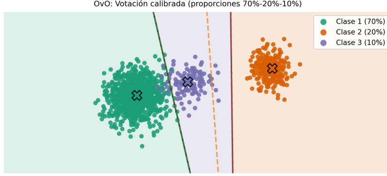
Figure 5.3: Dataset sintético desbalanceado y regiones de decisión con SVM lineal OvO.
