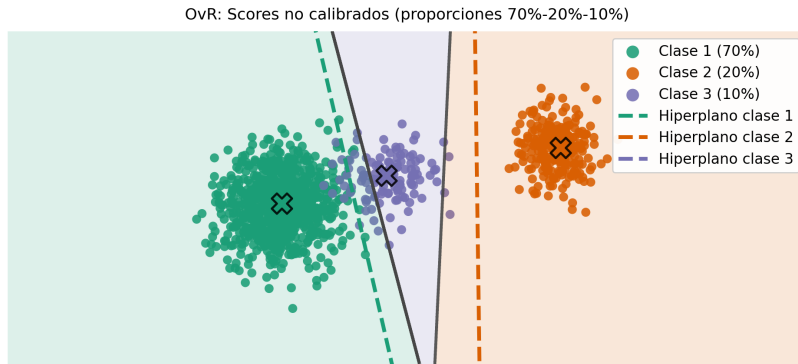
Figure 5.2: Dataset sintético desbalanceado y regiones de decisión con SVM lineal OvR.
