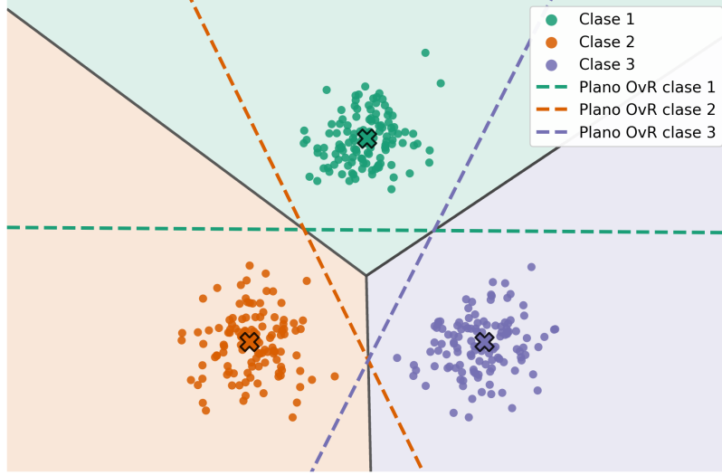
Figure 5.1: Nubes sintéticas en \mathbb{R}^2 y regiones de decisión de una SVM lineal OvR.
