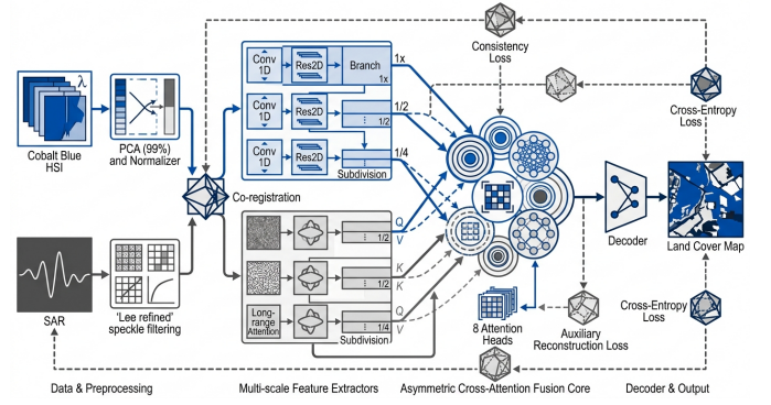
Fig. 2. Diagrama general de la arquitectura propuesta de fusión multimodal HSI-SAR.
