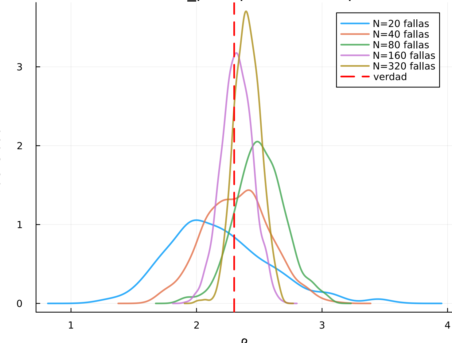
CONVERGENCIA — brake_pad: posterior de \beta al acumular fallas
