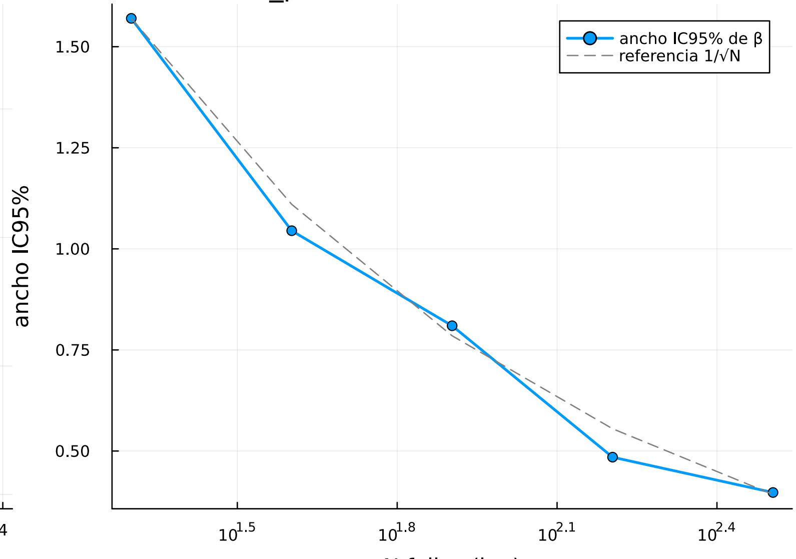
brake_pad — el IC se estrecha \propto 1/\sqrt{N}
