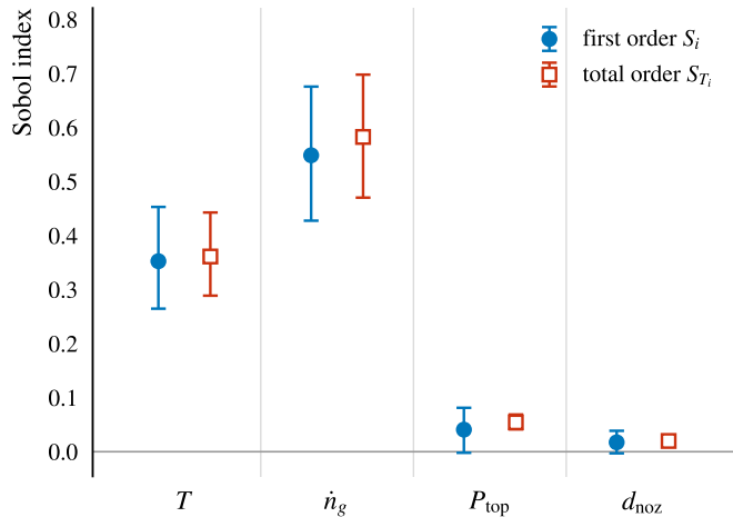
pessimistic (Calderoni K_s , D_l )
