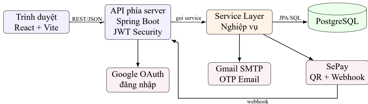
Hình 4.1: Kiến trúc tổng thể của hệ thống BlueMoon
