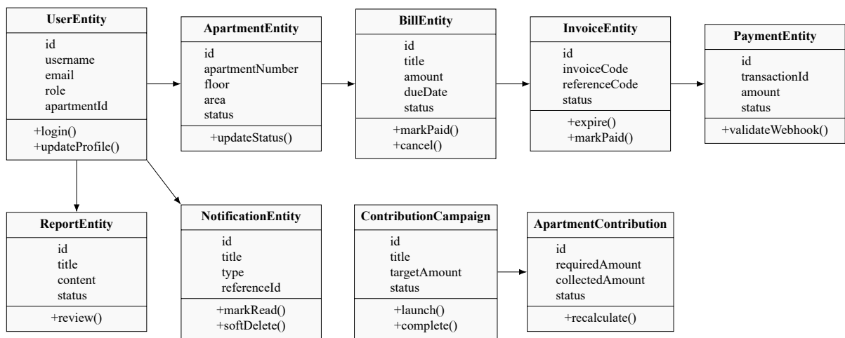
Hình 4.3: Sơ đồ lớp phân tích rút gọn
