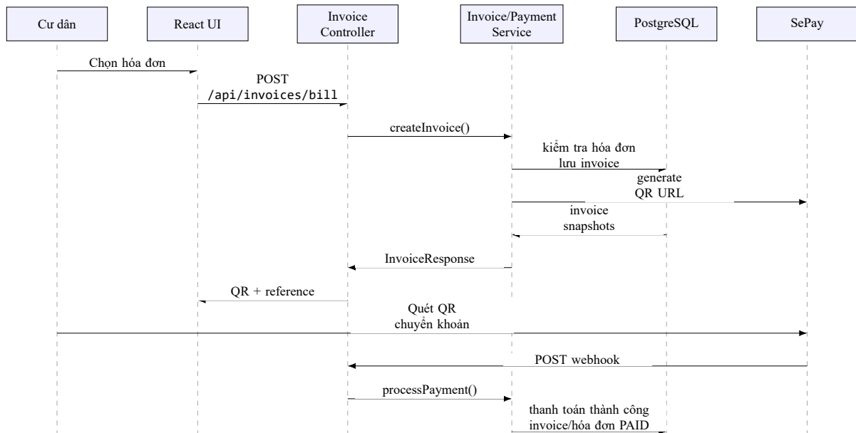
Hình 4.4: Sơ đồ tuần tự rút gọn cho luồng thanh toán hóa đơn
