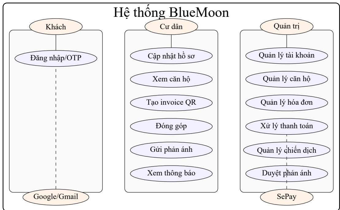
Hình 4.2: Sơ đồ Use Case tổng thể
