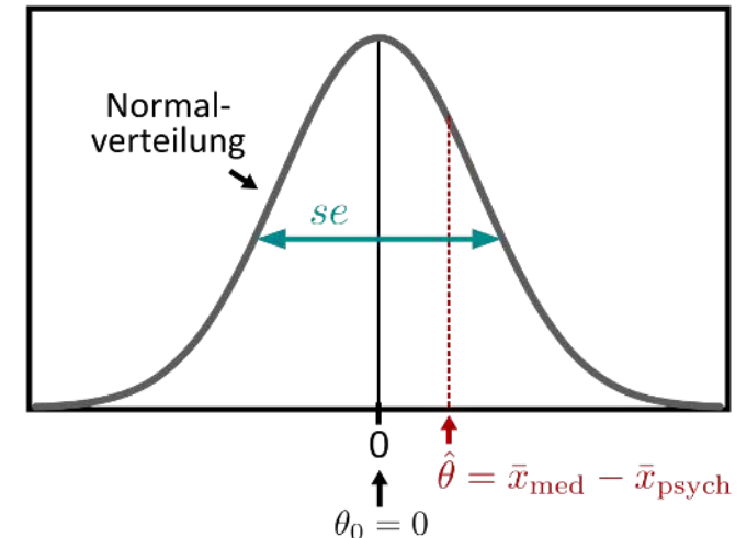
Theoretische Nullhypothesenverteilung
