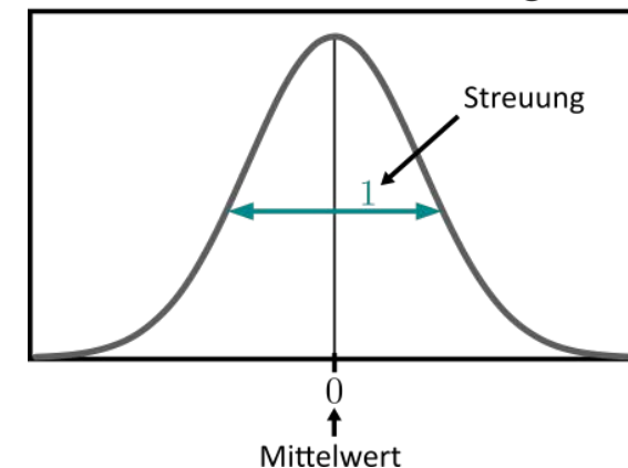
Standardnormalverteilung
