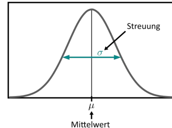
Unstandardisierte Normalverteilung
