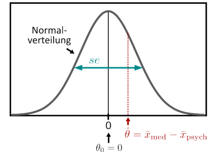
Theoretische Nullhypothesenverteilung
