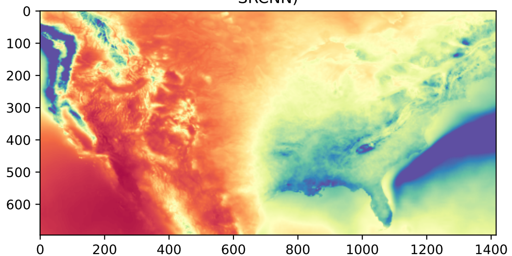
SRCNN)
