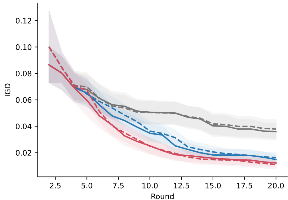
IGD convergence
