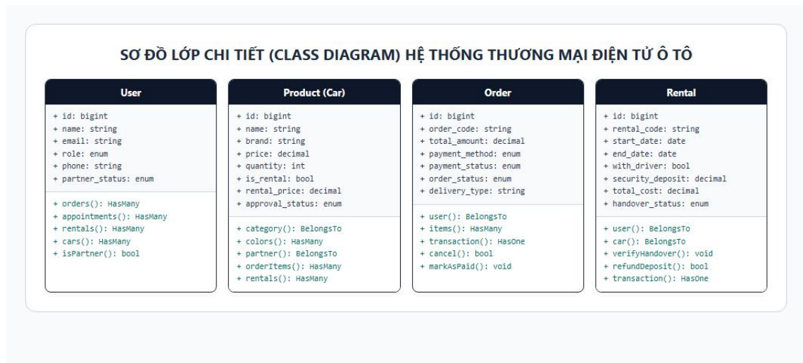
Hình 2.10: Sơ đồ lớp chi tiết của hệ thống thương mại điện tử ô tô
