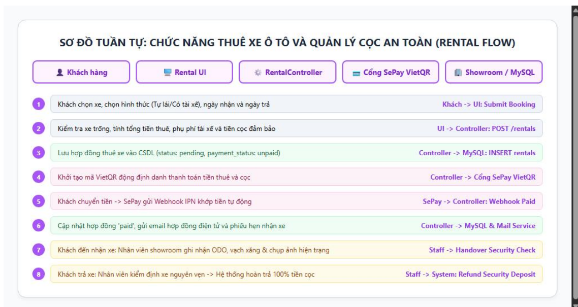
Hình 2.7: Sơ đồ tuần tự chức năng Thuê xe ô tô theo ngày và Quản lý cọc an toàn
