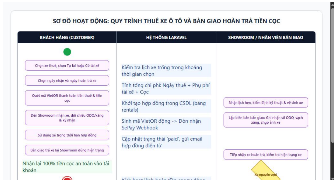
Hình 2.9: Sơ đồ hoạt động quy trình Thuê xe ô tô và Bàn giao hoàn trả tiền cọc
