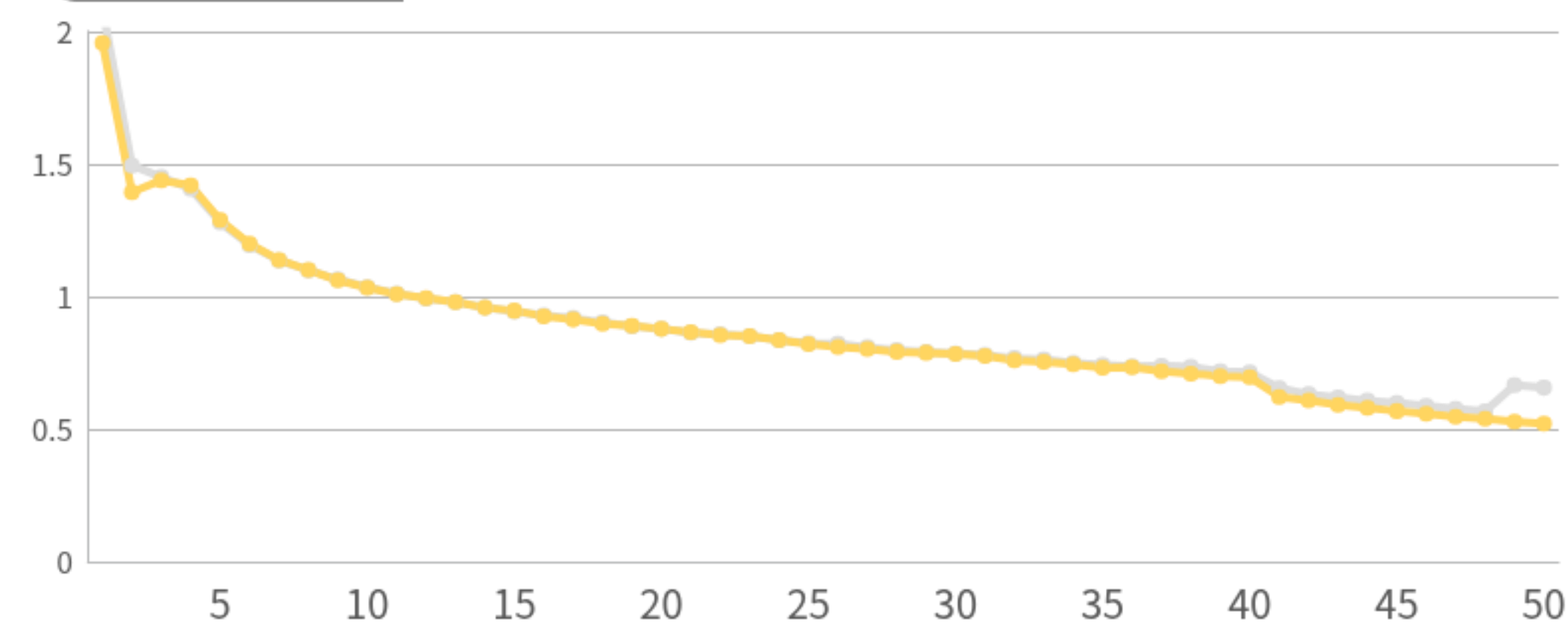
mAP50-95
