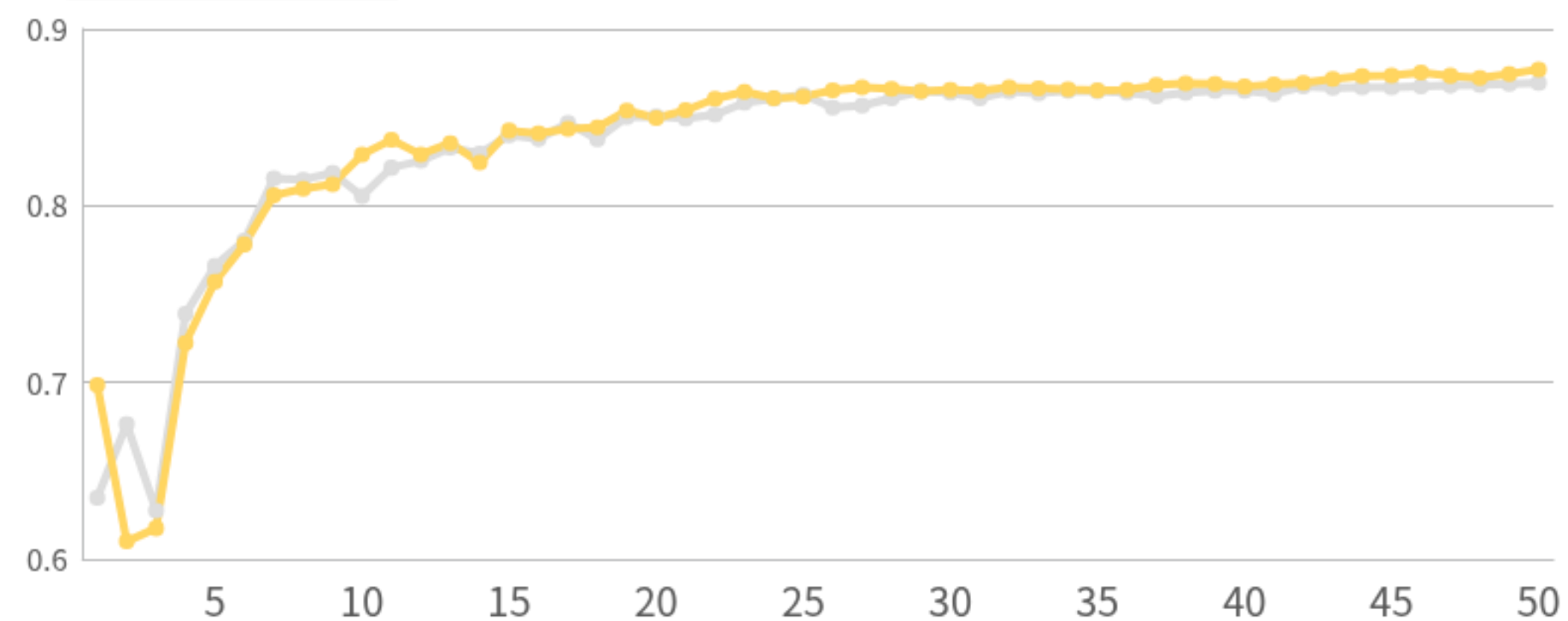
precision
