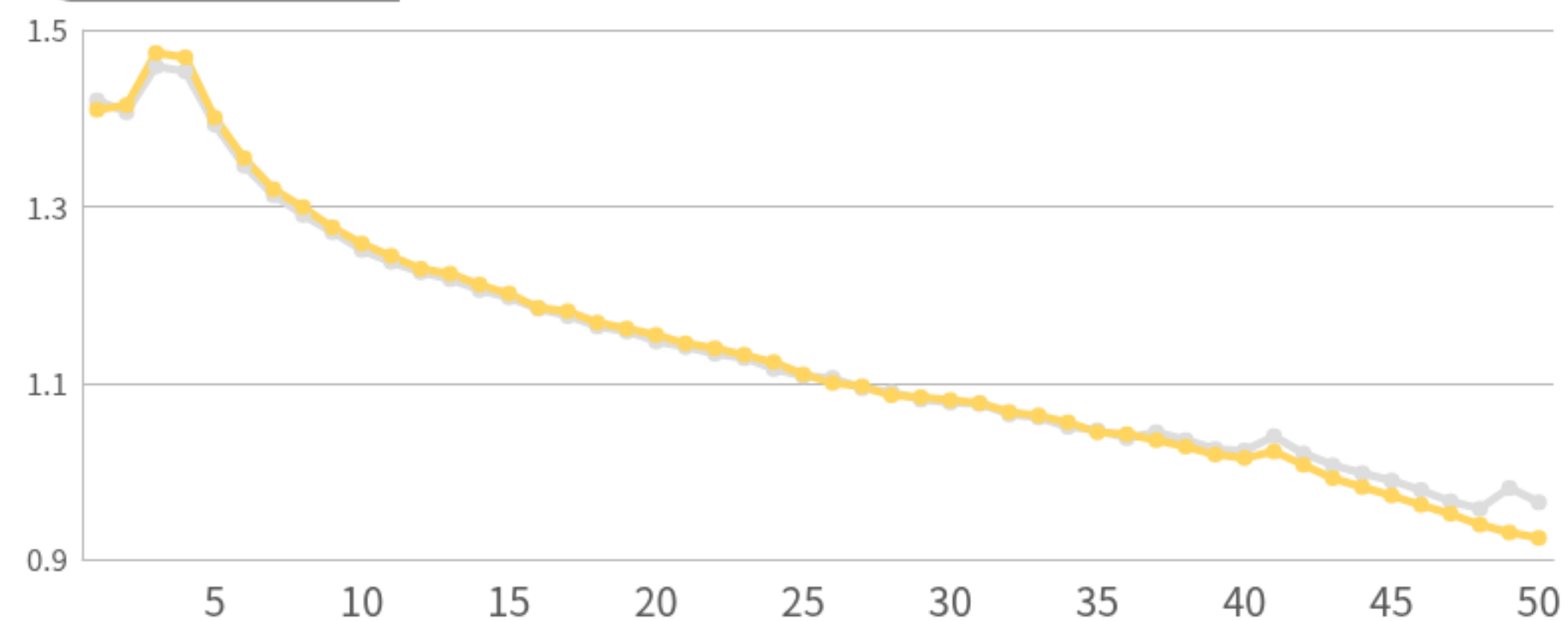
precision
