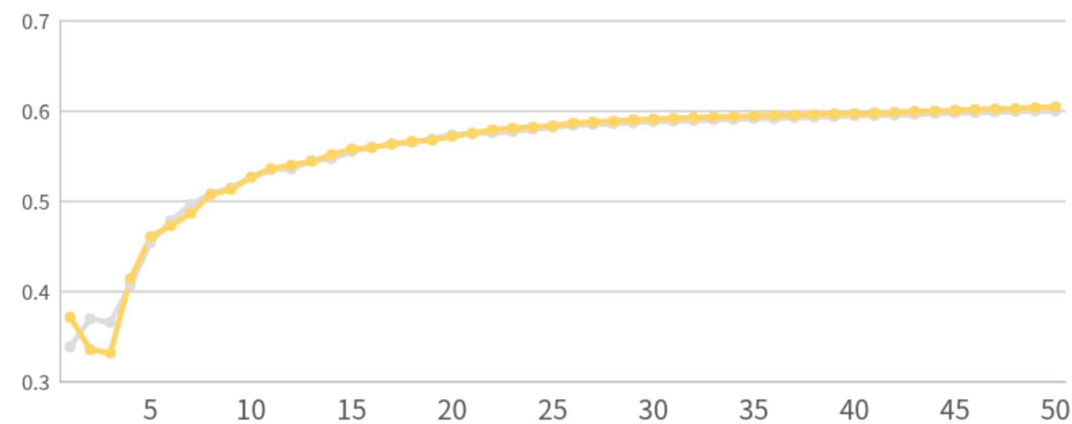
mAP50-95
