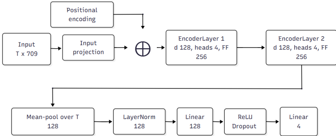
(d) openface_transformer.
