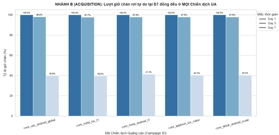
Hình 3. D1 / D3 / D7 retention theo UA campaign. D1 retention ~100% và D3 retention ~97–98% trên mọi campaign lớn — gần như giống hệt nhau. Sự giảm D7 (xuống ~40%) cũng đồng đều trên tất cả các kênh.
