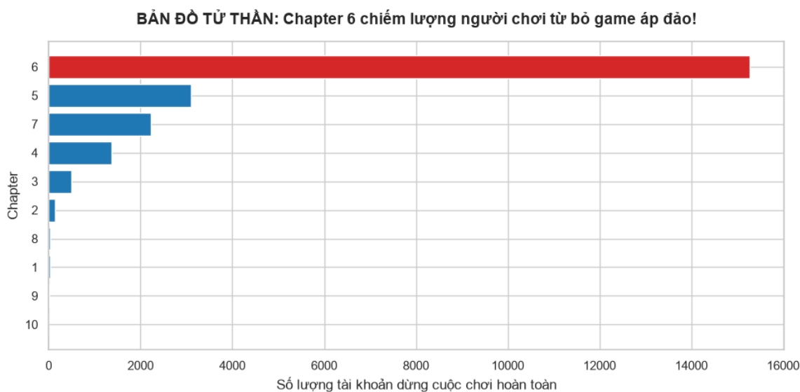
Hình 6. Số lượng người chơi churned có lần thử cuối cùng tại mỗi chapter. Chapter 6 là điểm drop-off chiếm ưu thế vượt trội - chiếm khoảng 73% số người chơi churned sớm, nhiều hơn tất cả các chapter khác cộng lại.
