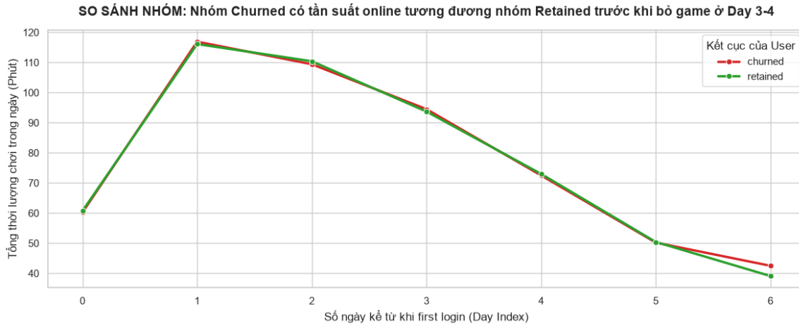
Hình 11. Thời gian chơi trung bình hàng ngày, F2P churned so với retained, Ngày 0–6. Hai nhóm gần như không thể phân biệt về thời gian chơi cho đến Ngày 4 - người chơi churned đã tương tác tích cực ngang với những người ở lại, một lần nữa củng cố rằng vấn đề là một rào cản chứ không phải sự khác biệt về mức độ hứng thú hoặc cam kết cơ bản.
