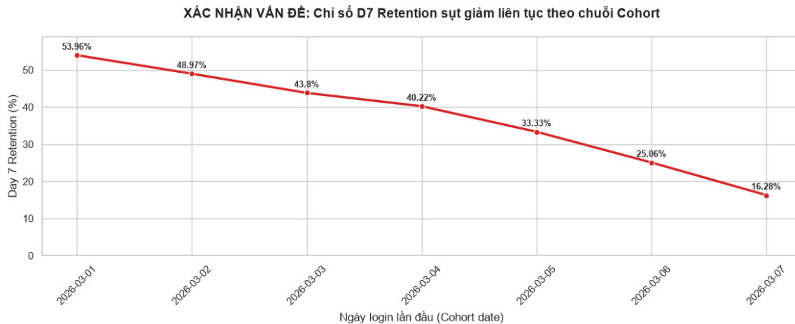
Hình 1. D7 retention theo cohort first-login, 1–7 tháng 3, 2026. Retention giảm đều đặn và đáng kể qua mọi cohort, từ 54,0% xuống 16,3% - giảm 38 điểm phần trăm chỉ trong một tuần.
