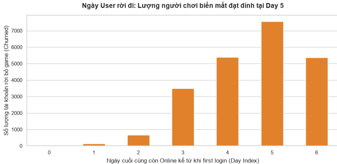
Hình 4. Phân phối ngày hoạt động cuối cùng của người chơi churned. Sự drop-off tăng tốc xuyên suốt tuần và đạt đỉnh vào ngày 5, với ngày 4 và 6 cũng cao - cho thấy một sự kiện churn tập trung vào giữa tuần, chứ không phải sự suy giảm dần dần.
