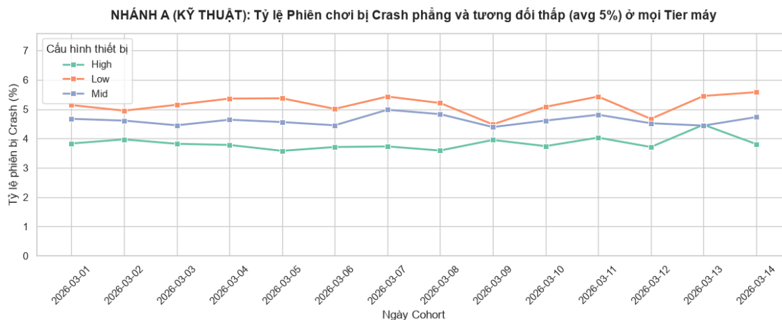
Hình 2. Tỷ lệ crash session theo device tier và ngày cohort. Tỷ lệ crash ổn định ở mức ~4–5% trên mọi ngày và mọi device tier, không có xu hướng tăng và không có đột biến nào.
