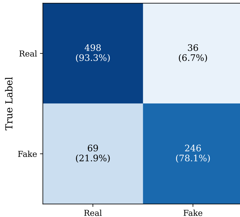
SVM
