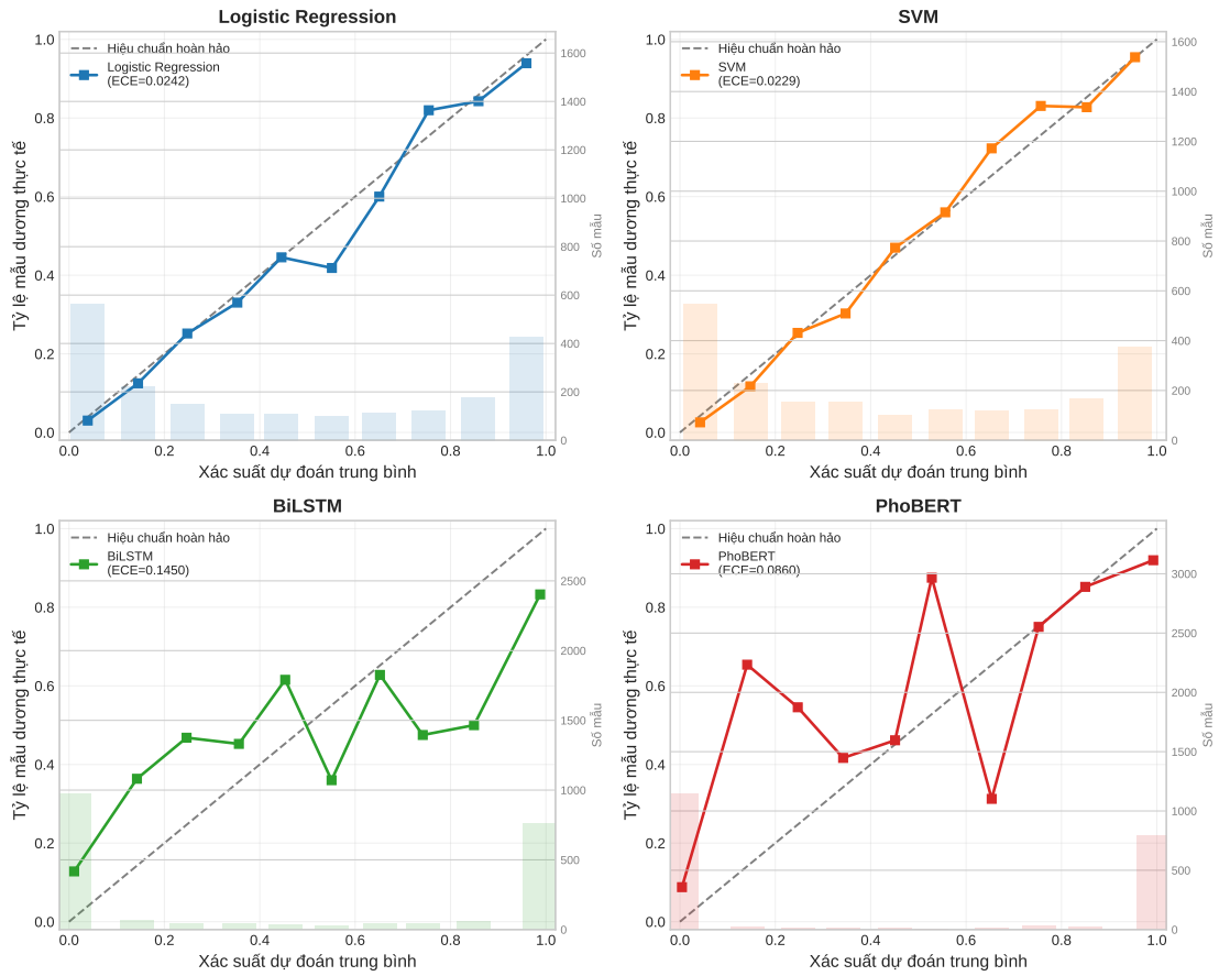
Hình 5.5: Biểu đồ hiệu chuẩn (Reliability Diagram) của bốn mô hình trên tập kiểm tra. Đường chéo nét đứt biểu diễn hiệu chuẩn hoàn hảo; các điểm vuông biểu diễn tỷ lệ dương tính thực tế trong mỗi bin xác suất.
