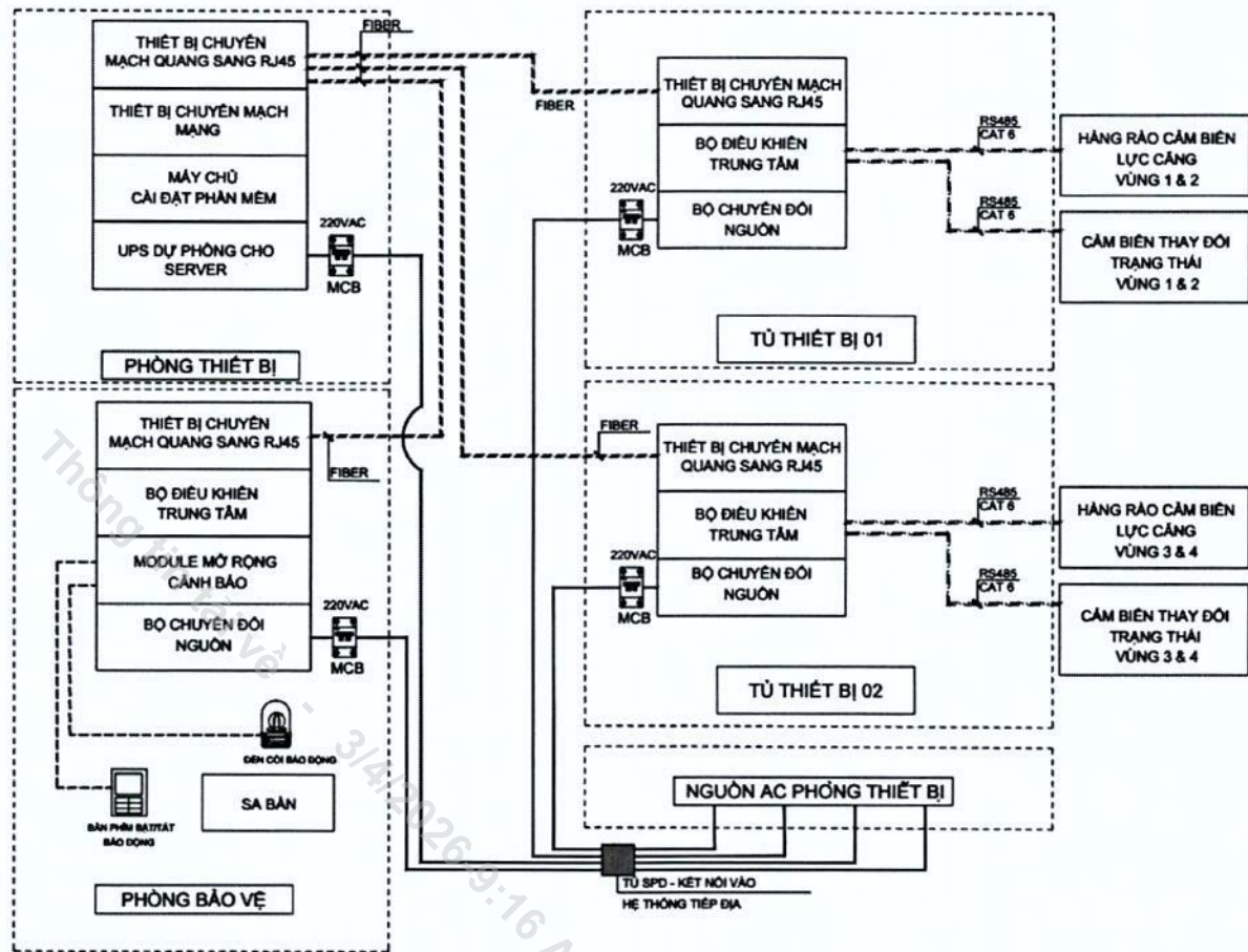
Hình 1. Sơ đồ nguyên lý hệ thống hàng rào điện tử sử dụng công nghệ dây căng có cảm biến lực căng dây vật lý phát hiện và cảnh báo xâm nhập gồm có các thiết bị chính và các thiết bị phụ trợ
