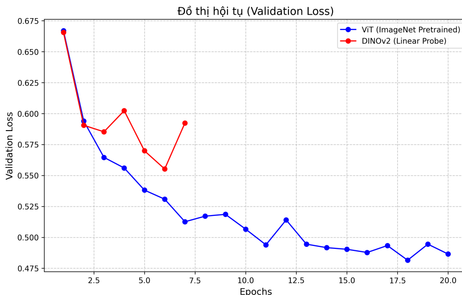
Hình 2.1: Tốc độ hội tụ (Validation Loss) của các mô hình
