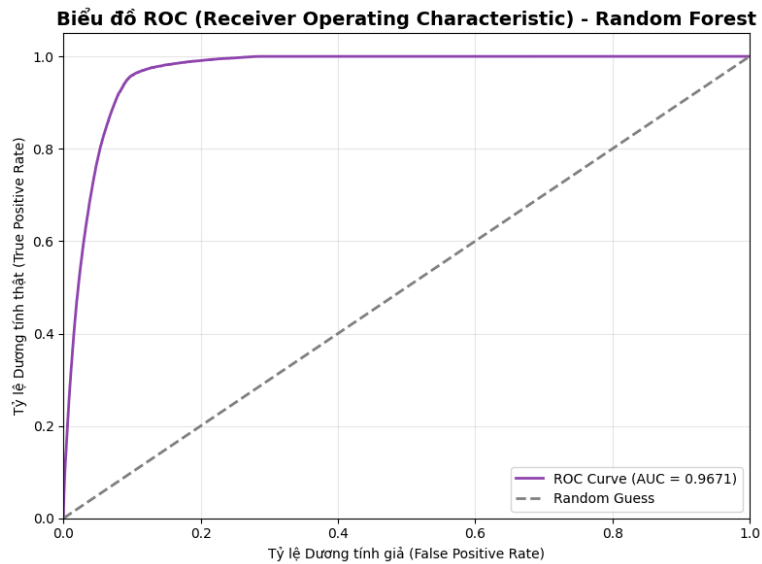
Hình 23: ROC của mô hình Random Forest
