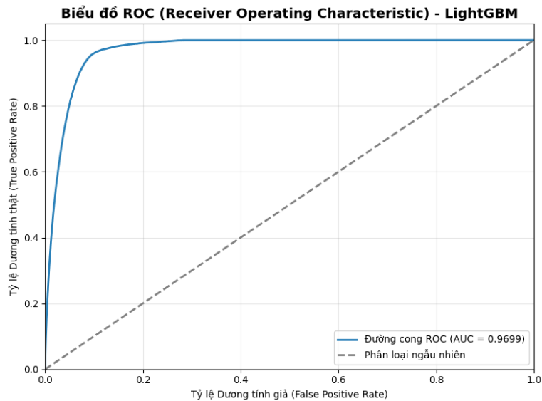
Hình 24: Đồ thị ROC của LightGBM
