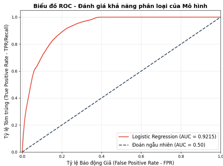
Hình 22: Biểu đồ ROC
