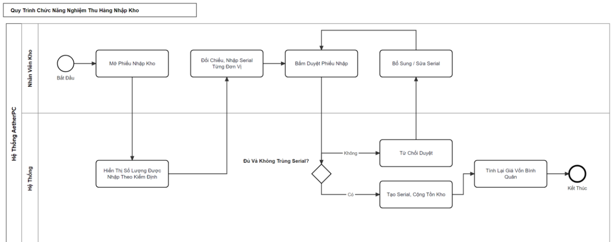
Hình 3.17 Sơ đồ BPMN quy trình chức năng nghiệp thu hàng nhập kho
