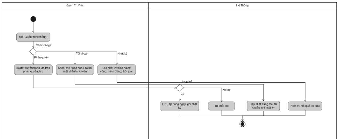
Hình 3.76 Sơ đồ hoạt động use case Quản trị tài khoản, phân quyền và nhật ký
