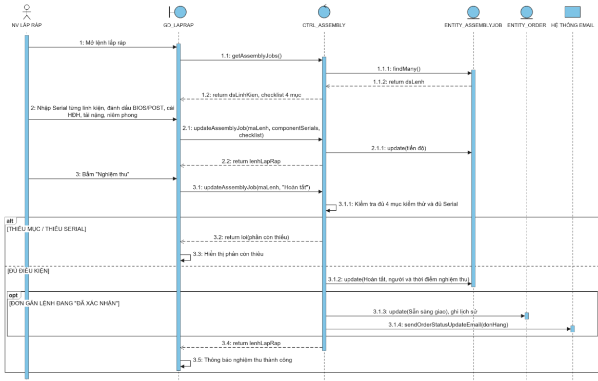
Hình 3.57 Sơ đồ tuần tự use case Cập nhật tiến độ lắp ráp
