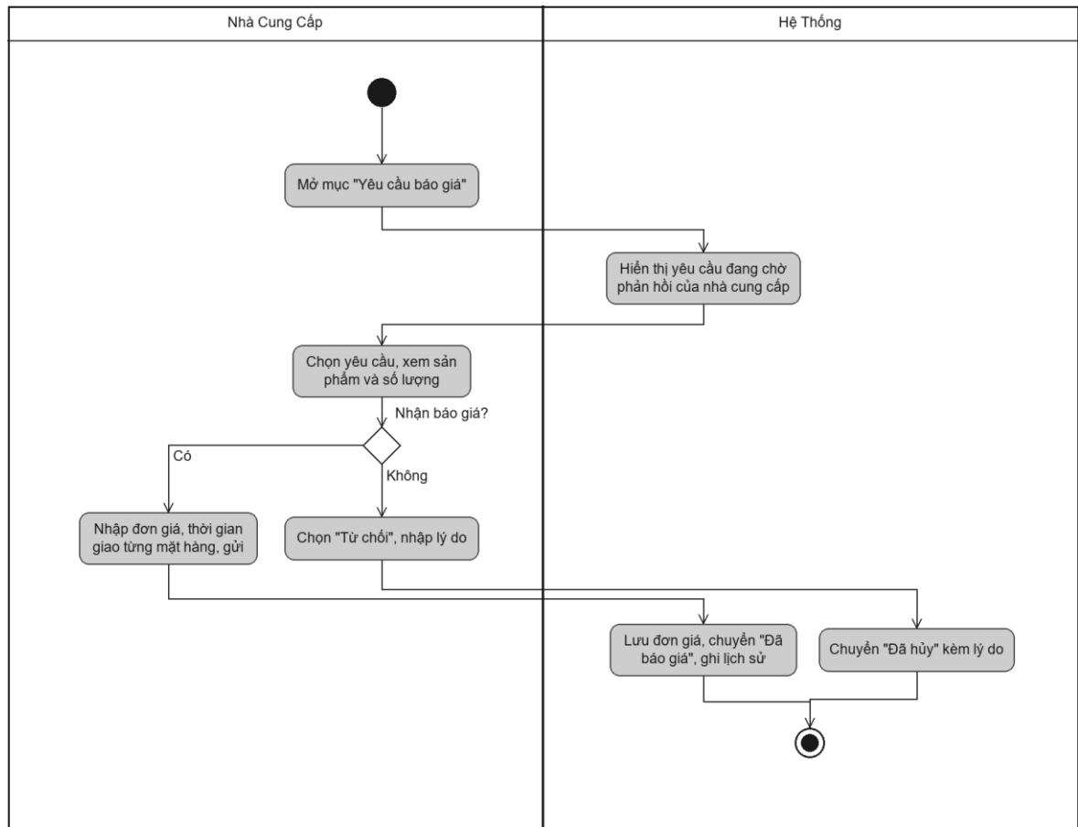
Hình 3.46 Sơ đồ hoạt động use case Phản hồi yêu cầu báo giá
