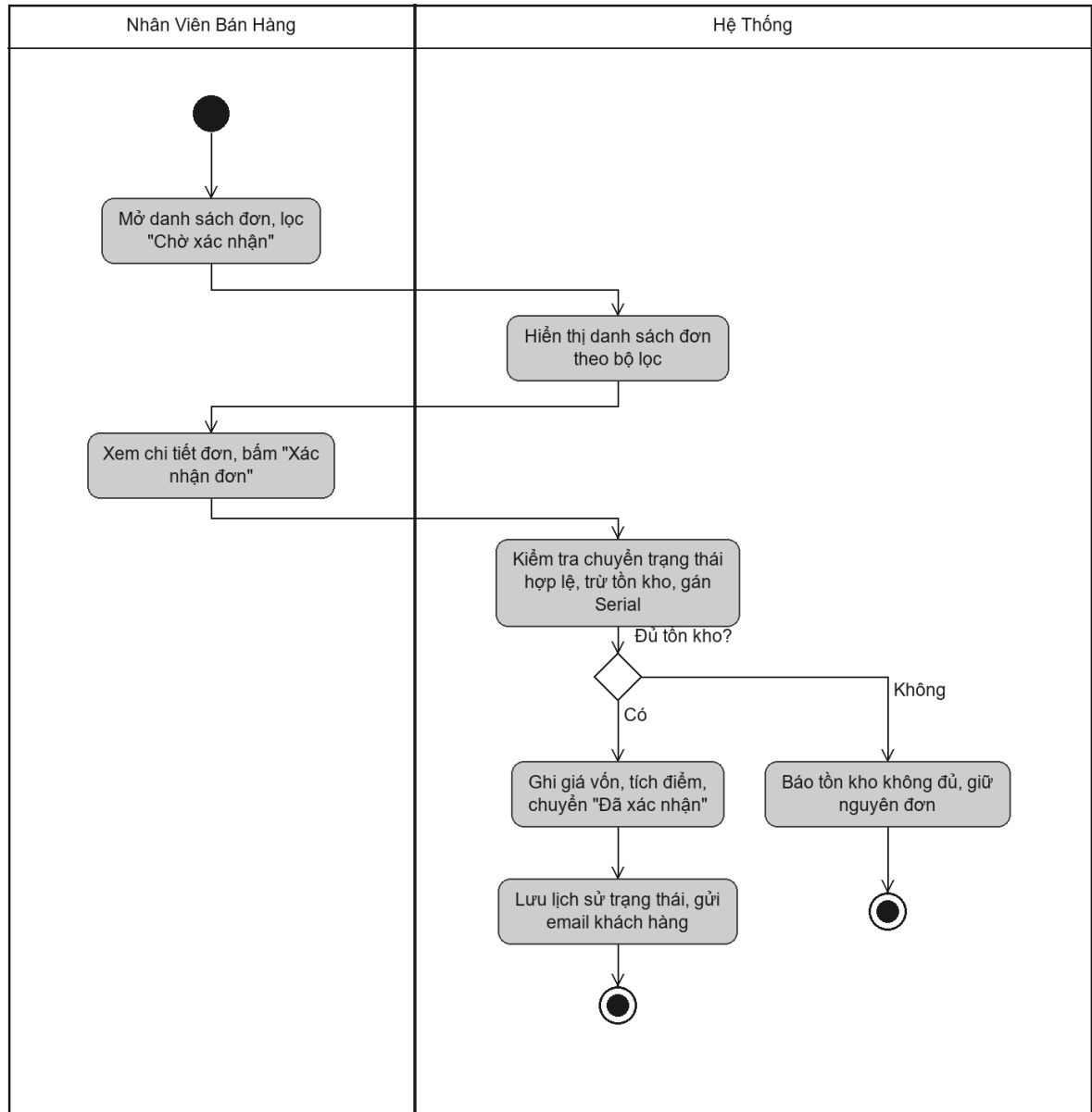
Hình 3.42 Sơ đồ hoạt động use case Xử lý và cập nhật đơn hàng
