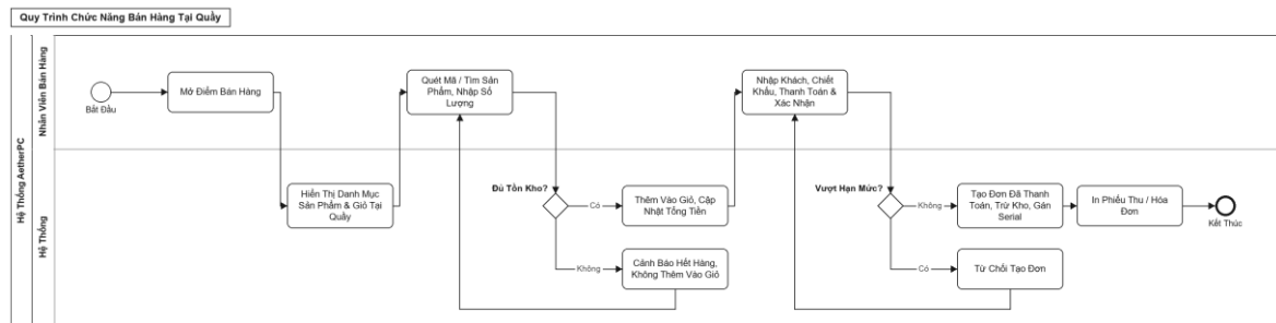
Hình 3.10 Sơ đồ BPMN quy trình chức năng bán hàng tại quầy
