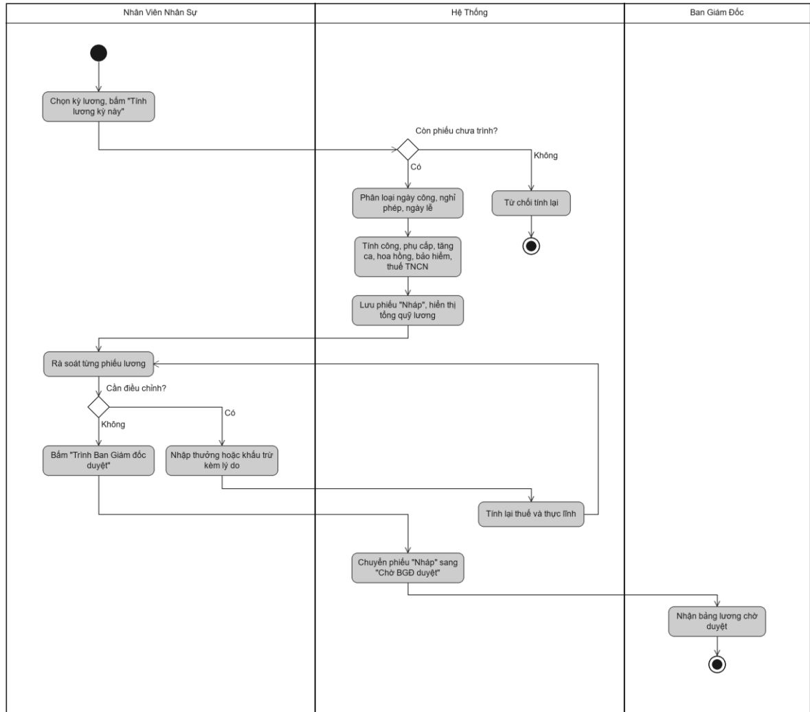
Hình 3.70 Sơ đồ hoạt động use case Tính lương và trình duyệt bảng lương
