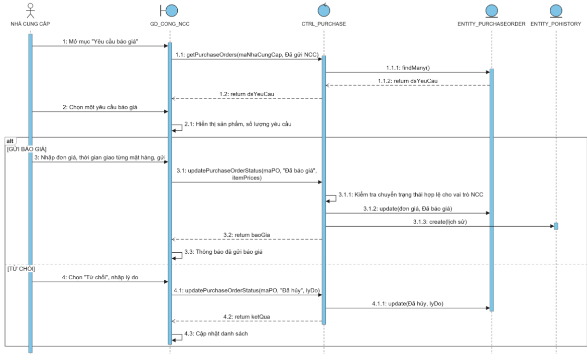
Hình 3.47 Sơ đồ tuần tự use case Phản hồi yêu cầu báo giá
