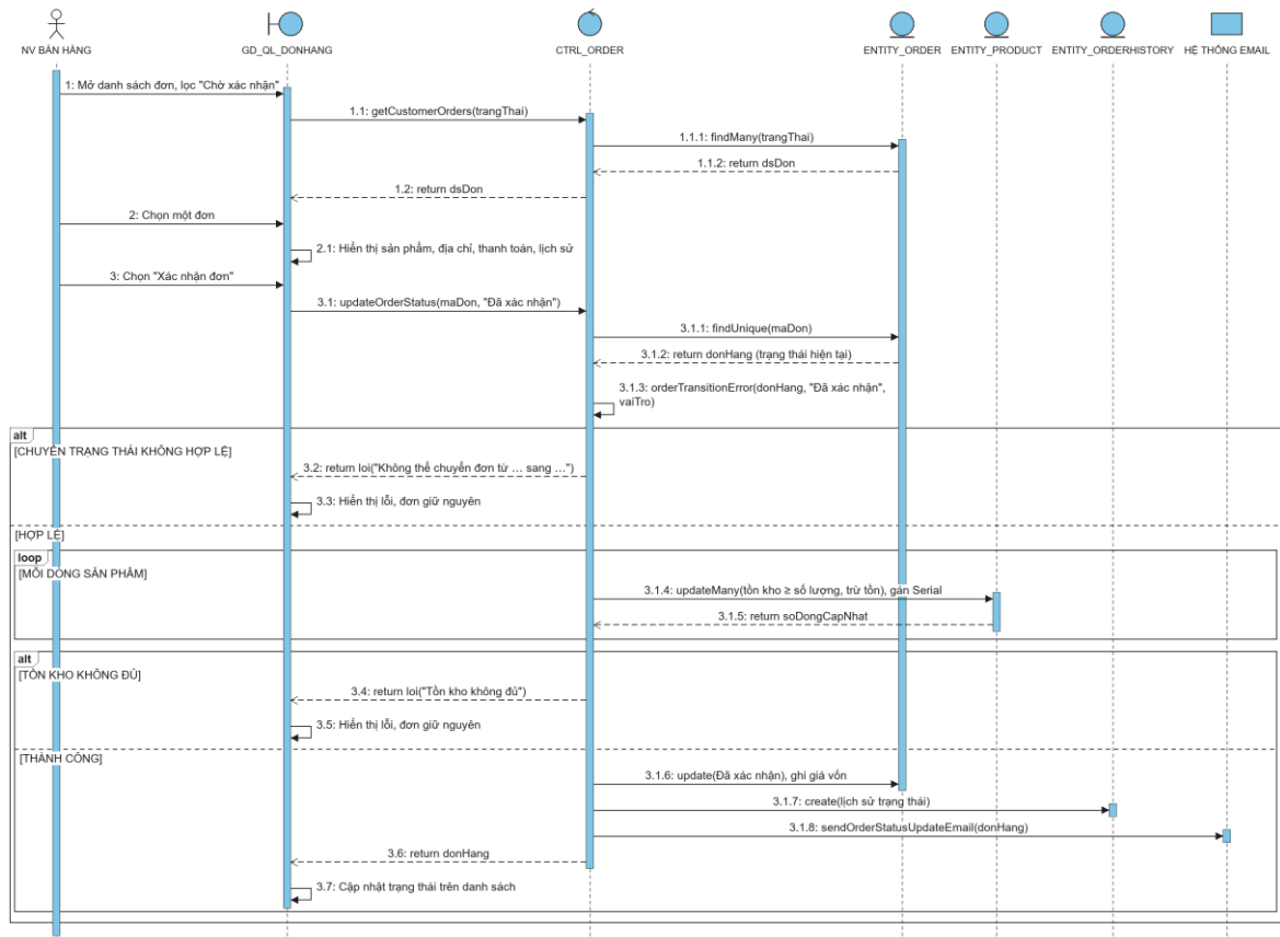
Hình 3.43 Sơ đồ tuần tự use case Xử lý và cập nhật đơn hàng
