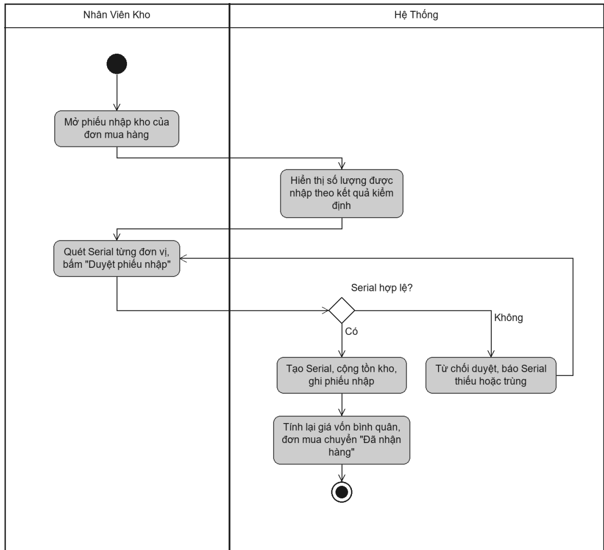
Hình 3.54 Sơ đồ hoạt động use case Nghiệm thu hàng nhập kho
