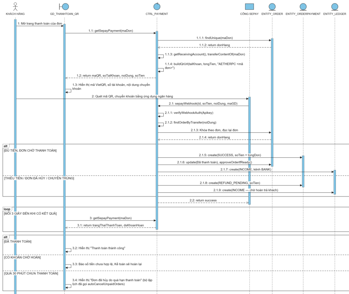
Hình 3.37 Sơ đồ tuần tự use case Chọn phương thức và xác nhận thanh toán
