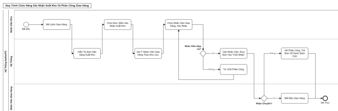
Hình 3.19 Sơ đồ BPMN quy trình chức năng xác nhận xuất kho và phân công giao hàng
