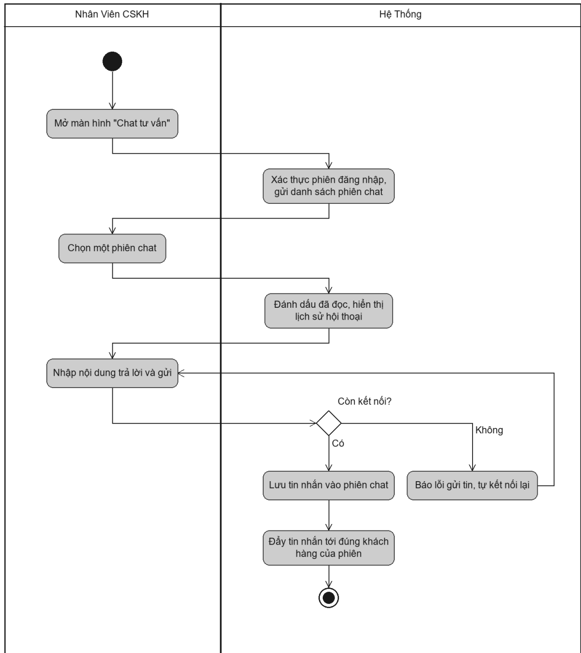
Hình 3.38 Sơ đồ hoạt động use case Trả lời chat trực tuyến
