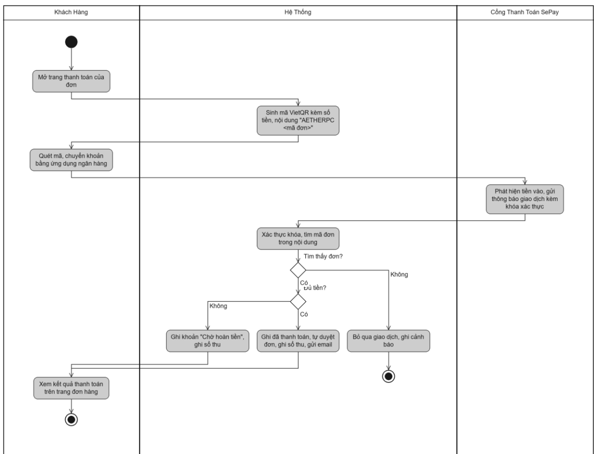
Hình 3.36 Sơ đồ hoạt động use case Chọn phương thức và xác nhận thanh toán
