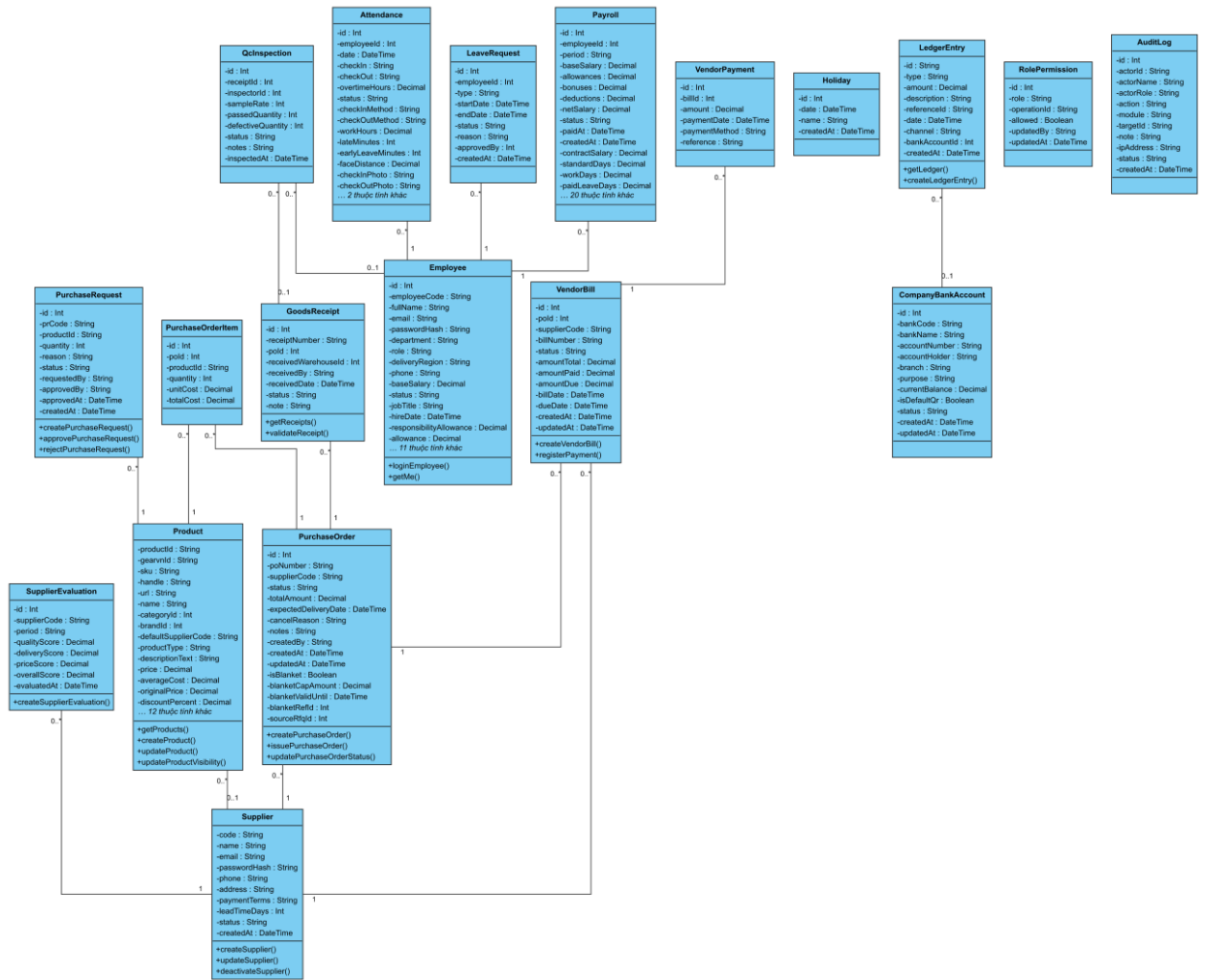
Hình 3.80 Sơ đồ lớp thực thể phân hệ mua hàng, nhân sự và kế toán
