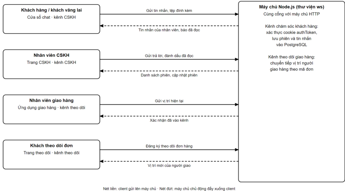
Hình 2.4 Mô hình kết nối WebSocket giữa máy chủ và các client
