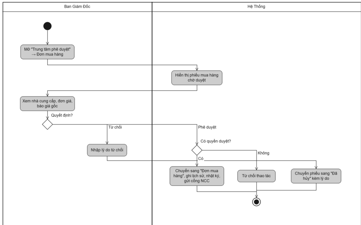
Hình 3.48 Sơ đồ hoạt động use case Duyệt đơn mua hàng
