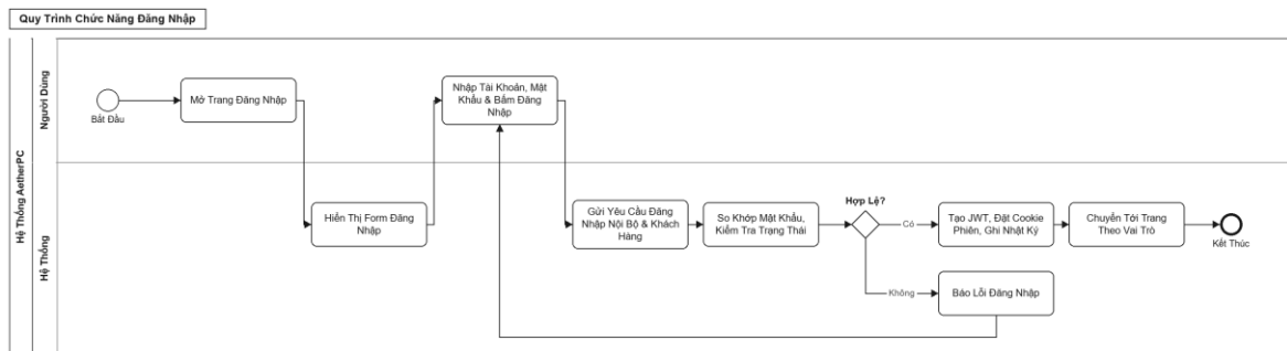
Hình 3.27 Sơ đồ BPMN quy trình chức năng đăng nhập
