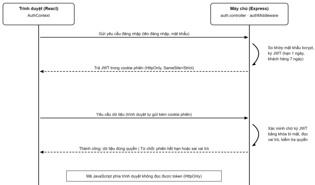
Hình 2.3 Luồng xác thực người dùng dựa trên JWT
