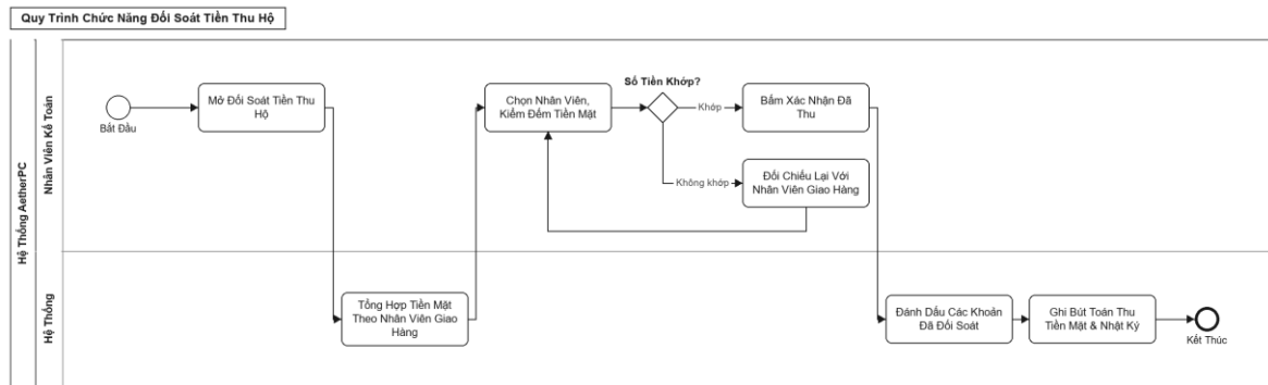
Hình 3.22 Sơ đồ BPMN quy trình chức năng đối soát tiền thu hộ
