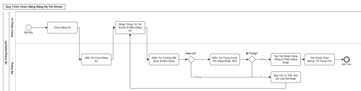
Hình 3.5 Sơ đồ BPMN quy trình chức năng đăng ký tài khoản
