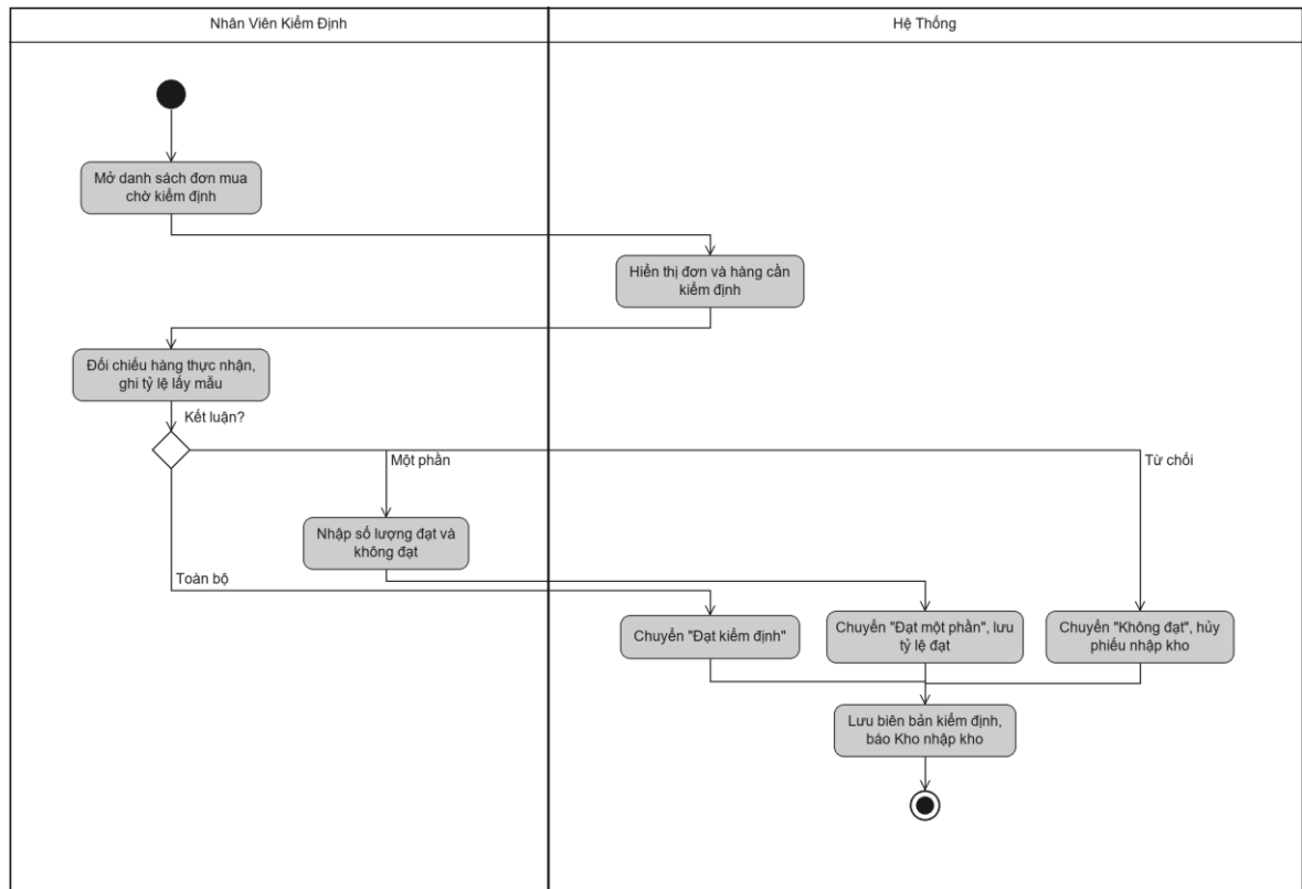
Hình 3.50 Sơ đồ hoạt động use case Kiểm tra chất lượng hàng nhập
