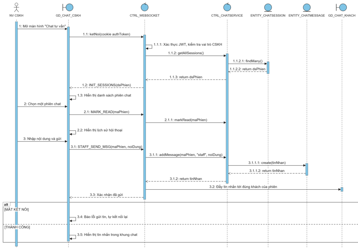
Hình 3.39 Sơ đồ tuần tự use case Trả lời chat trực tuyến
