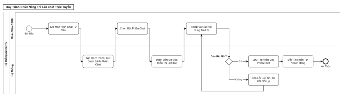
Hình 3.9 Sơ đồ BPMN quy trình chức năng trả lời chat trực tuyến
