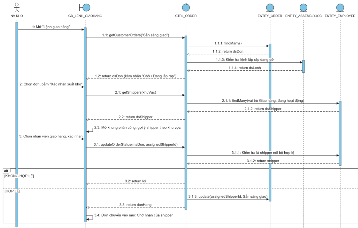
Hình 3.59 Sơ đồ tuần tự use case Xác nhận xuất kho và phân công giao hàng
