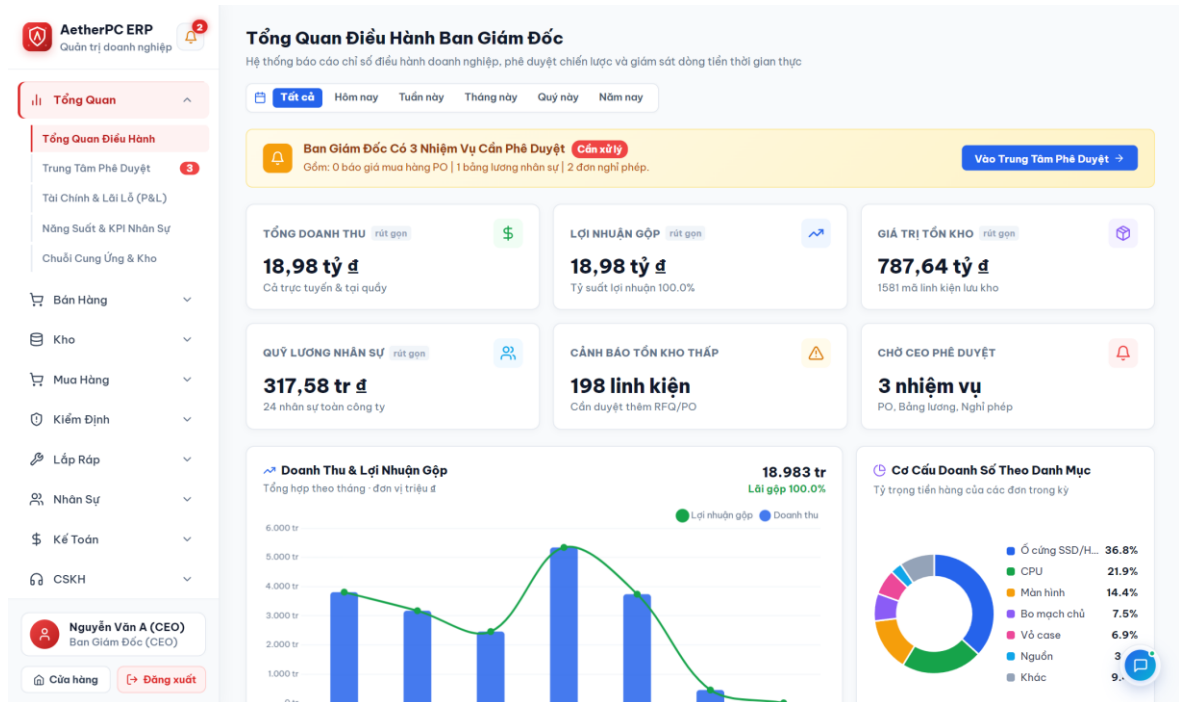
Hình 5.34 Giao diện tổng quan điều hành
