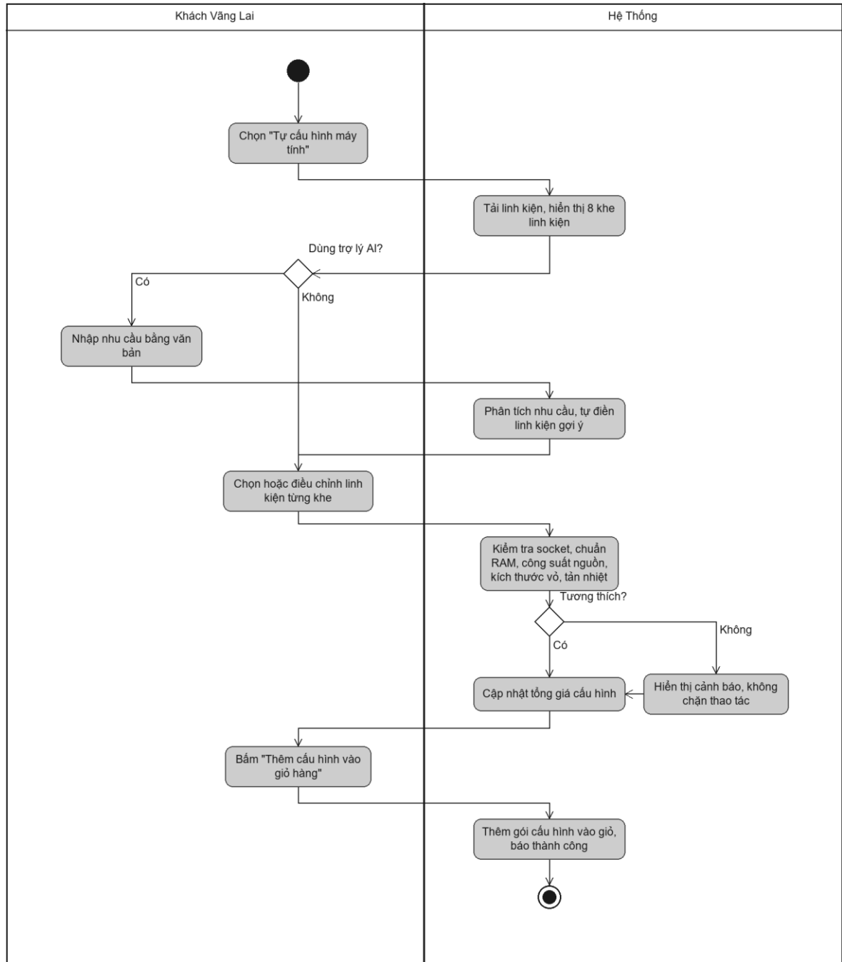
Hình 3.32 Sơ đồ hoạt động use case Tự cấu hình máy tính
