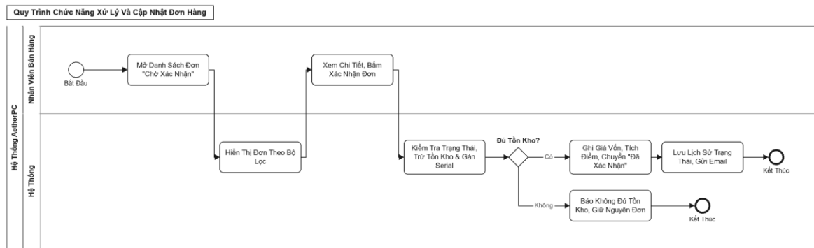
Hình 3.11 Sơ đồ BPMN quy trình chức năng xử lý và cập nhật đơn hàng
