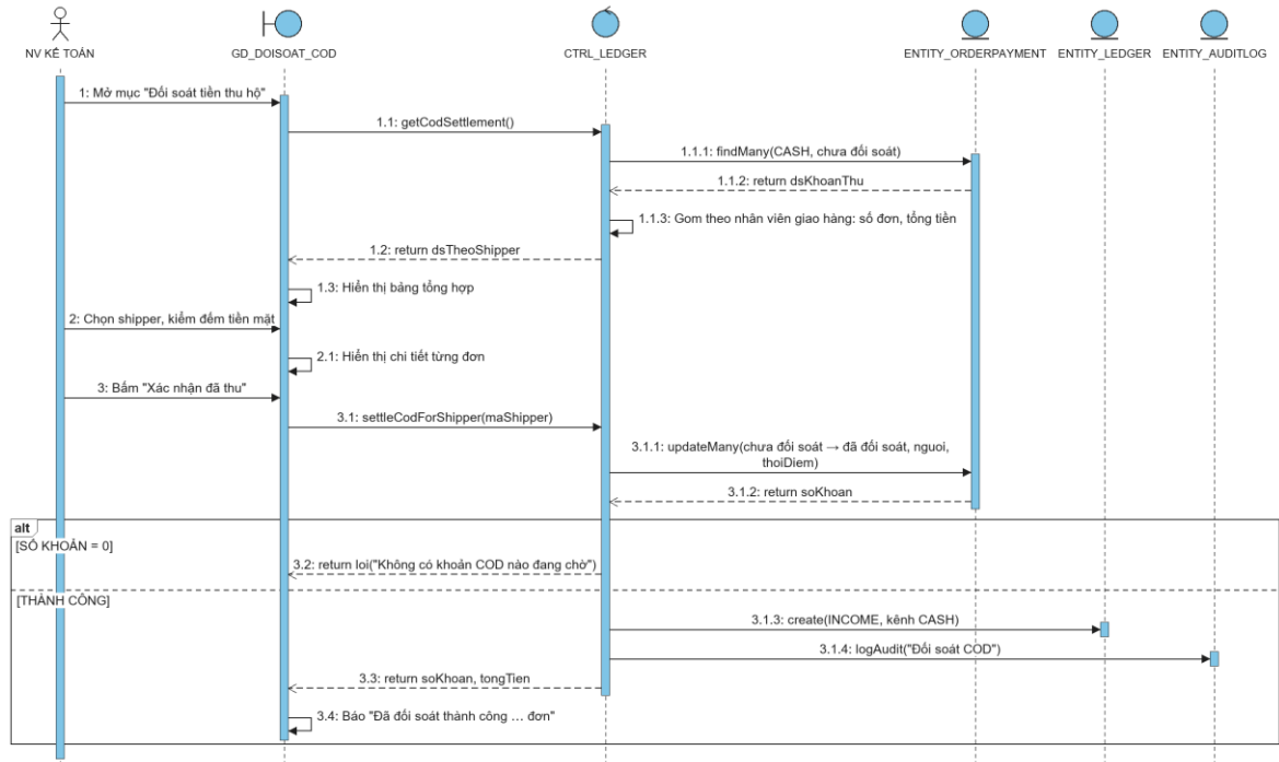
Hình 3.65 Sơ đồ tuần tự use case Đối soát tiền thu hộ
