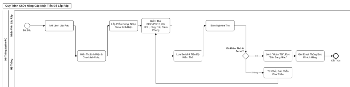
Hình 3.18 Sơ đồ BPMN quy trình chức năng cập nhật tiến độ lắp ráp
