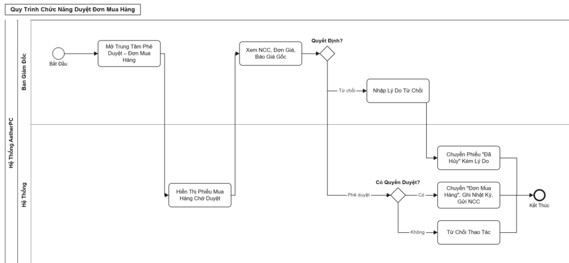
Hình 3.14 Sơ đồ BPMN quy trình chức năng duyệt đơn mua hàng
