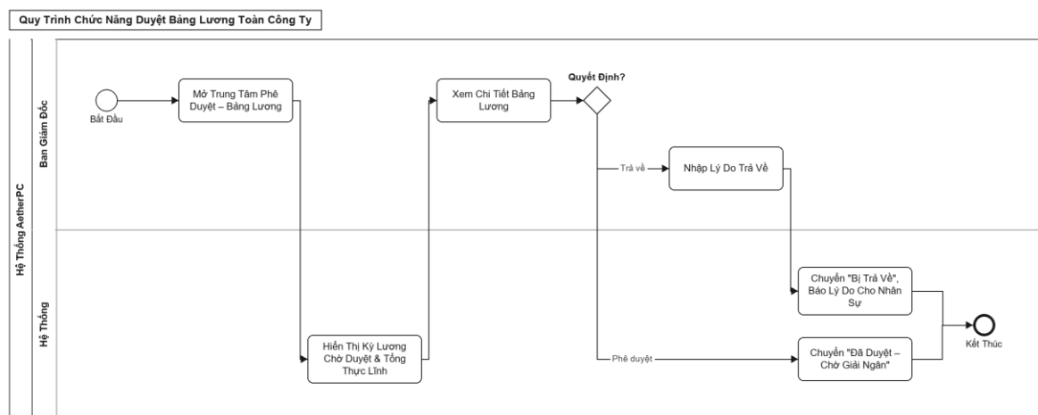
Hình 3.26 Sơ đồ BPMN quy trình chức năng duyệt bảng lương toàn công ty
