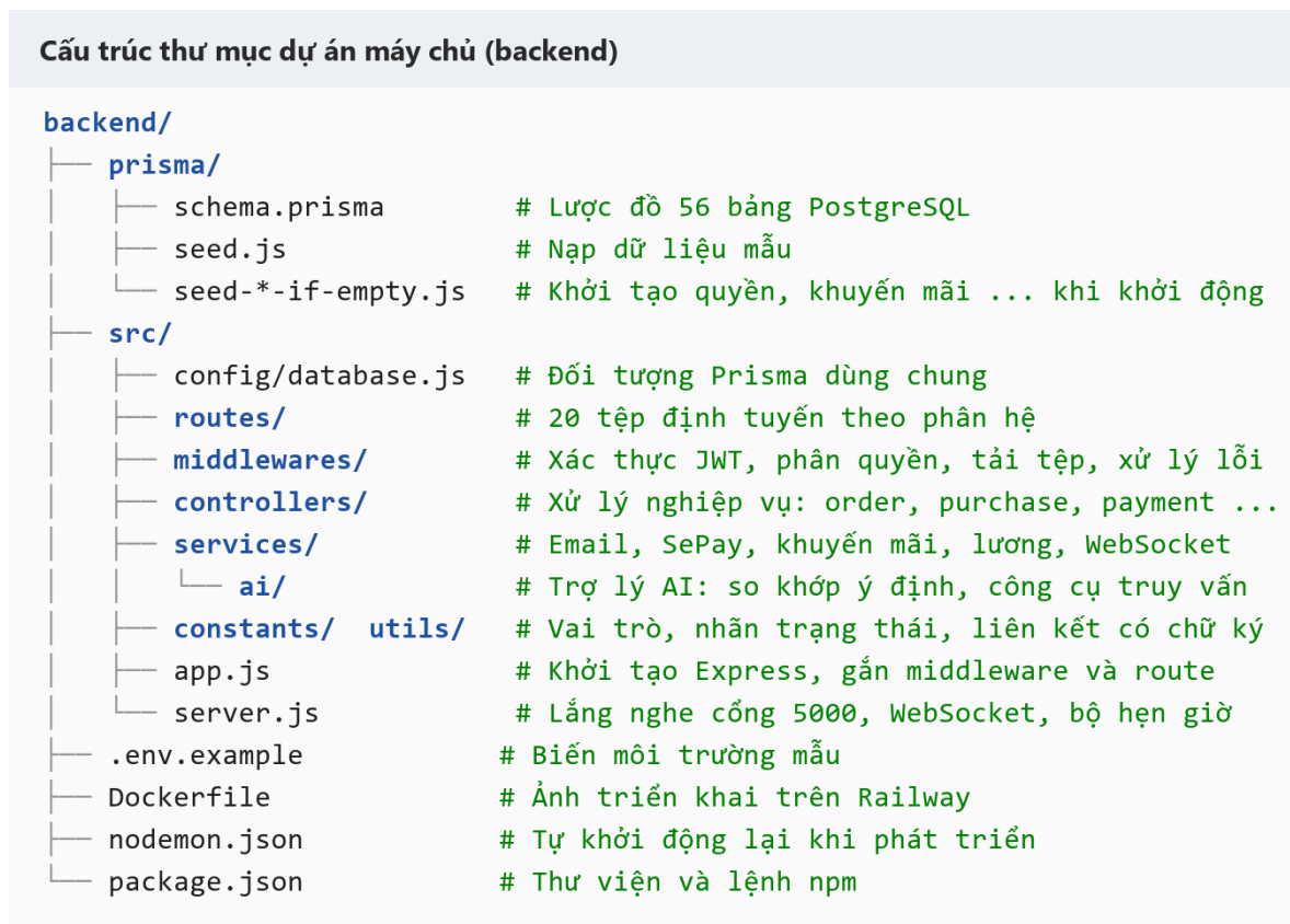
Hình 5.3 Cấu trúc thư mục dự án máy chủ
