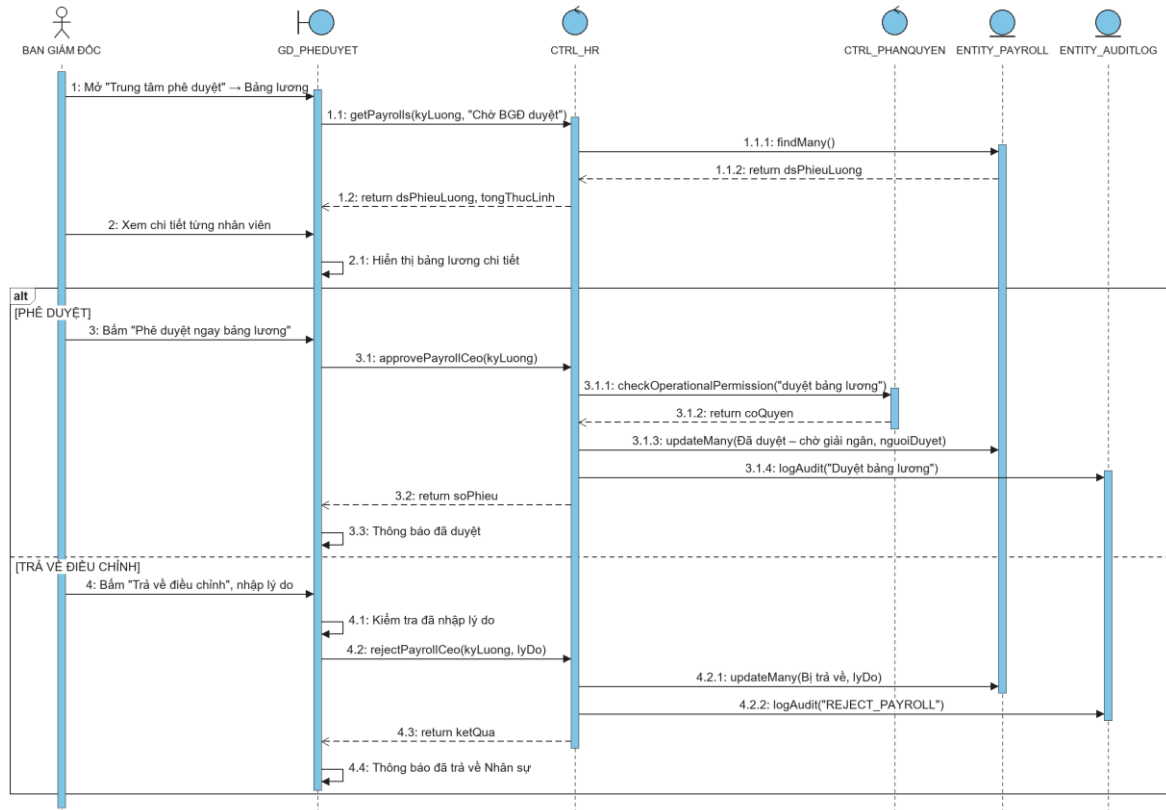
Hình 3.73 Sơ đồ tuần tự use case Duyệt bảng lương toàn công ty
