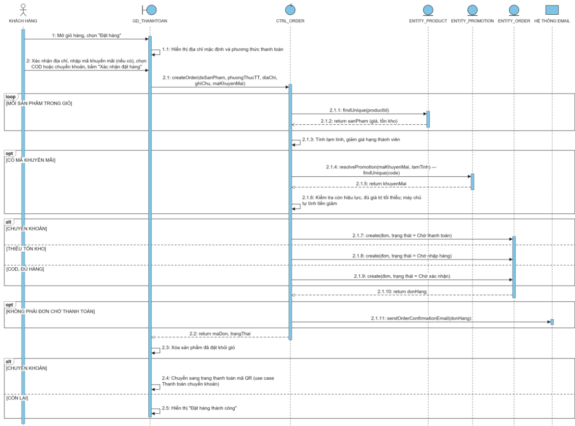
Hình 3.35 Sơ đồ tuần tự use case Đặt hàng
