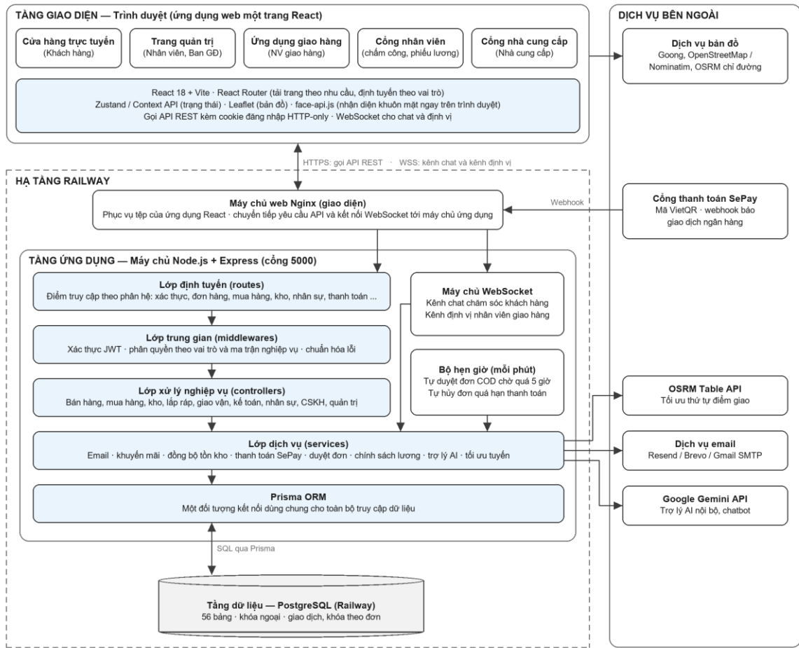
Hình 4.1 Kiến trúc tổng thể của hệ thống
