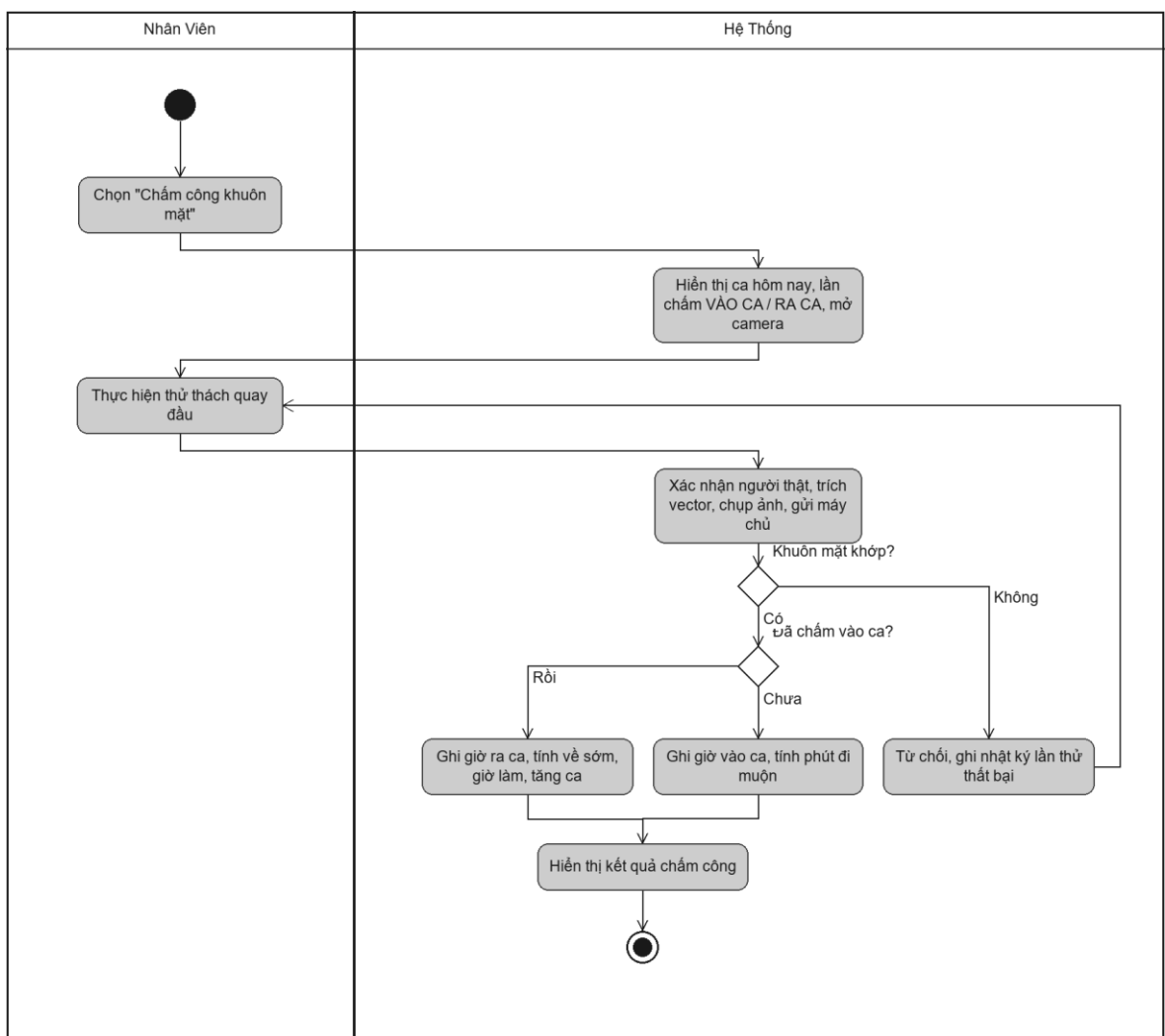
Hình 3.68 Sơ đồ hoạt động use case Chấm công bằng khuôn mặt
