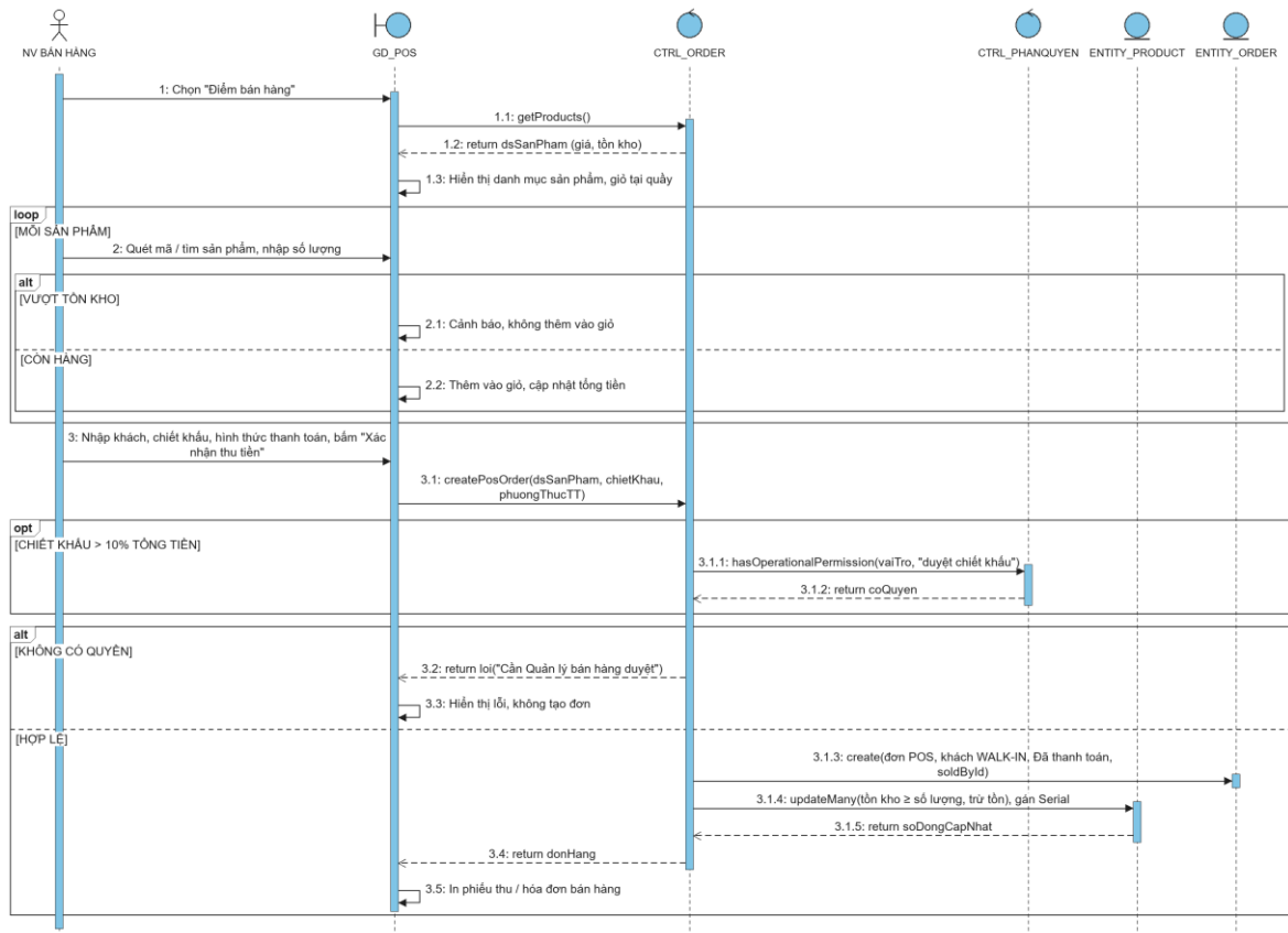
Hình 3.41 Sơ đồ tuần tự use case Bán hàng tại quầy
