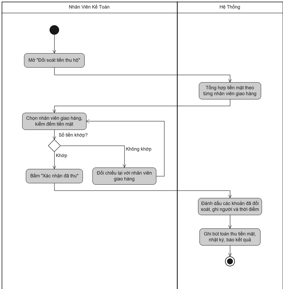
Hình 3.64 Sơ đồ hoạt động use case Đối soát tiền thu hộ
