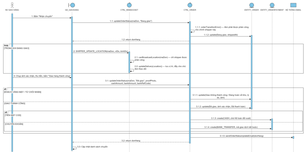
Hình 3.61 Sơ đồ tuần tự use case Giao hàng và thu tiền hộ
