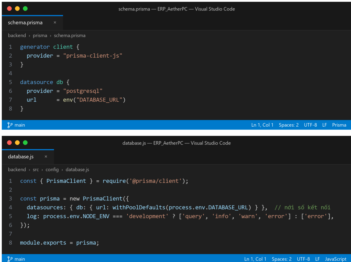
Hình 5.8 Khai báo kết nối cơ sở dữ liệu qua Prisma
