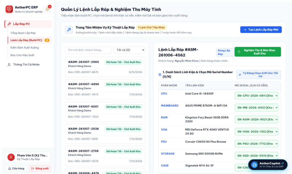
Hình 5.27 Giao diện quản lý lệnh lắp ráp
