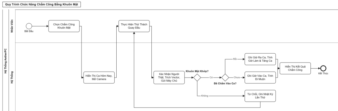
Hình 3.24 Sơ đồ BPMN quy trình chức năng chấm công bằng khuôn mặt
