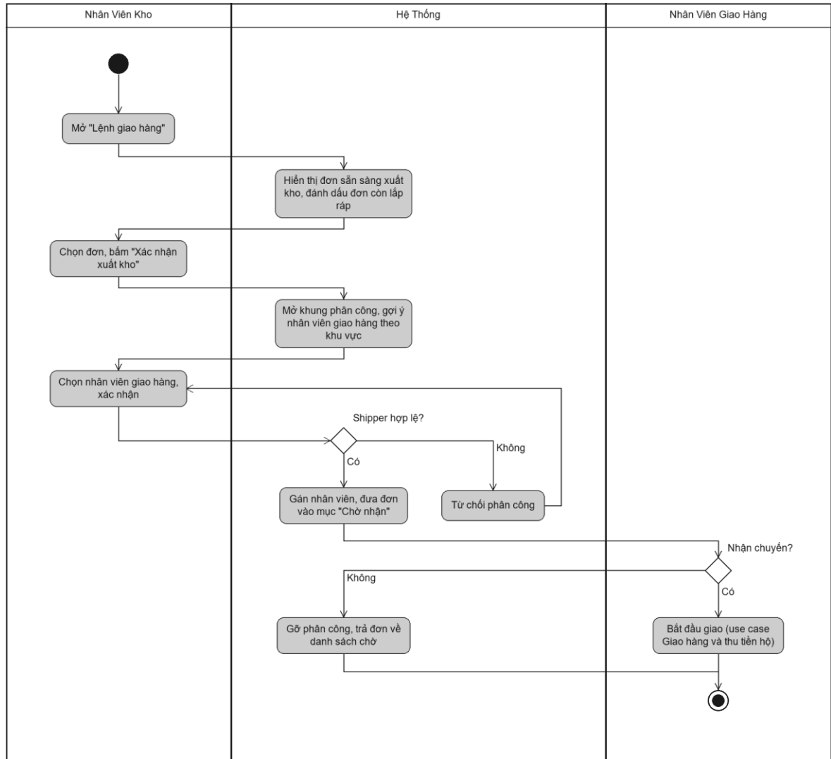
Hình 3.58 Sơ đồ hoạt động use case Xác nhận xuất kho và phân công giao hàng
