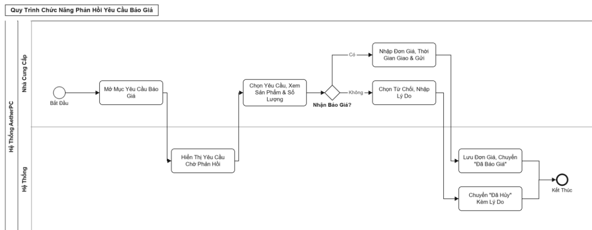
Hình 3.13 Sơ đồ BPMN quy trình chức năng phản hồi yêu cầu báo giá
