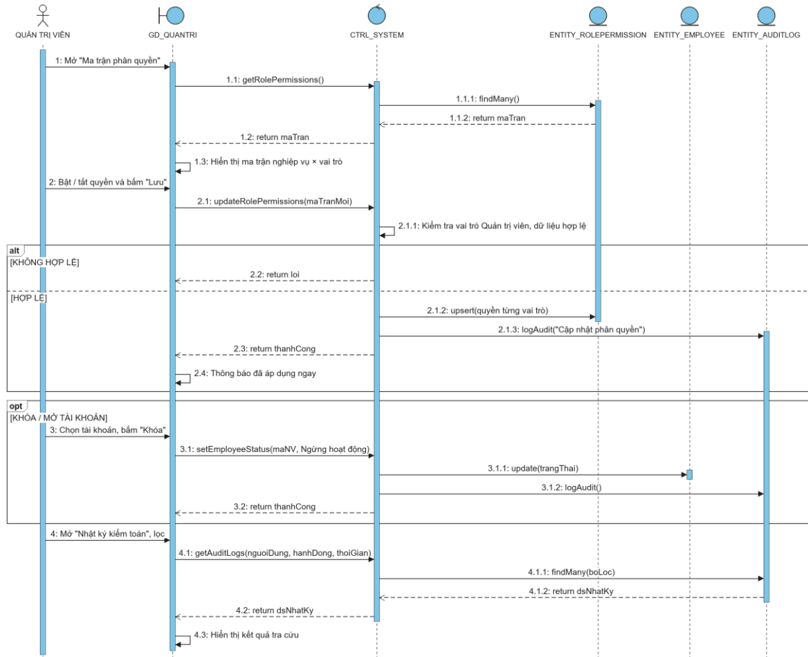
Hình 3.77 Sơ đồ tuần tự use case Quản trị tài khoản, phân quyền và nhật ký
