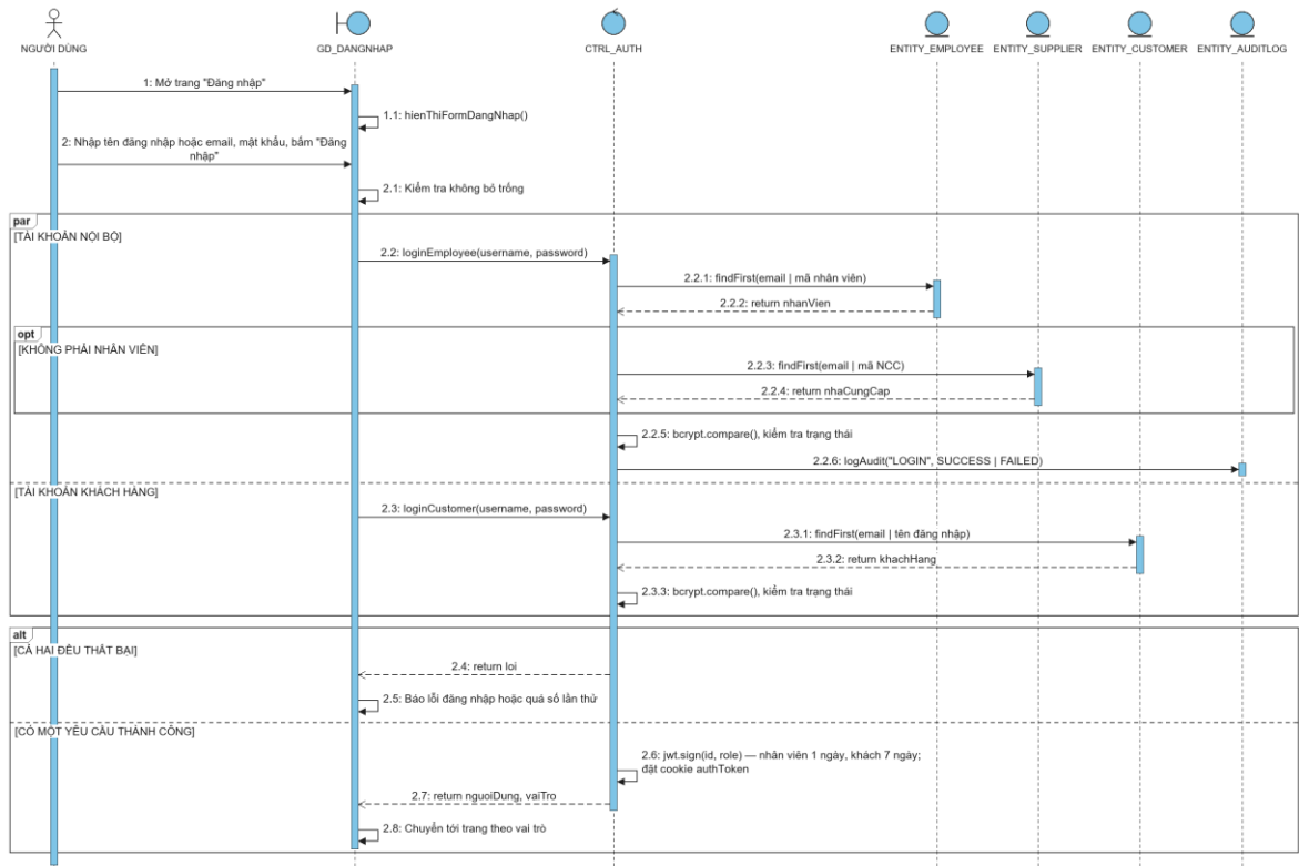
Hình 3.75 Sơ đồ tuần tự use case Đăng nhập
