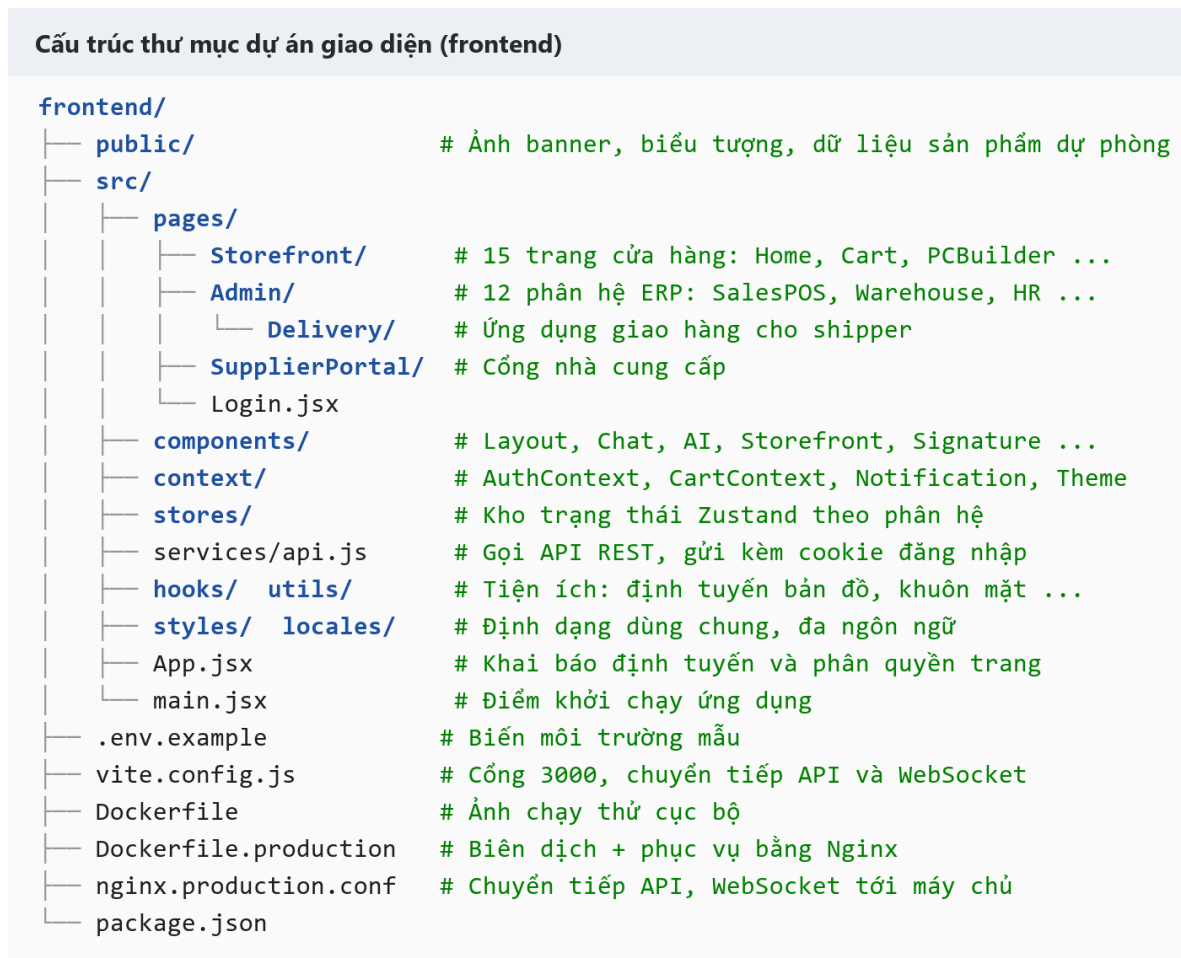
Hình 5.2 Cấu trúc thư mục dự án giao diện
