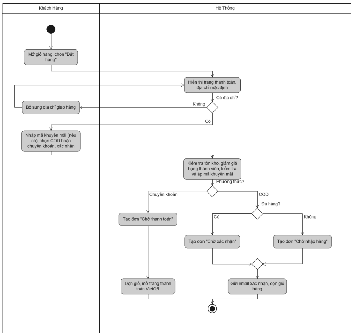
Hình 3.34 Sơ đồ hoạt động use case Đặt hàng
