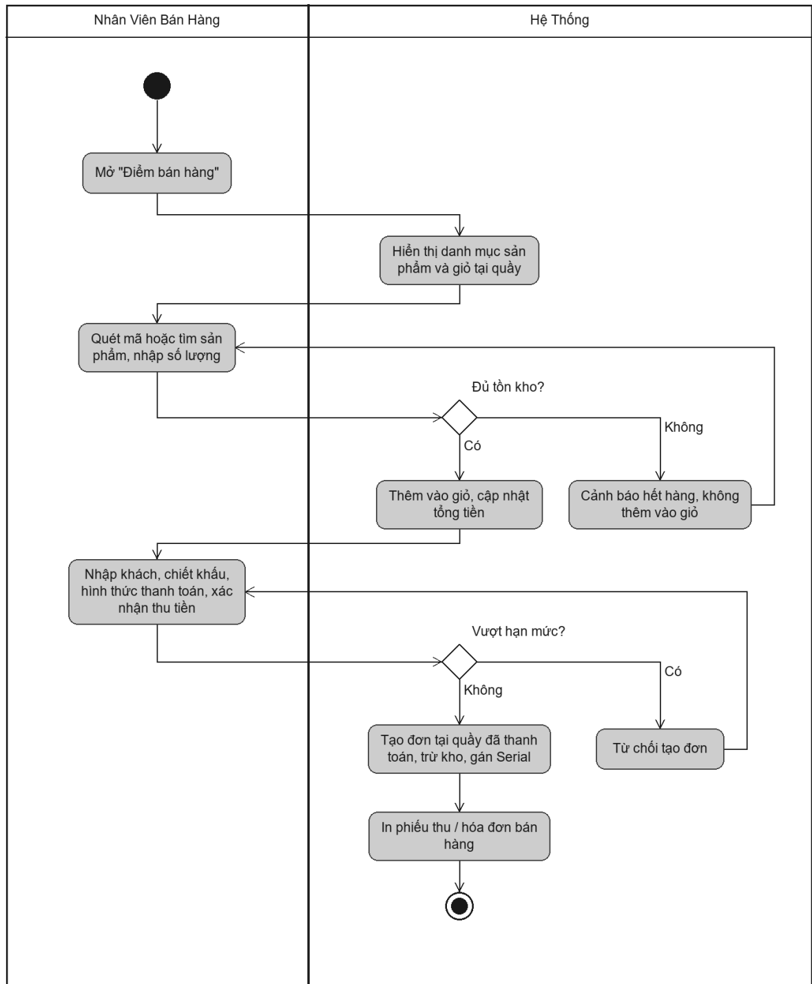
Hình 3.40 Sơ đồ hoạt động use case Bán hàng tại quầy
