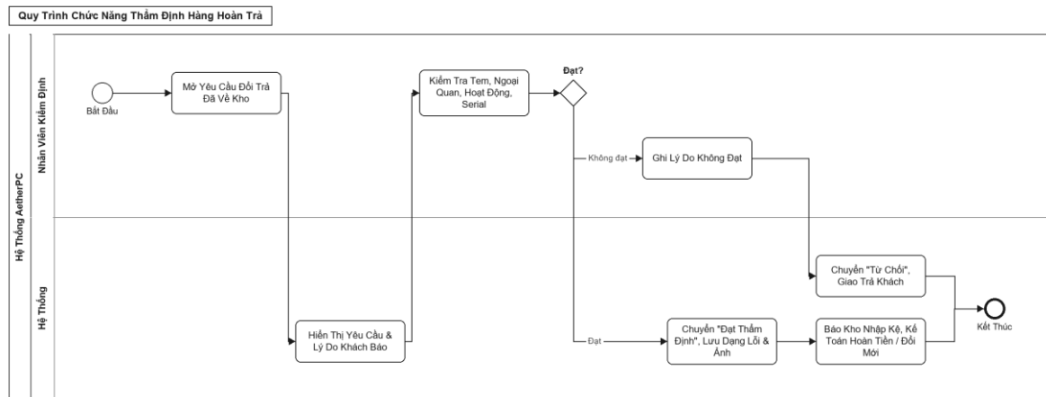
Hình 3.16 Sơ đồ BPMN quy trình chức năng thẩm định hàng hoàn trả
