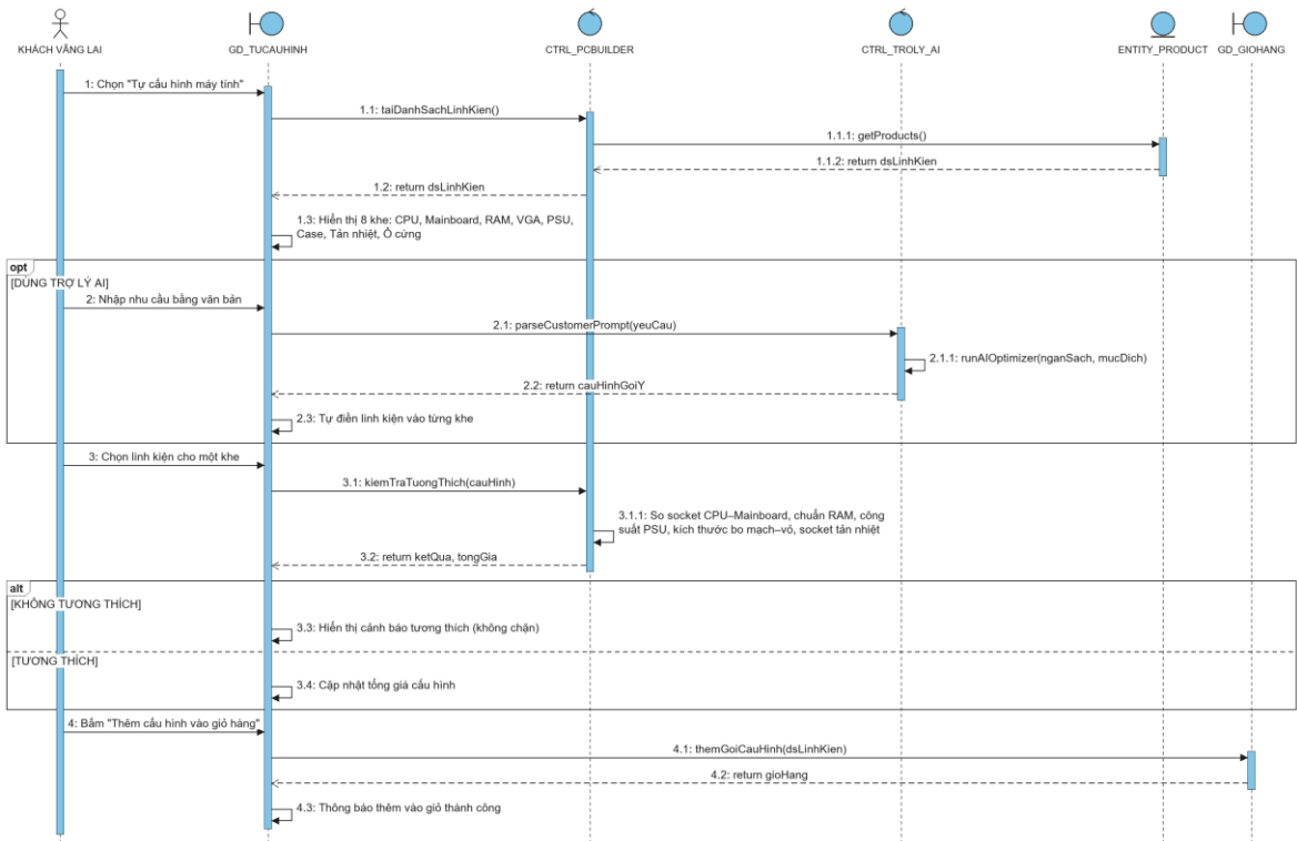
Hình 3.33 Sơ đồ tuần tự use case Tự cấu hình máy tính
