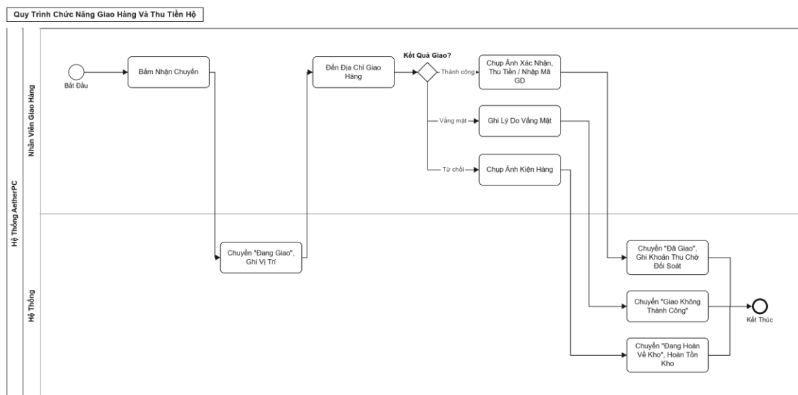
Hình 3.20 Sơ đồ BPMN quy trình chức năng giao hàng và thu tiền hệ
