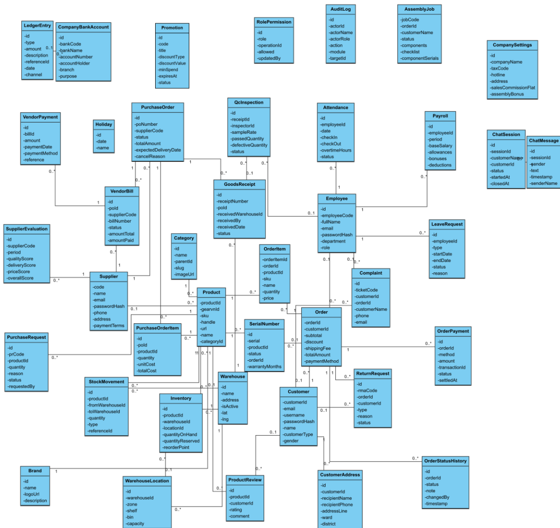
Hình 3.78 Sơ đồ Domain của hệ thống AetherPC
