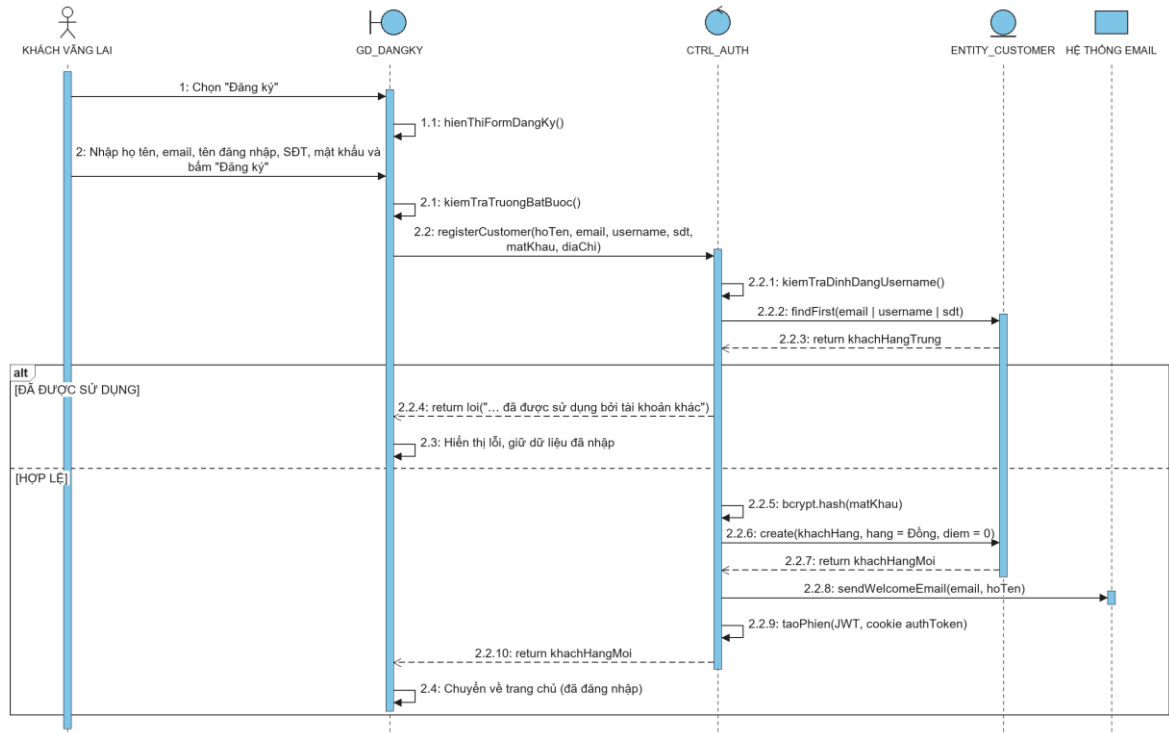
Hình 3.31 Sơ đồ tuần tự use case Đăng ký tài khoản
