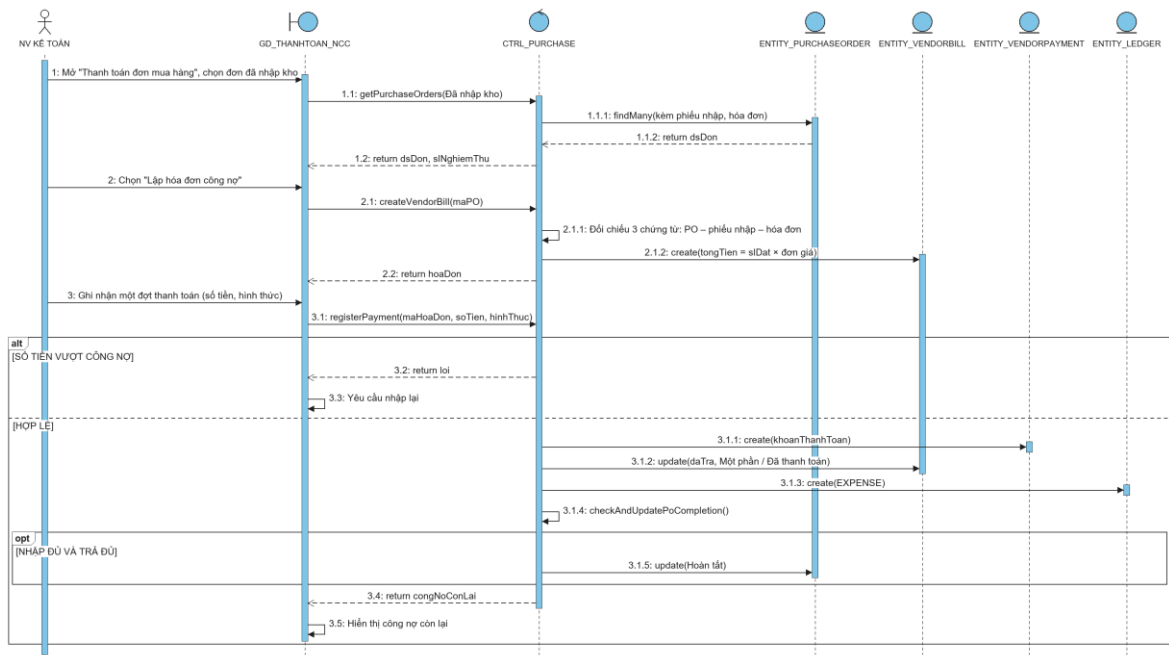
Hình 3.63 Sơ đồ tuần tự use case Thanh toán nhà cung cấp
