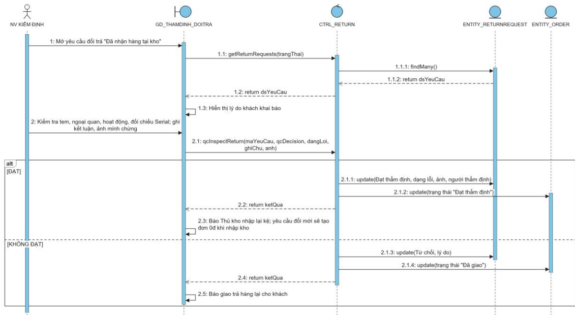
Hình 3.53 Sơ đồ tuần tự use case Thẩm định hàng hoàn trả
