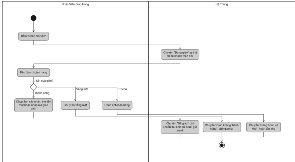
Hình 3.60 Sơ đồ hoạt động use case Giao hàng và thu tiền hộ
