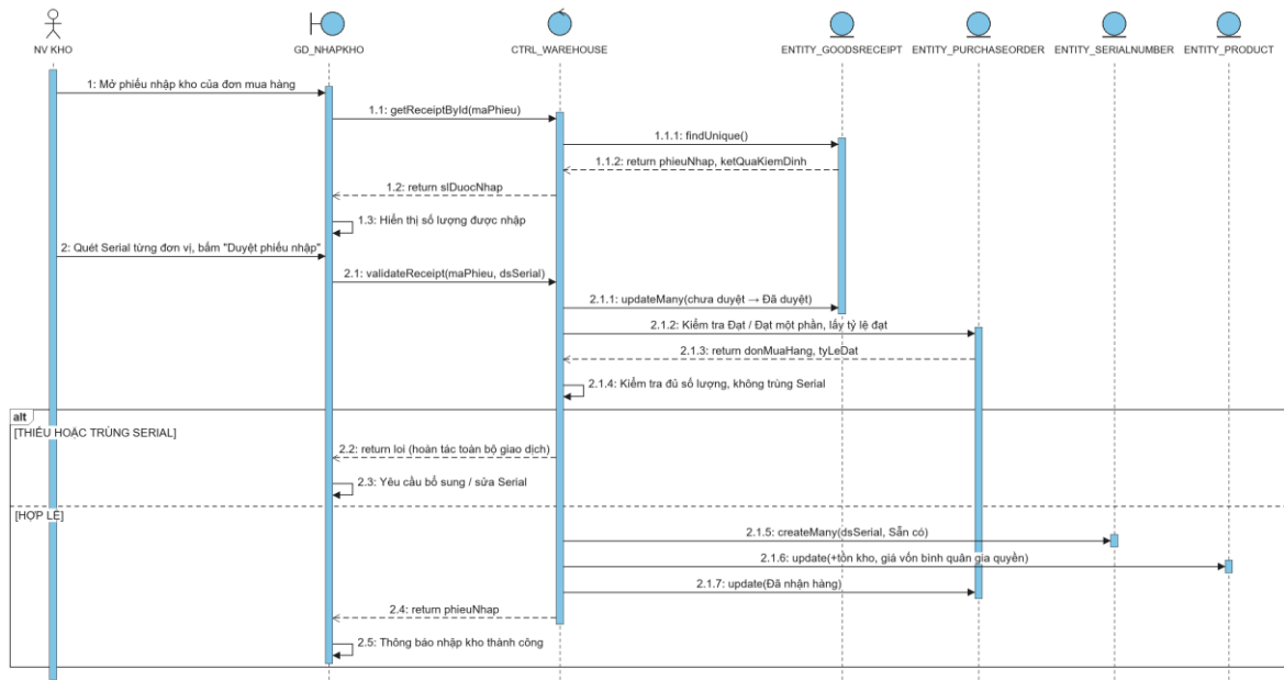
Hình 3.55 Sơ đồ tuần tự use case Nghiệm thu hàng nhập kho
