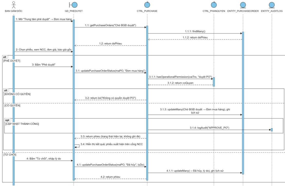
Hình 3.49 Sơ đồ tuần tự use case Duyệt đơn mua hàng
