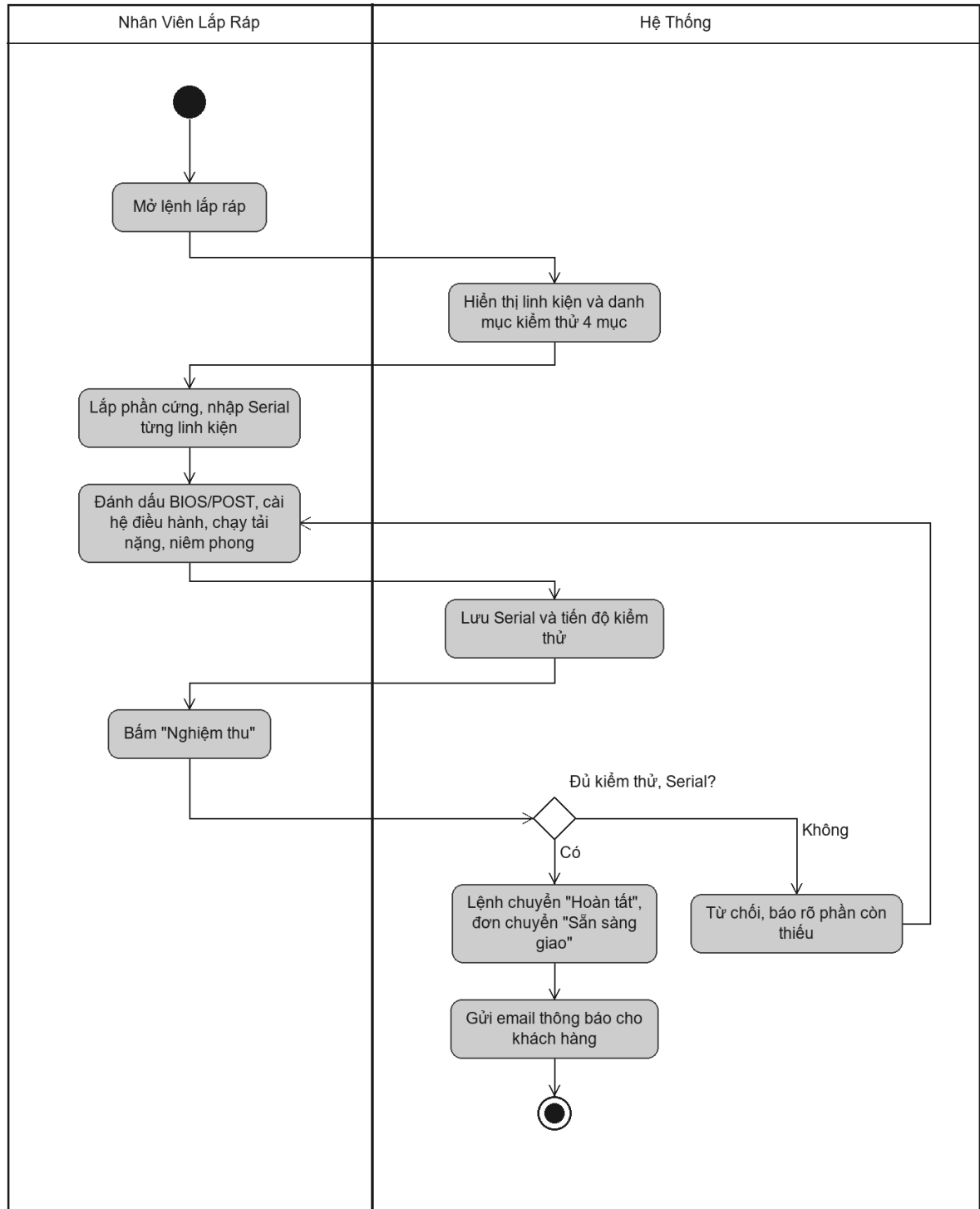
Hình 3.56 Sơ đồ hoạt động use case Cập nhật tiến độ lắp ráp
