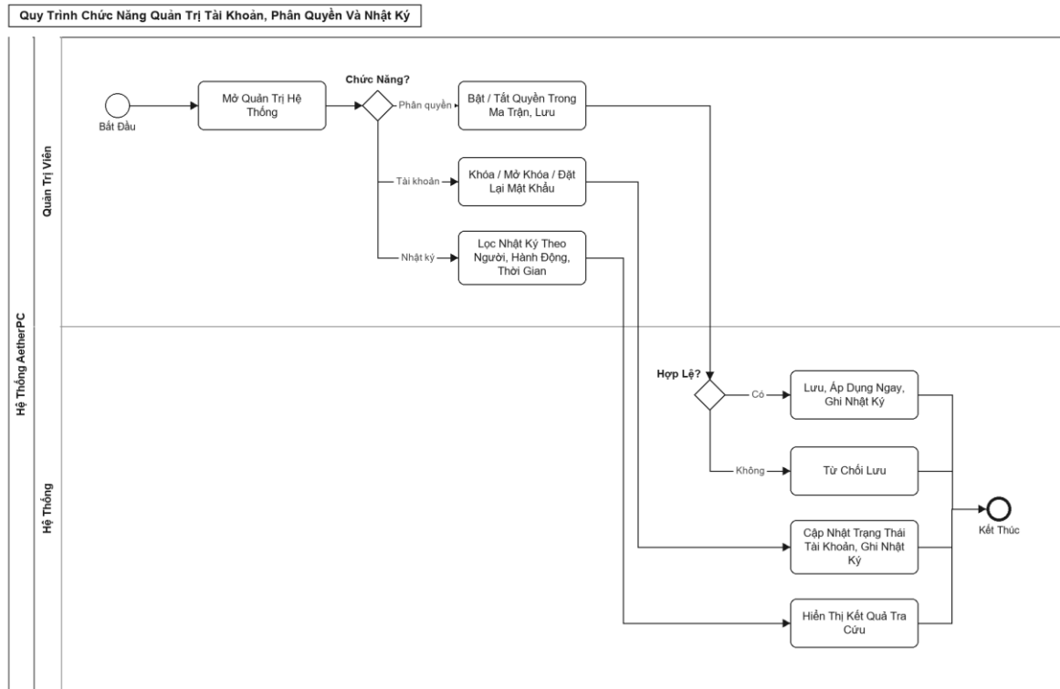
Hình 3.28 Sơ đồ BPMN quy trình chức năng quản trị tài khoản, phân quyền và nhật ký
