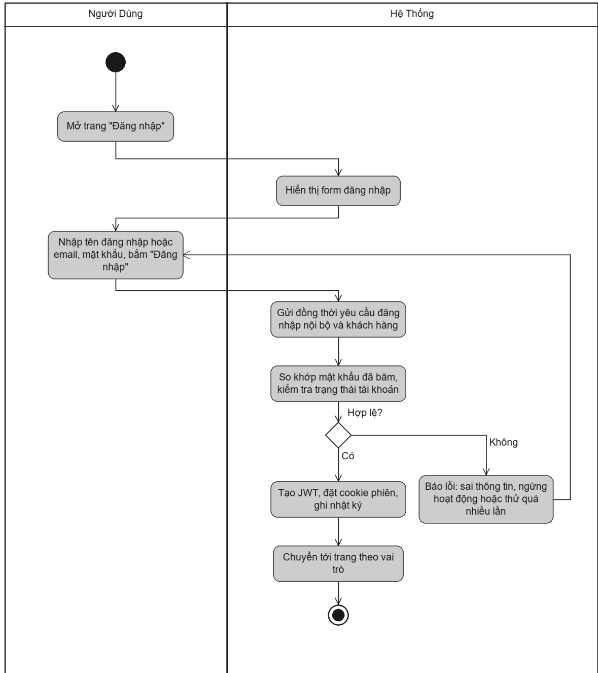
Hình 3.74 Sơ đồ hoạt động use case Đăng nhập
