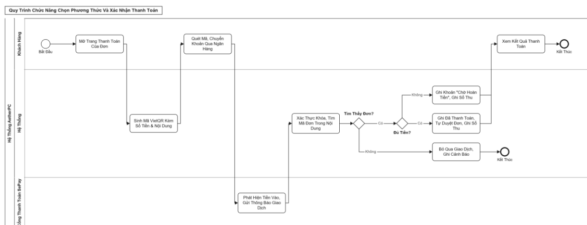
Hình 3.8 Sơ đồ BPMN quy trình chức năng chọn phương thức và xác nhận thanh toán
