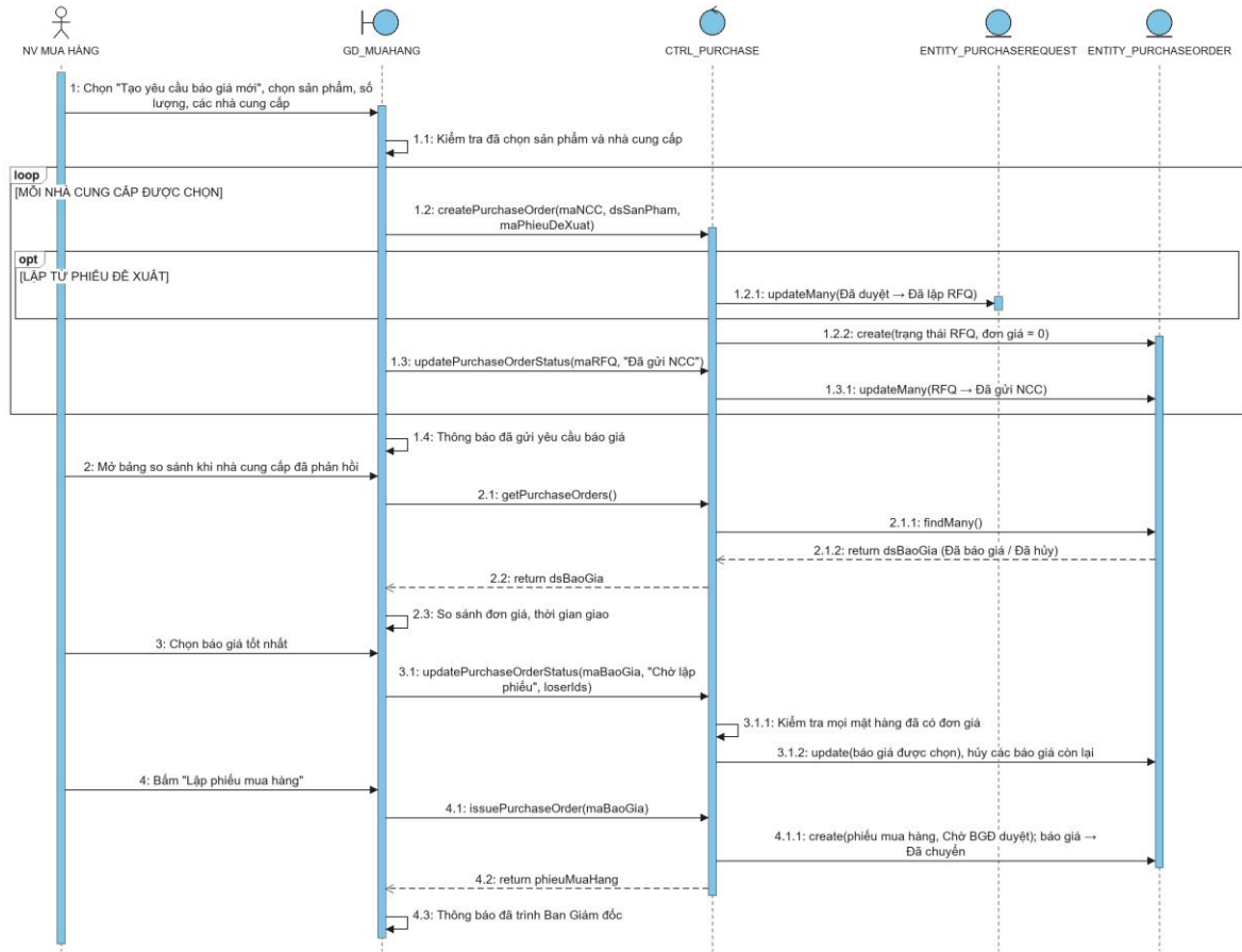
Hình 3.45 Sơ đồ tuần tự use case Lập yêu cầu báo giá và so sánh báo giá
