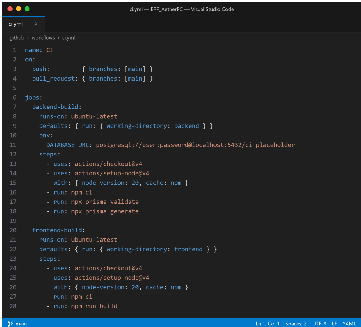
Hình 5.43 Quy trình kiểm tra biên dịch tự động bằng GitHub Actions
