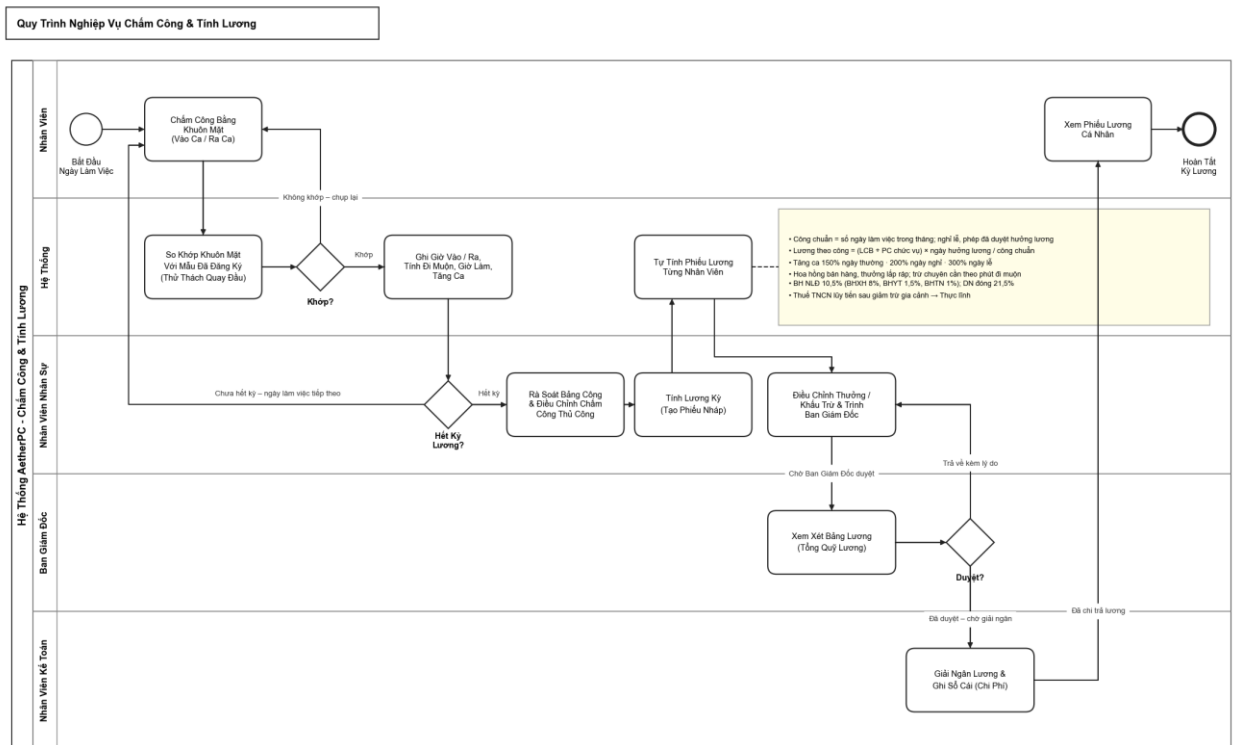
Hình 3.4 Sơ đồ BPMN quy trình chấm công và tính lương
