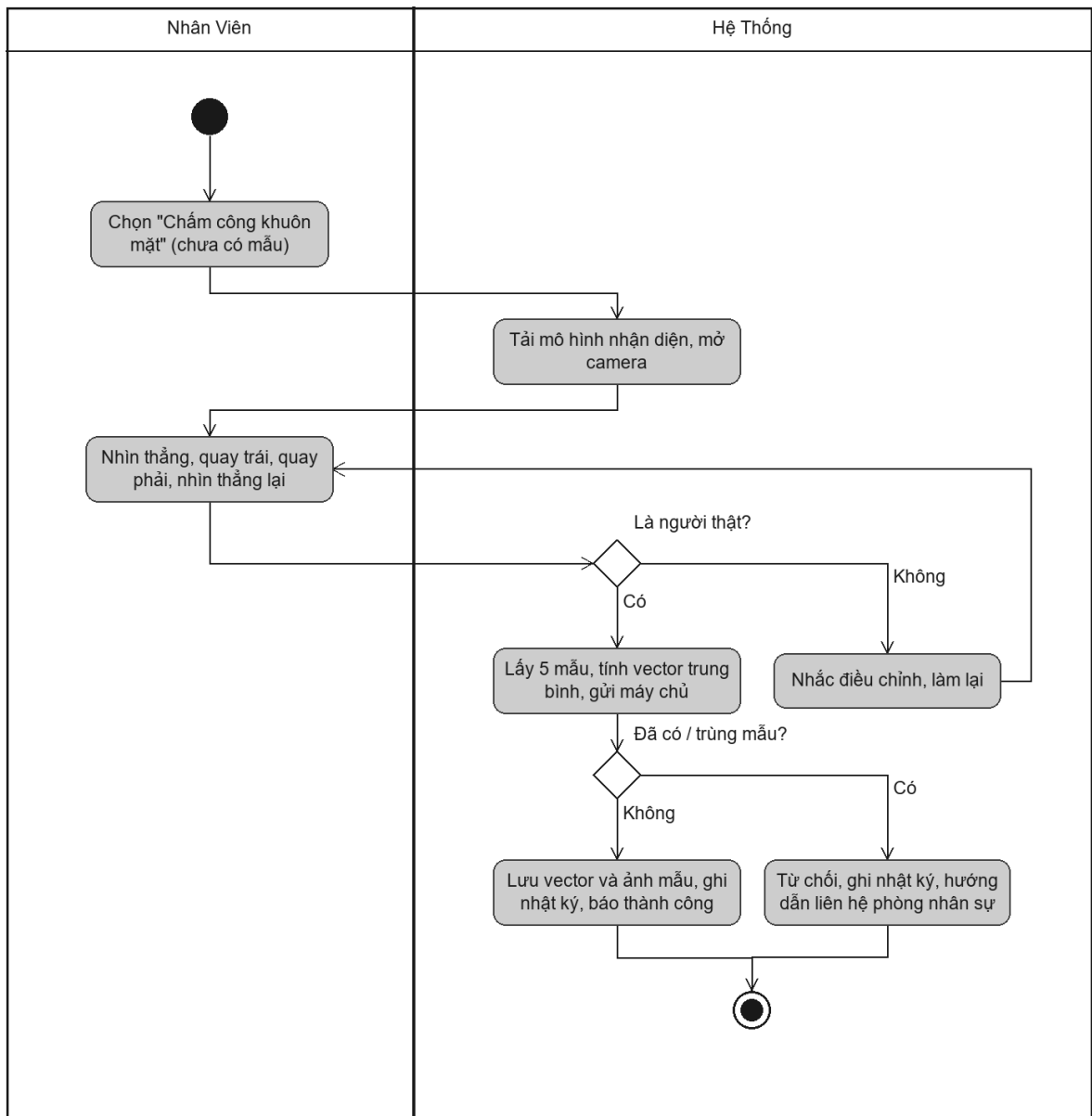
Hình 3.66 Sơ đồ hoạt động use case Đăng ký khuôn mặt
