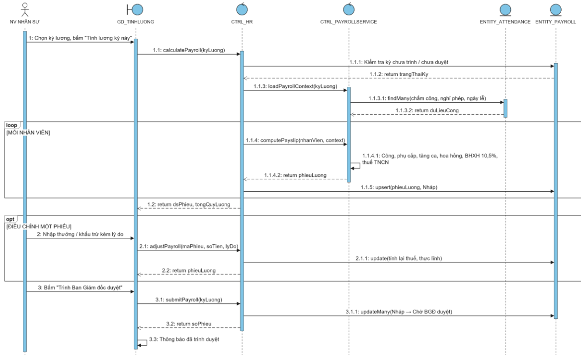
Hình 3.71 Sơ đồ tuần tự use case Tính lương và trình duyệt bảng lương
