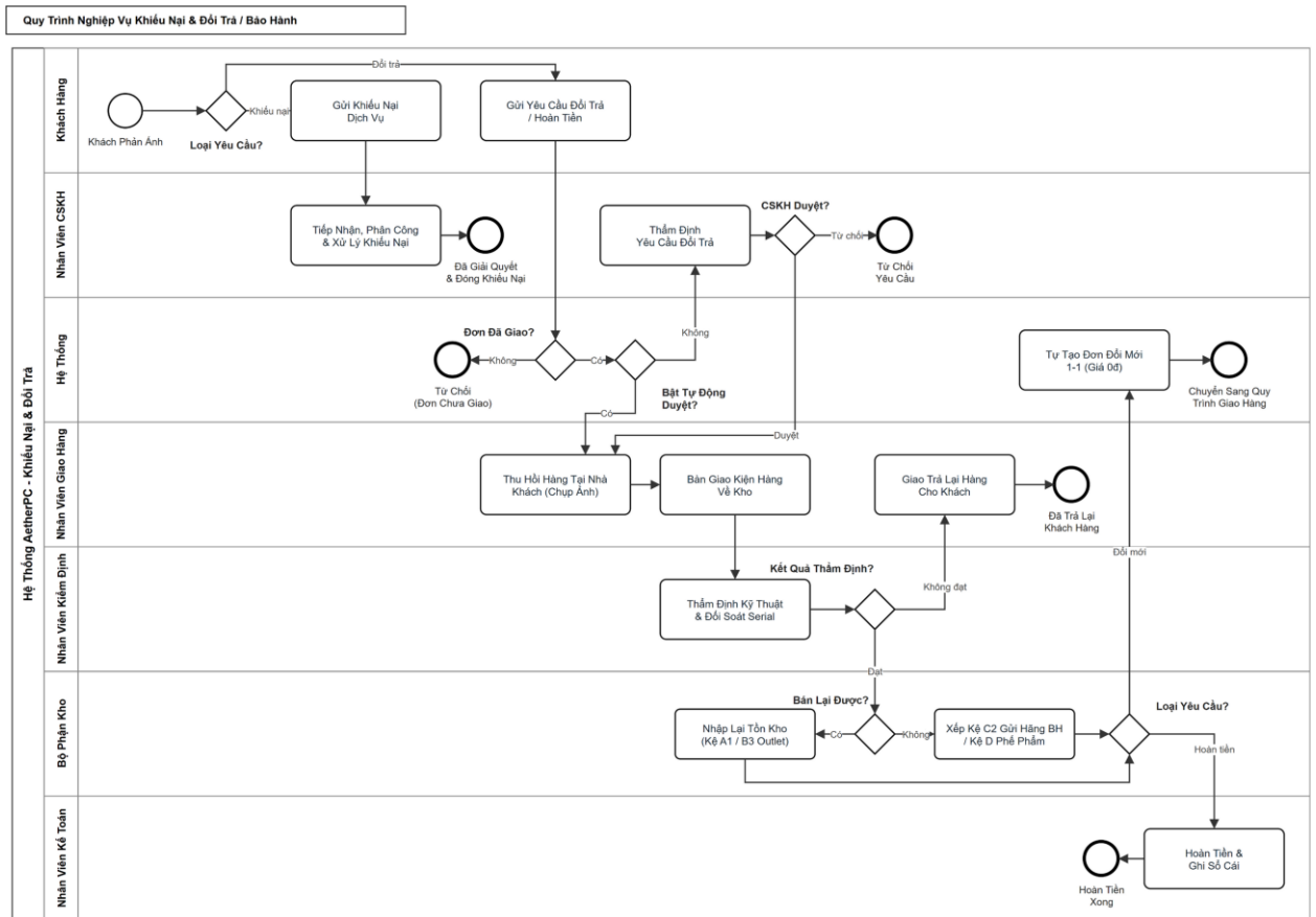
Hình 3.3 Sơ đồ BPMN quy trình khiếu nại và đổi trả – bảo hành
