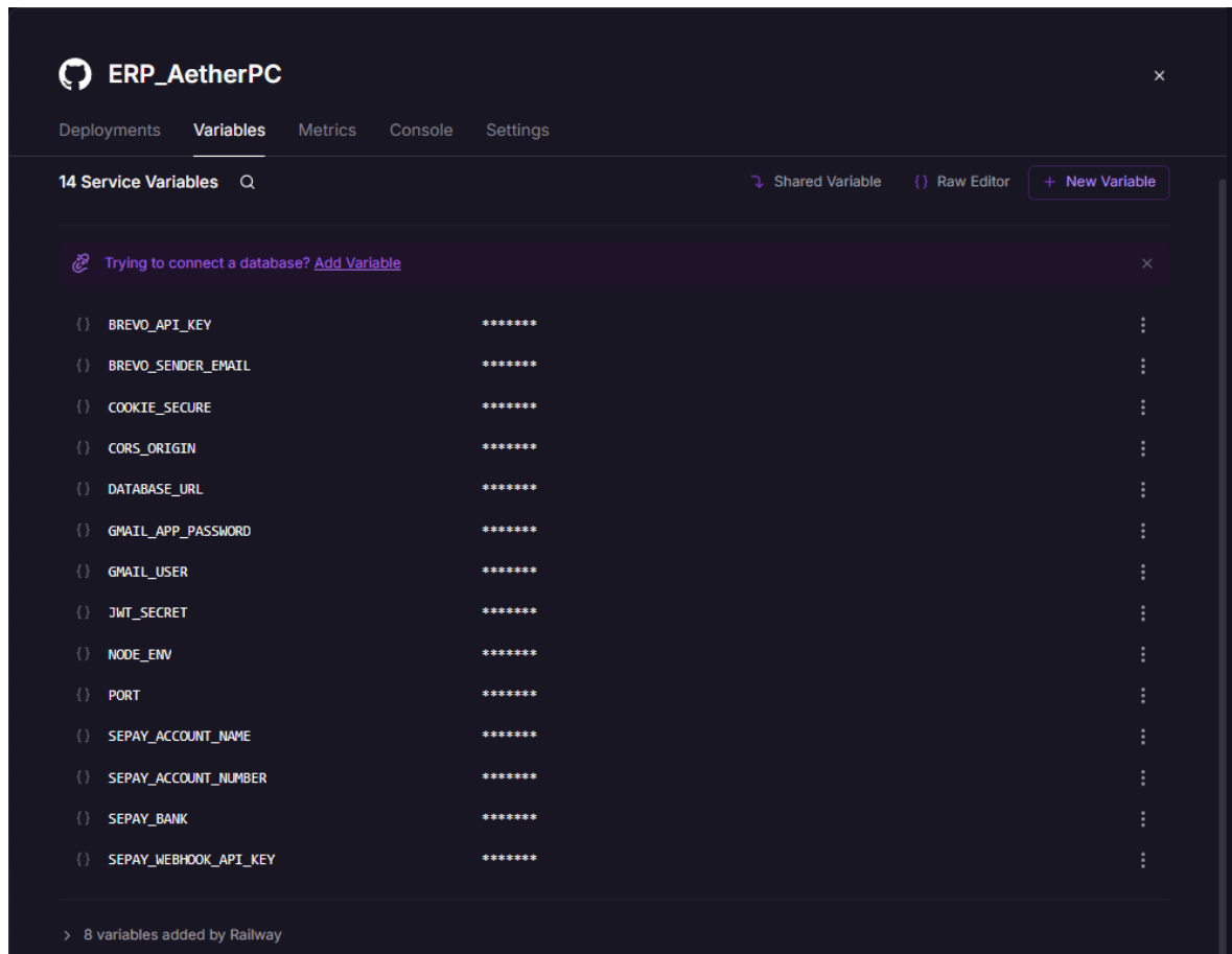
Hình 5.38 Biến môi trường của dịch vụ máy chủ ứng dụng trên Railway
