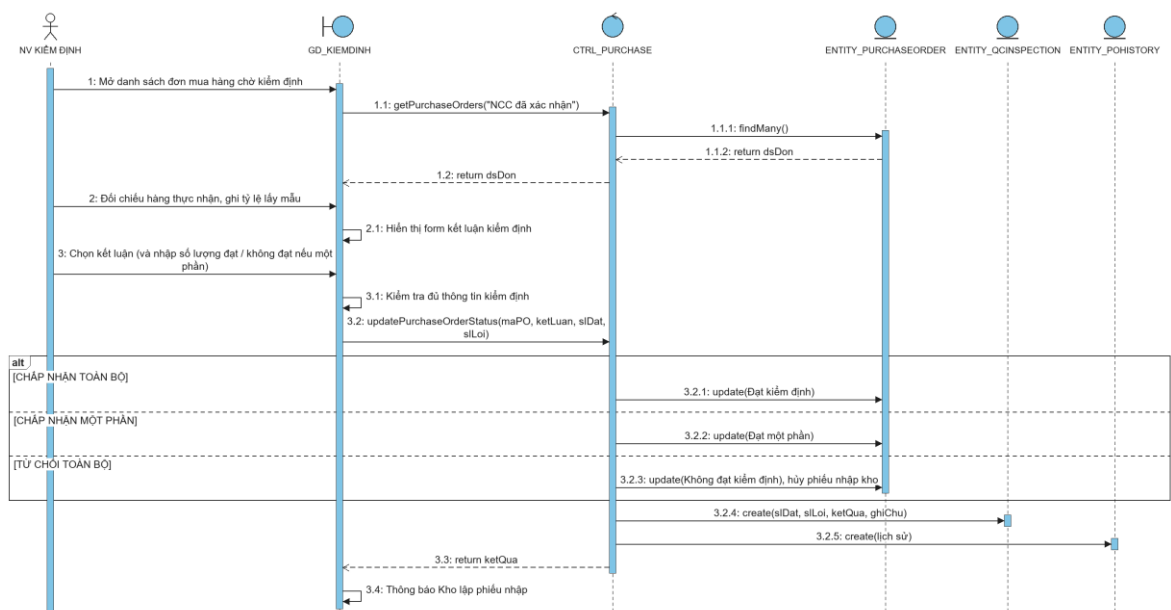
Hình 3.51 Sơ đồ tuần tự use case Kiểm tra chất lượng hàng nhập
