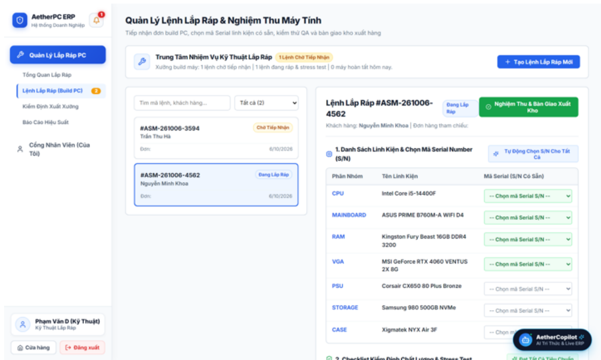
Hình 5.32 Giao diện quản lý lệnh lắp ráp
