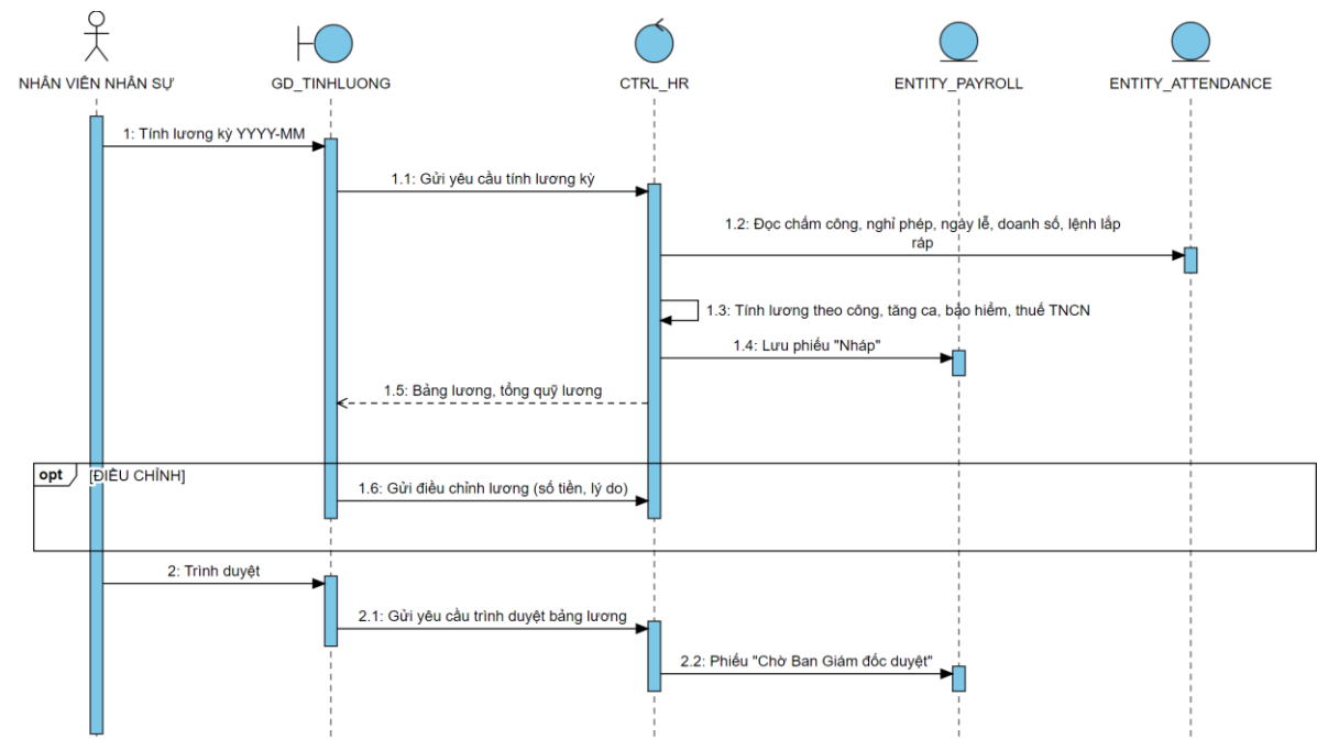
Hình 3.77 Sơ đồ tuần tự use case Tính lương và trình duyệt bảng lương
