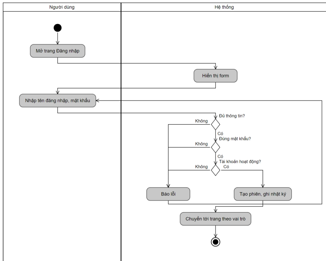
Hình 3.80 Sơ đồ hoạt động use case Đăng nhập
