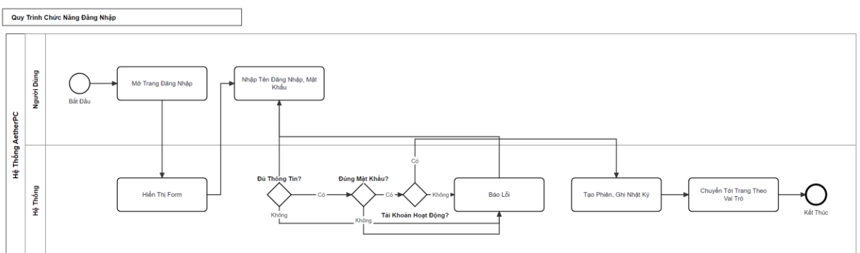
Hình 3.29 Sơ đồ BPMN quy trình chức năng đăng nhập
