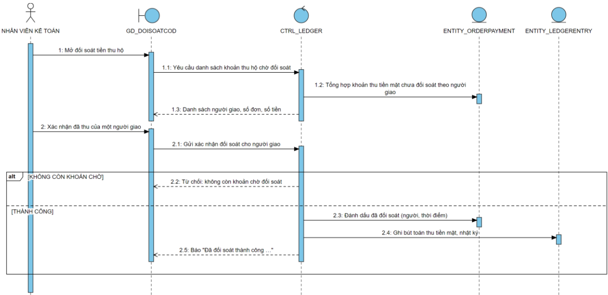
Hình 3.69 Sơ đồ tuần tự use case Đối soát tiền thu hộ
