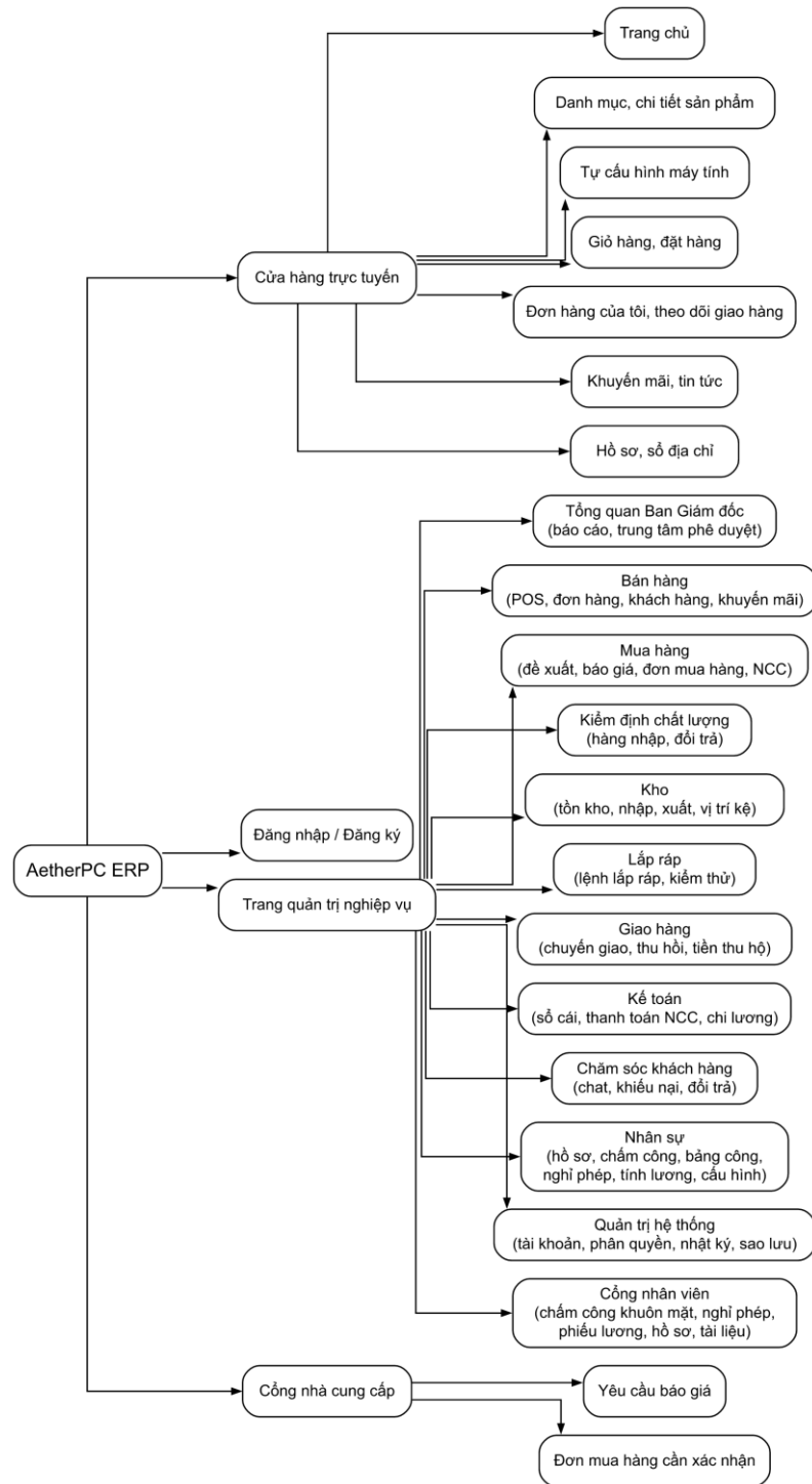
Hình 5.1 Sơ đồ site map của hệ thống AetherPC ERP
