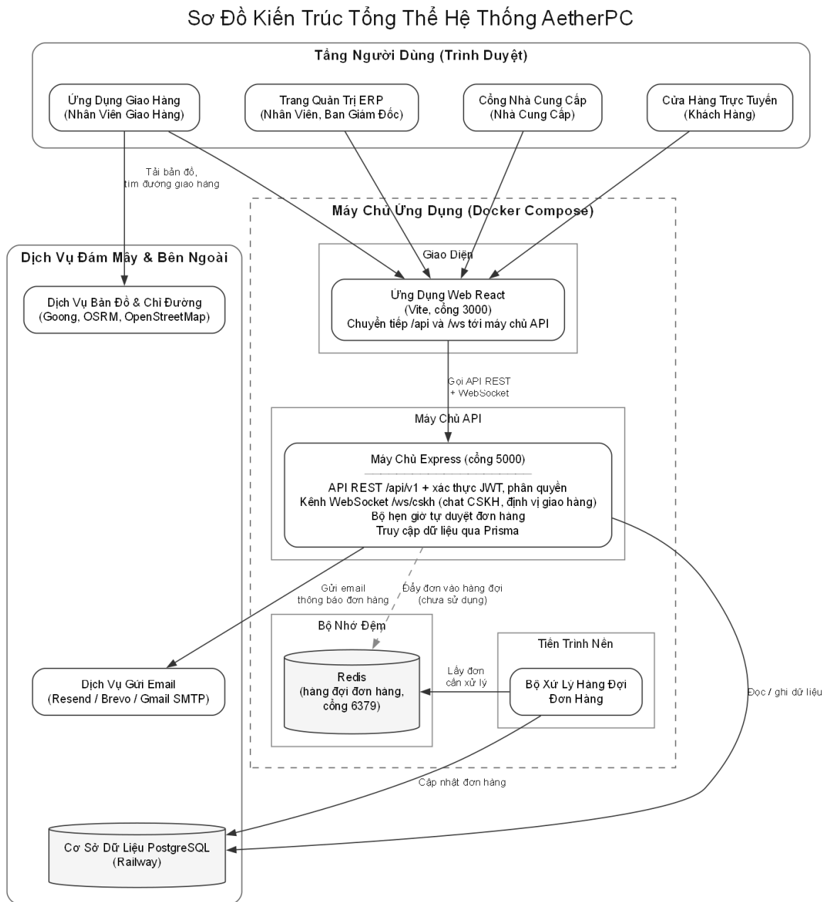
Hình 4.1 Kiến trúc tổng thể của hệ thống
