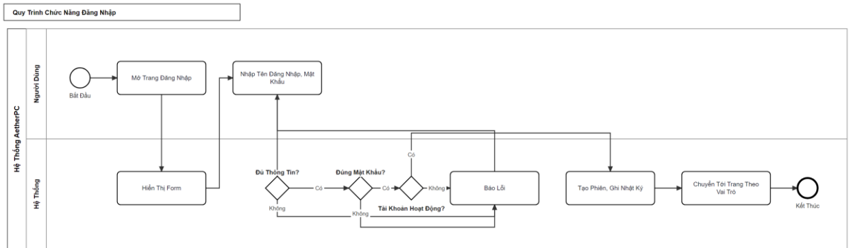
Hình 3.29 Sơ đồ BPMN quy trình chức năng đăng nhập
