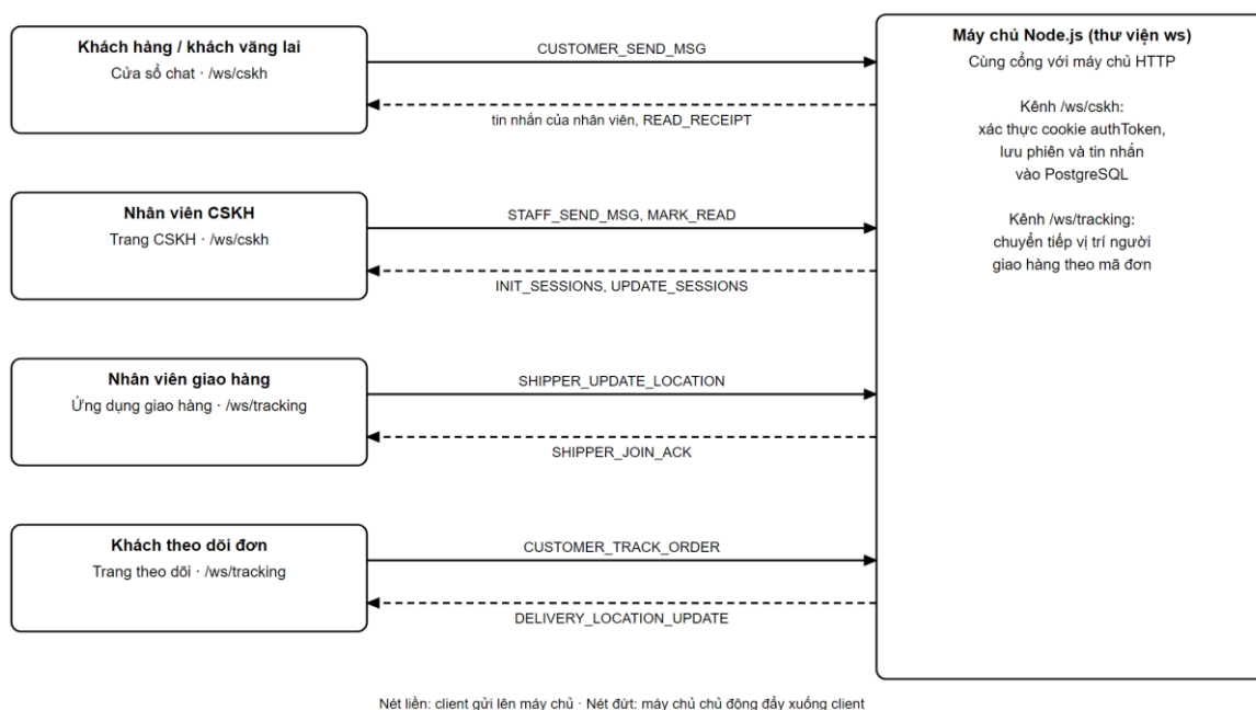
Hình 2.4 Mô hình kết nối WebSocket giữa máy chủ và các client
