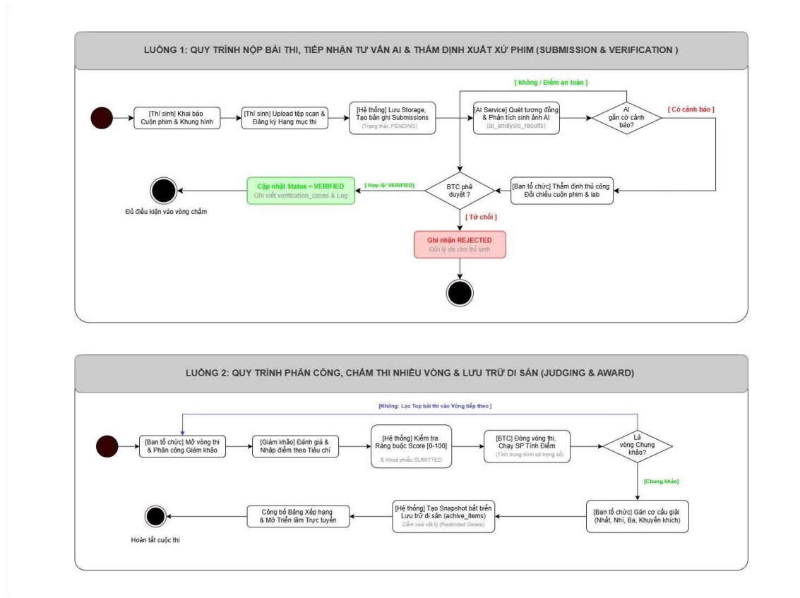
Hình 2.1. Sơ đồ Hoạt động (Activity Diagram) thể hiện 2 luồng nghiệp vụ cốt lõi của hệ thống
