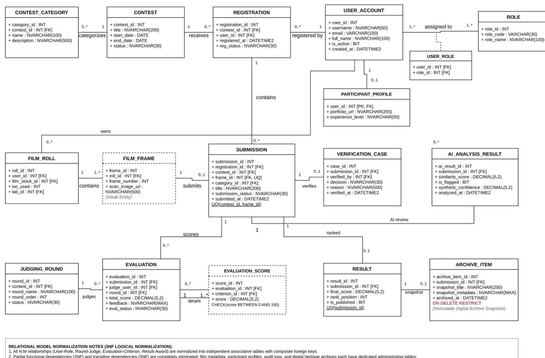
Hình 4.2. Sơ đồ Lớp / Mô hình Quan hệ Logic (Logical Schema / UML Class Diagram) đạt chuẩn 3NF
