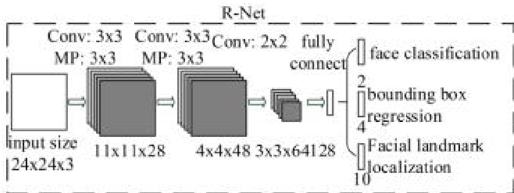
Hình 4. R-Net
