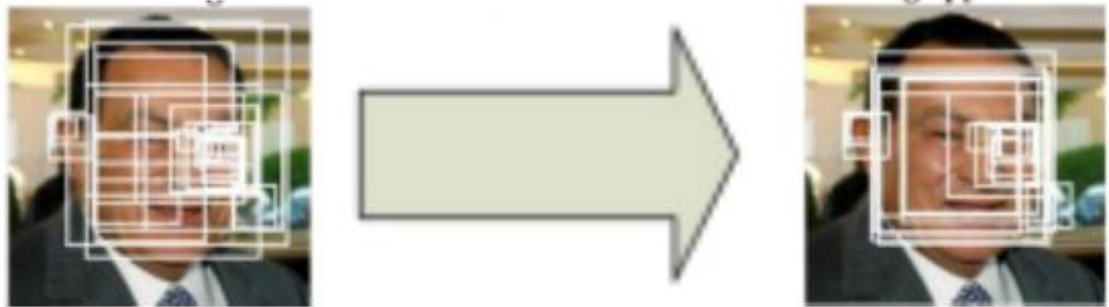
Hình 3. Picture P-Net
