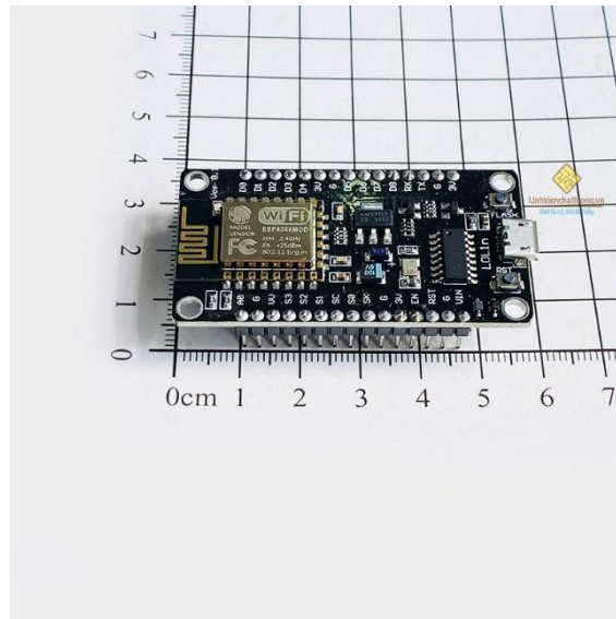
Hình 10. ESP8266 NodeMCU
