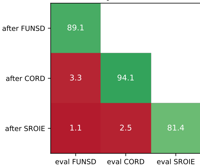
LayoutLMv3
