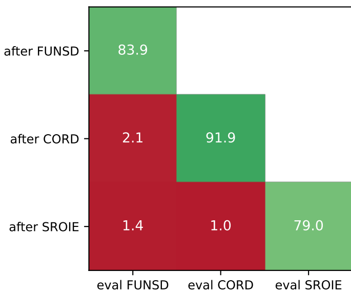
LiLT
