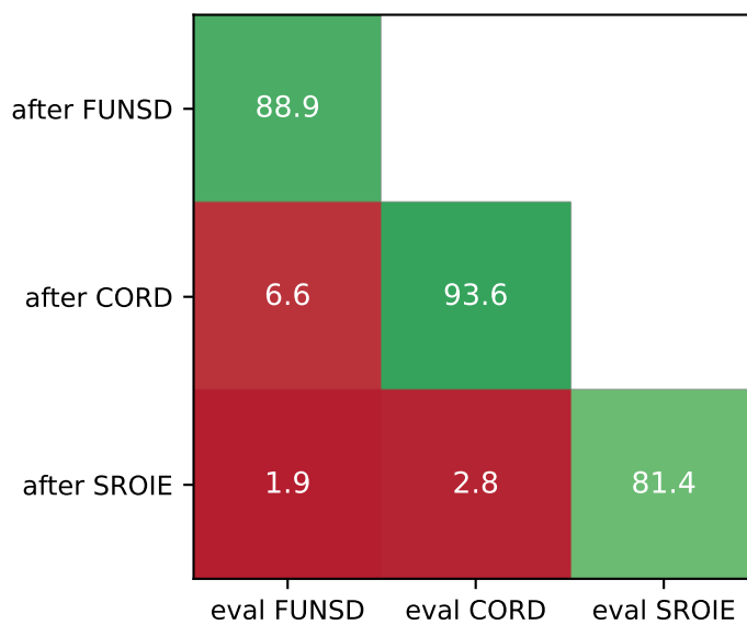
BROS
