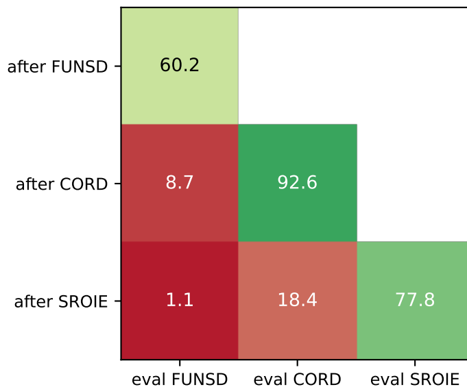
BERT
