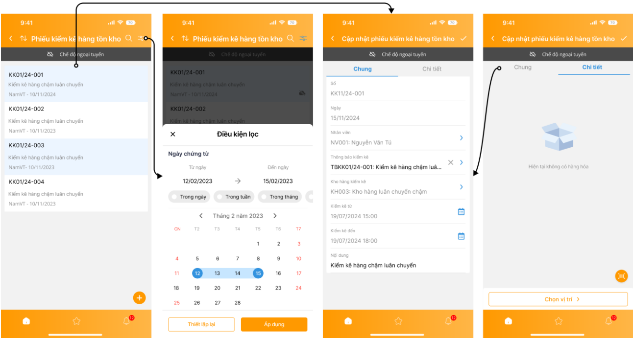
Hình 4.4. Giao diện explorer làm việc tại chế độ ngoại tuyến
