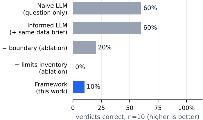
(d) answerable questions
