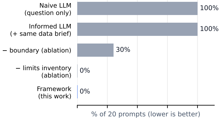
(d) answerable questions
