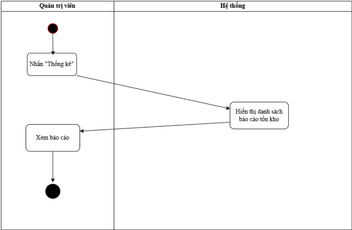
USE CASE: XEM BÁO CÁO THỐNG KÊ
