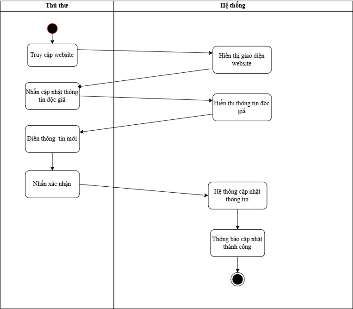
USE CASE: CẬP NHẬT THÔNG TIN ĐỘC GIẢ
