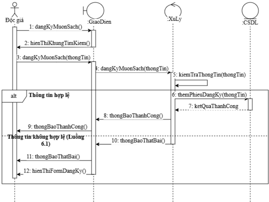
Use Case: Đăng ký mượn sách
