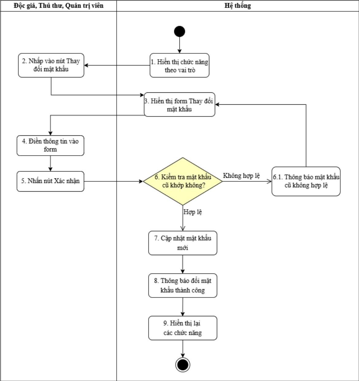
Use case: Thay đổi mật khẩu
