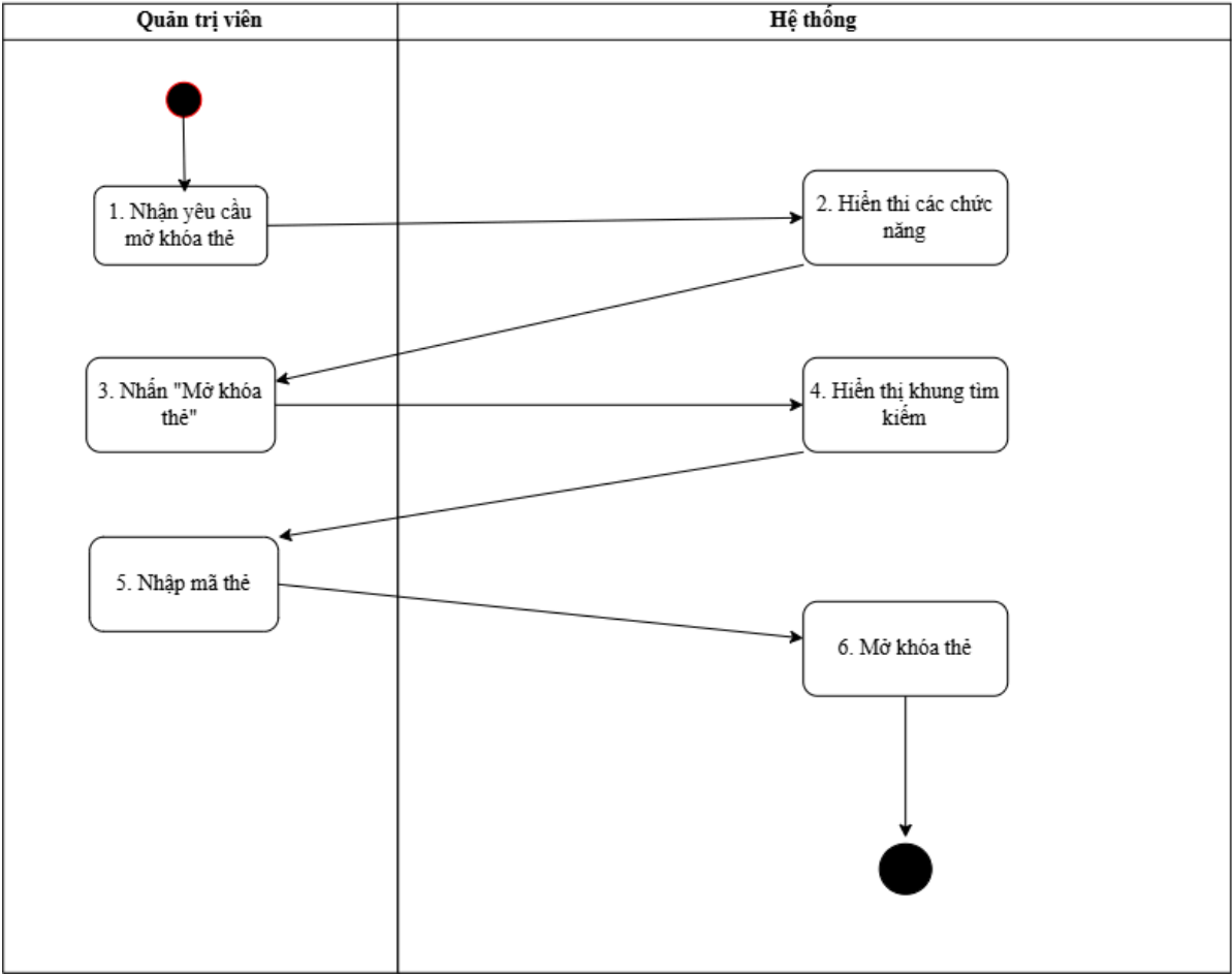
USE CASE: MỞ KHÓA THẺ
