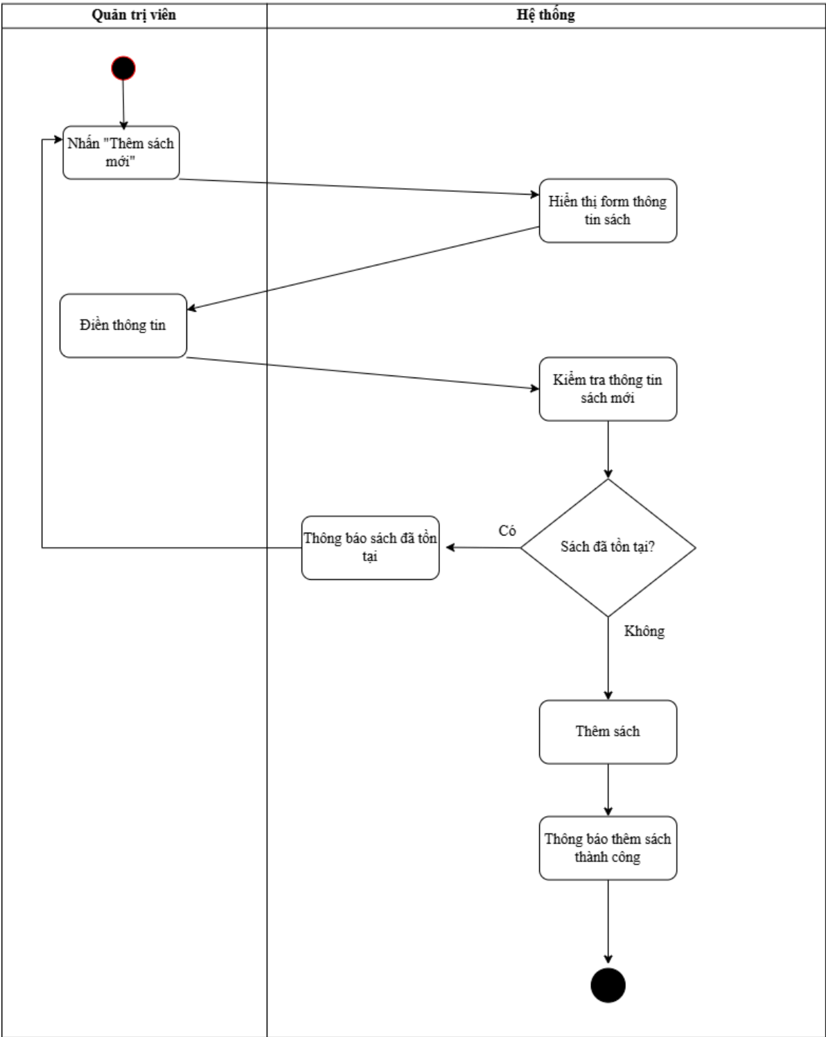
USE CASE: THÊM SÁCH MỚI
