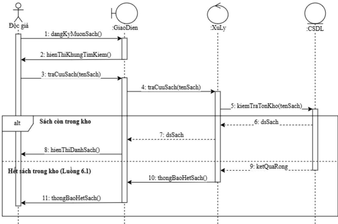
Use case: Tra cứu thông tin sách
