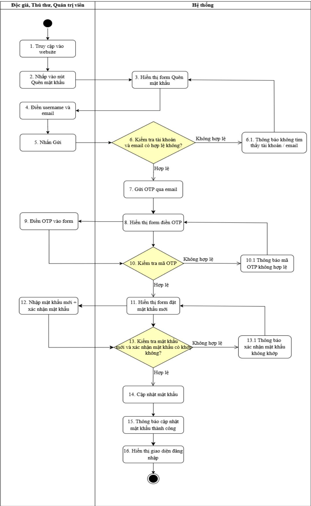
Use case: Quên mật khẩu
