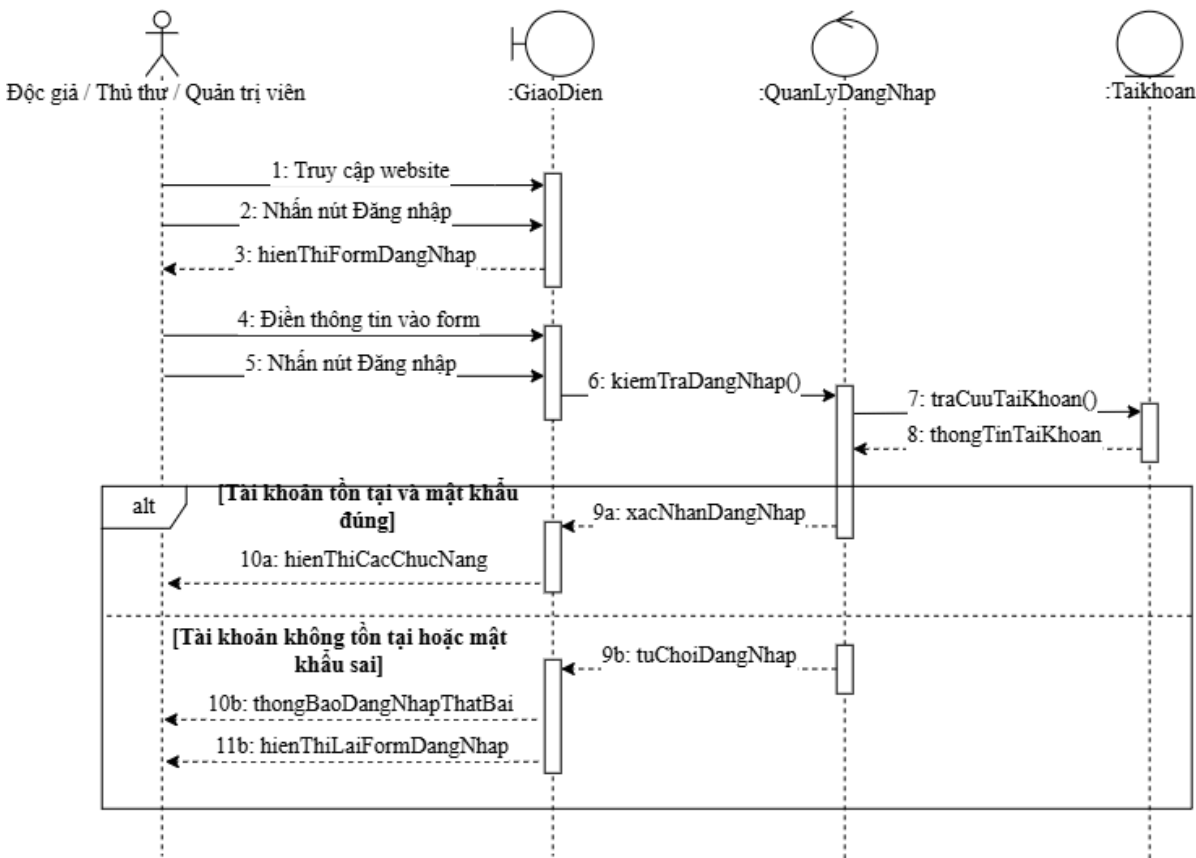
Use case: Đăng nhập
