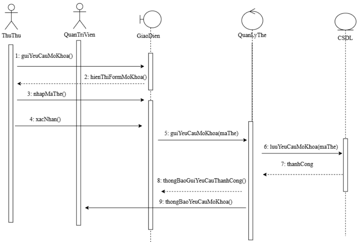
USE CASE:YÊU CẦU MỞ KHÓA THẺ
