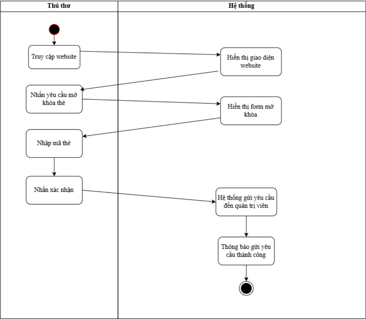
USE CASE: YÊU CẦU MỞ KHÓA THẺ
