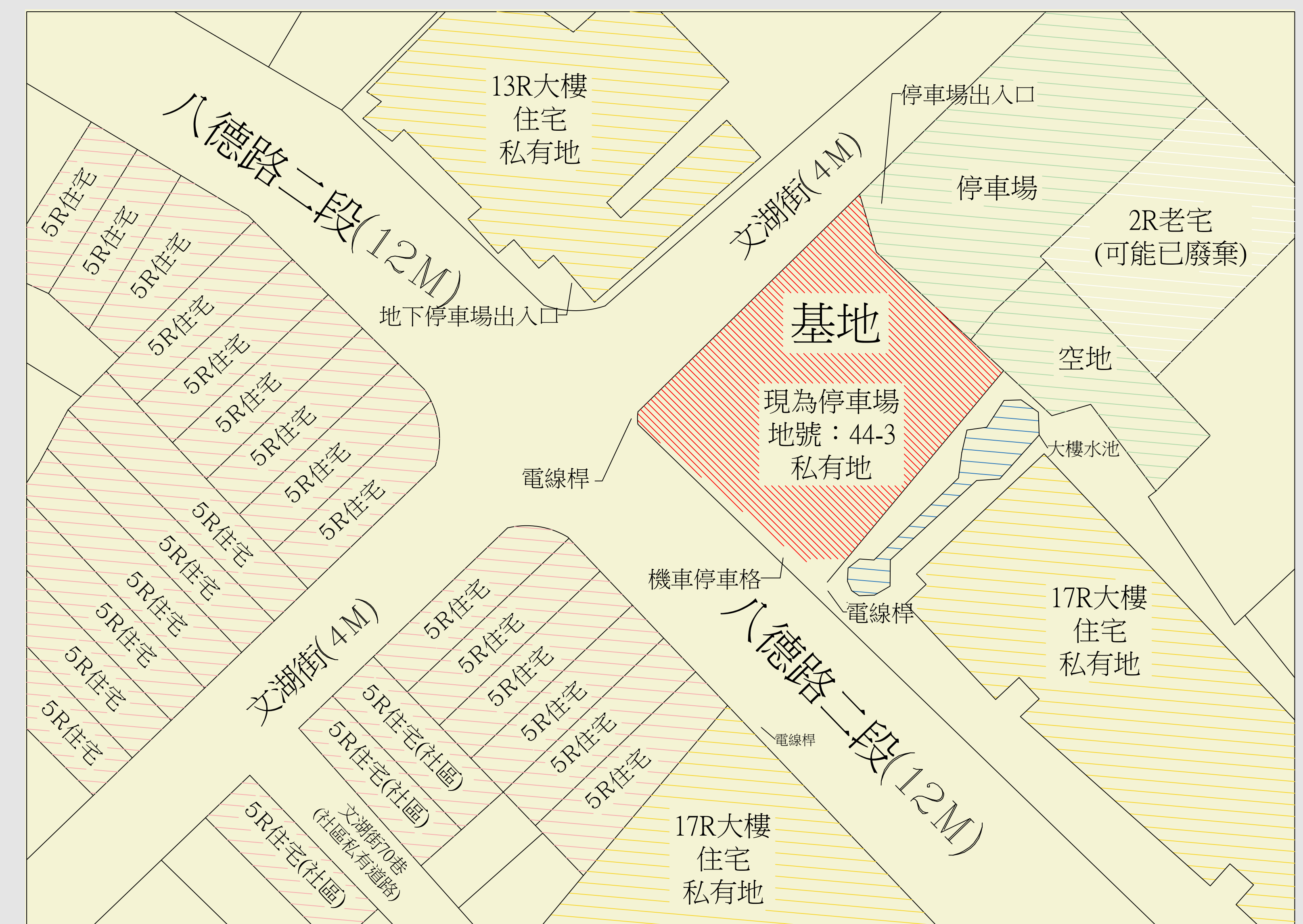
基地配置圖 比例：1/1000
