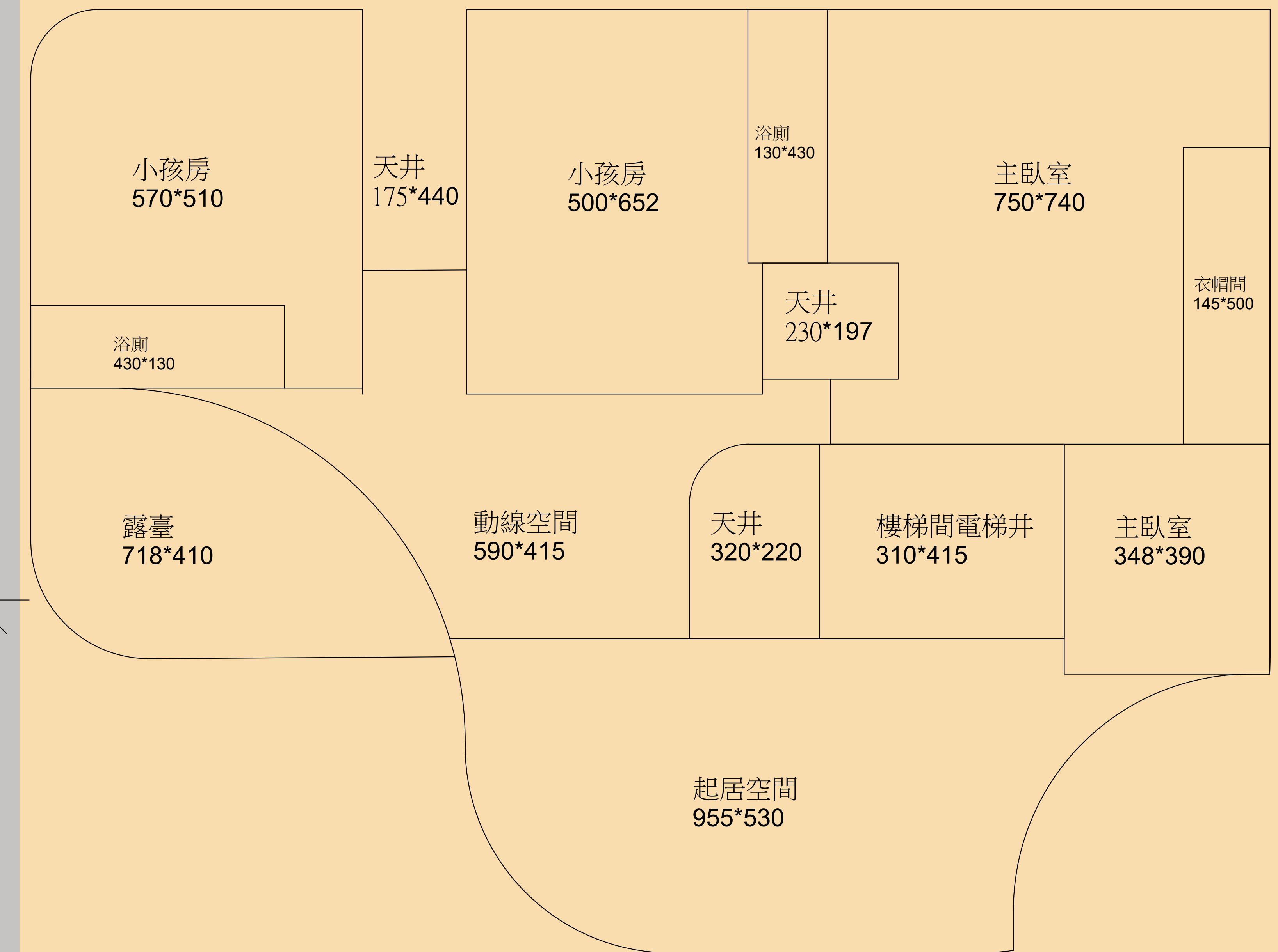
三層空間定量圖
