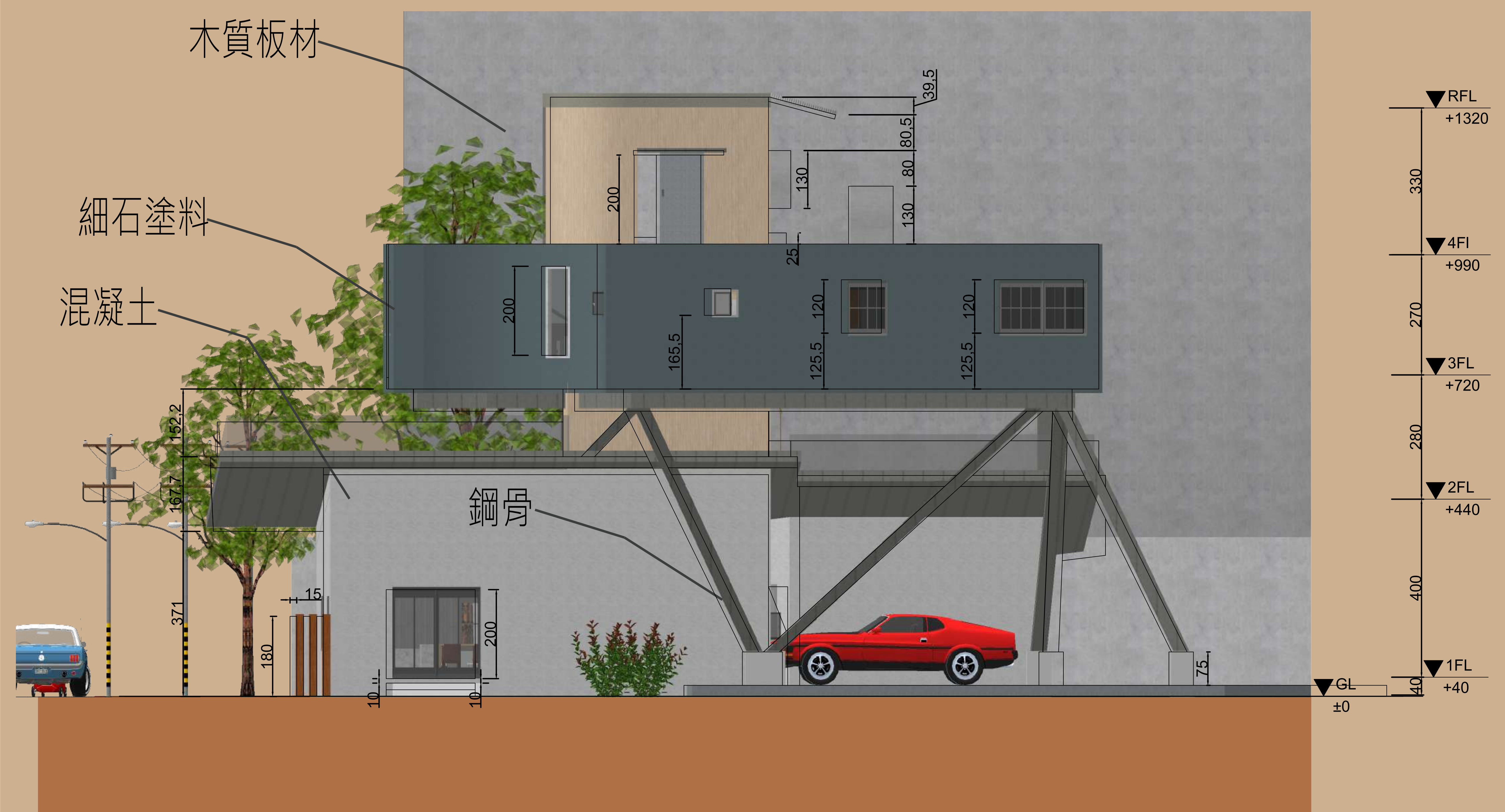
西向立面圖 比例：1/50
