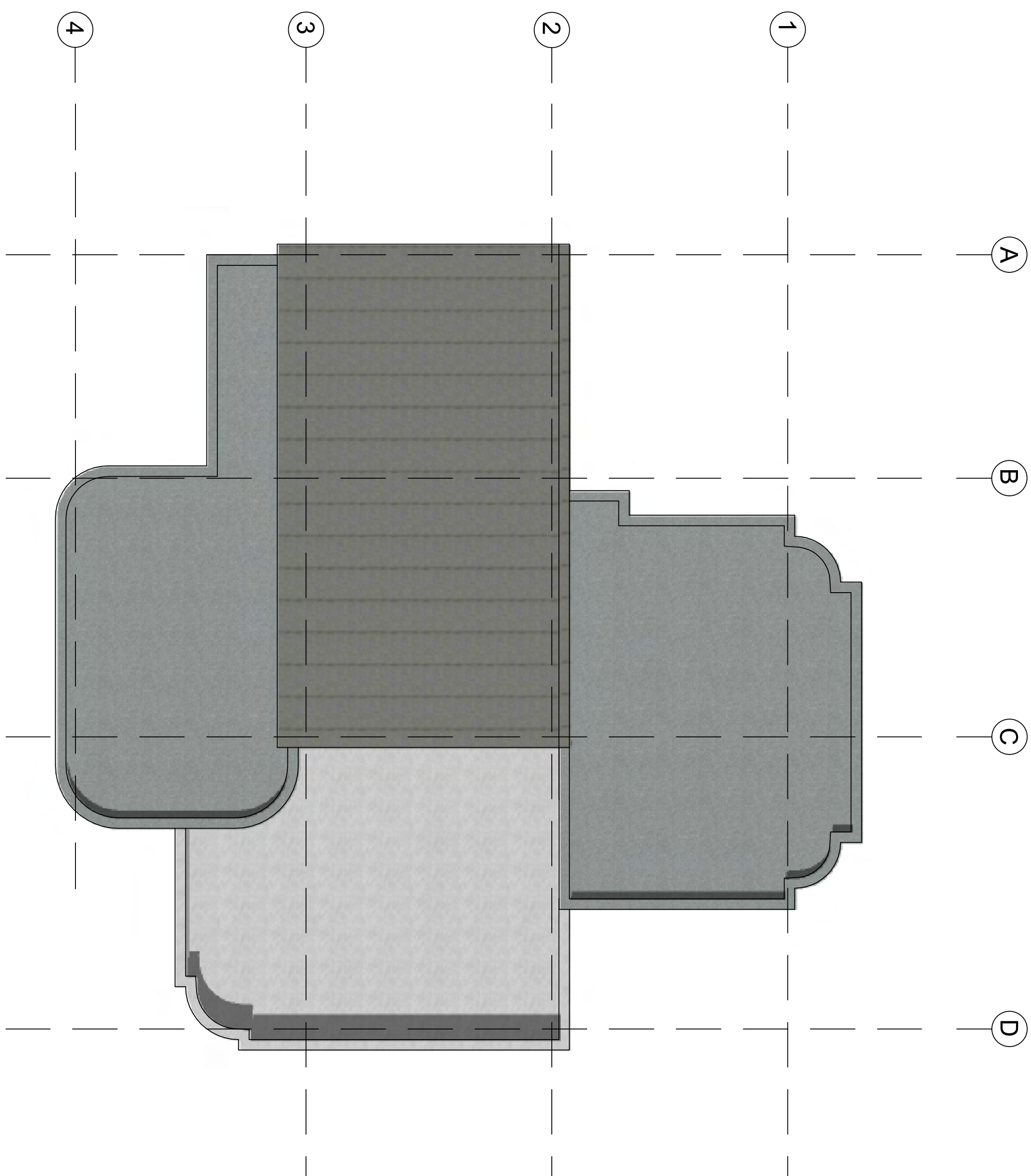
屋頂層平面圖 比例：1/50
