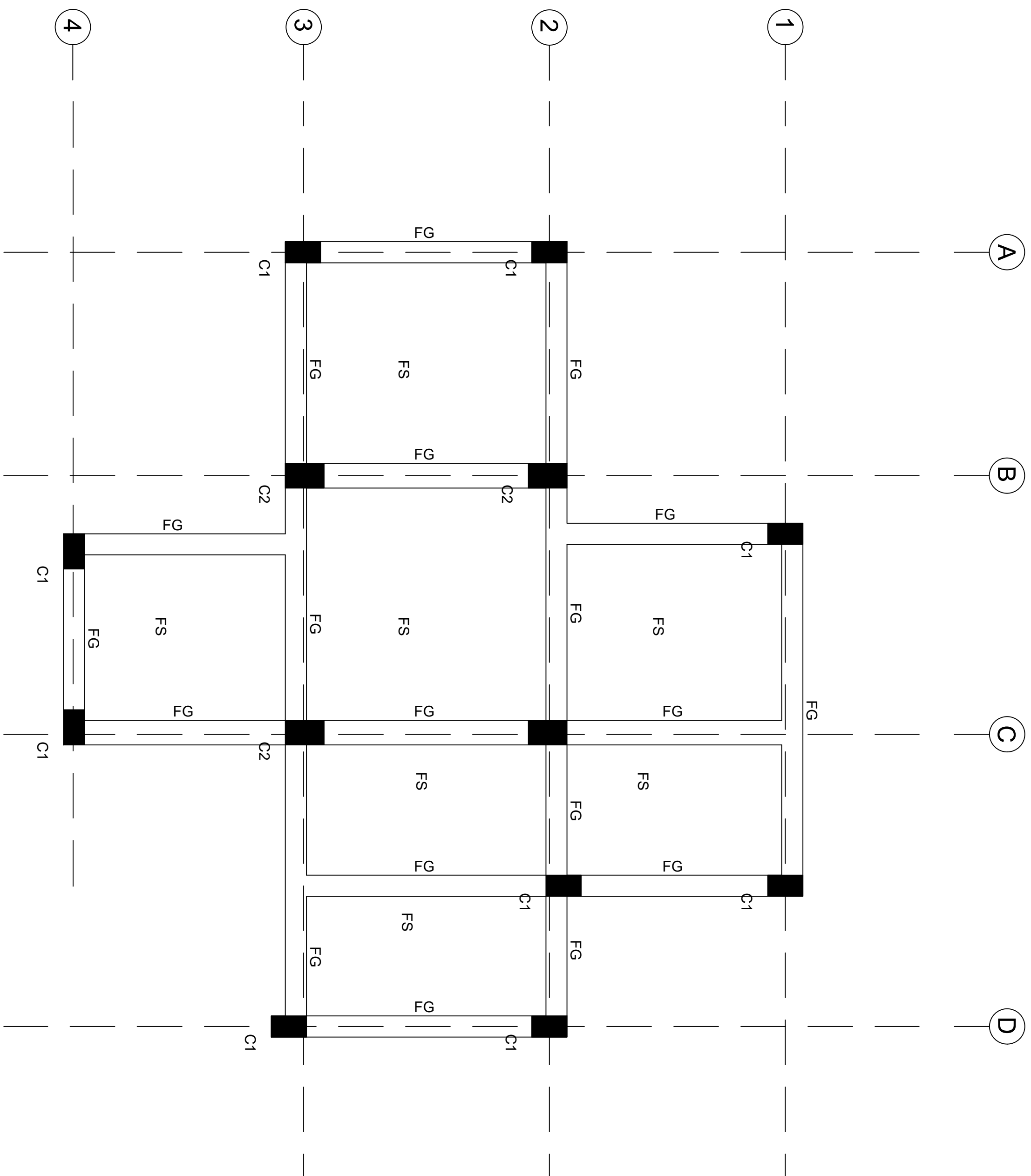
基礎平面圖 比例：1/50
