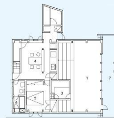
1F Plan 1/200
