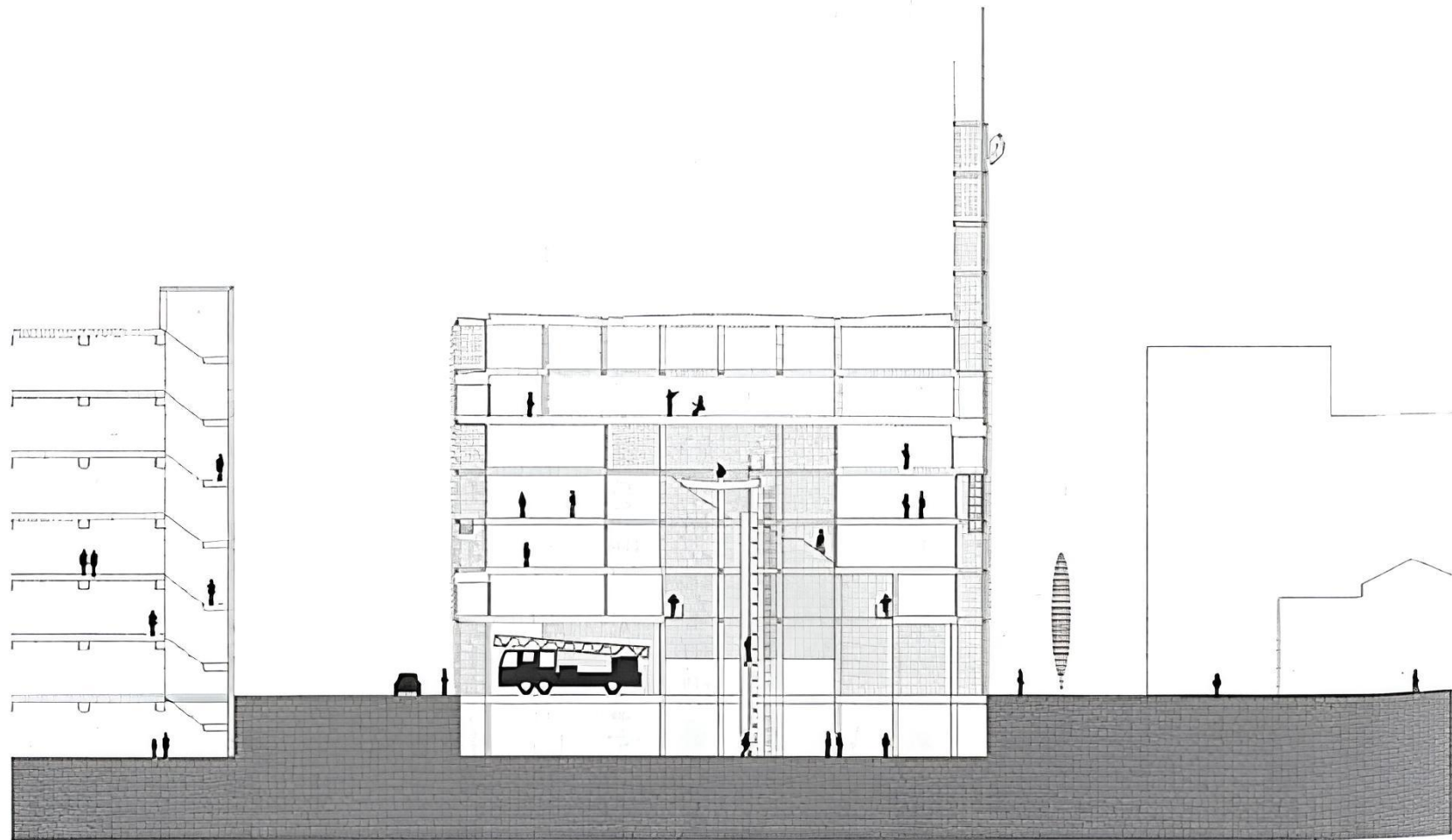
断面 縮尺1/800
