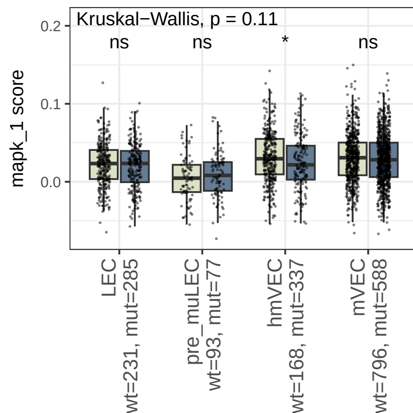
mapk_1, RAW PVALUE
