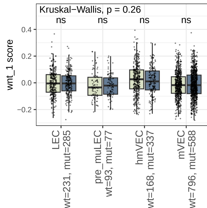
wnt_1, RAW PVALUE
