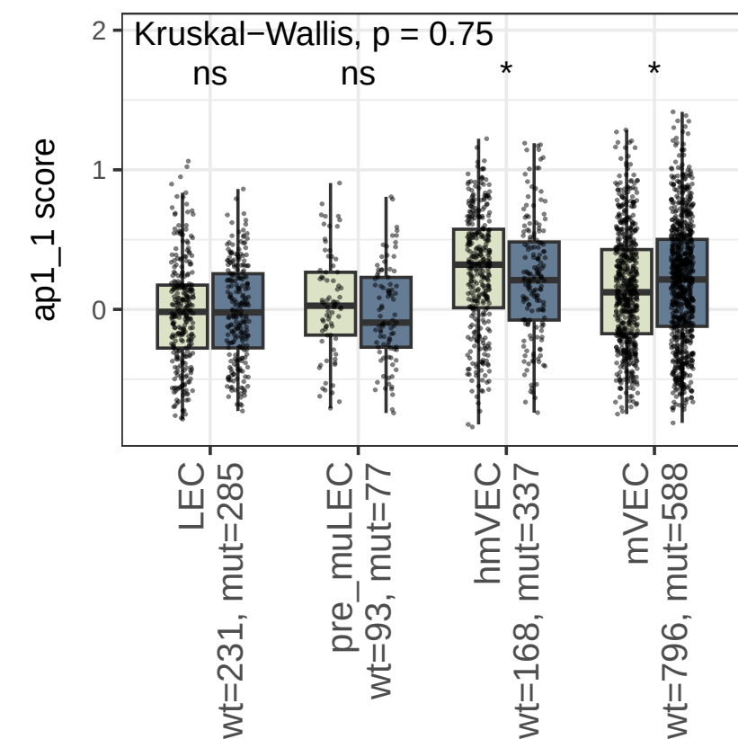
ap1_1, RAW PVALUE
