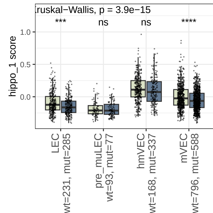
hippo_1, RAW PVALUE
