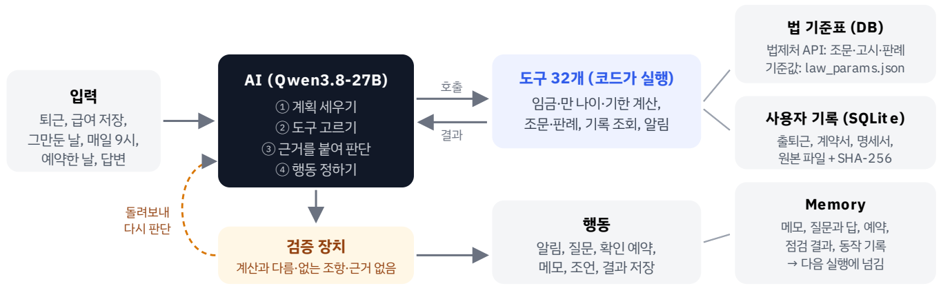
그림 1. 알바지킴이 에이전트 구조. 판단 반복은 최대 30회이고, 매 단계를 화면과 동작 기록에 남깁니다.
